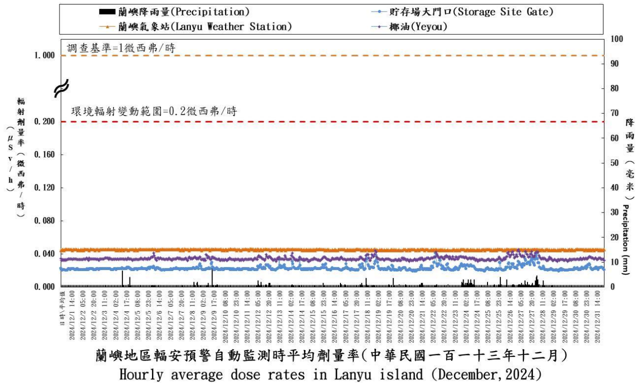
圖 6 蘭嶼地區輻安預警自動監測劑量率時變動圖
