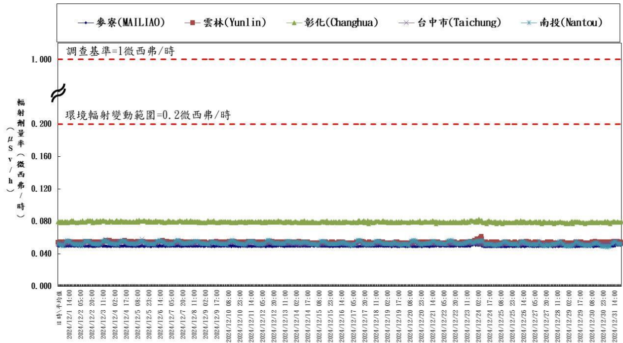
台灣中區輻安預警自動監測時平均劑量率(中華民國一百一十三年十二月) Hourly average dose rates in cities in central Taiwan (December, 2024)
