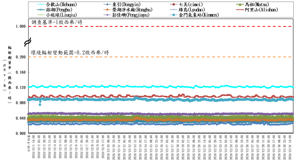
台灣外島與高山地區輻安預警自動監測時平均劑量率(中華民國一百一十三年十二月) Hourly average dose rates in mountain and islands in Taiwan (December, 2024)
