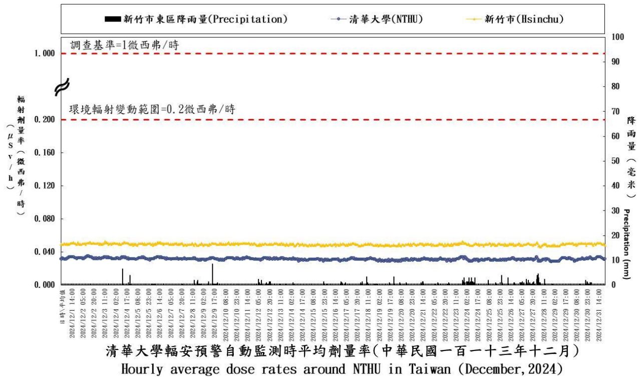
圖 5 清華大學周圍輻安預警自動監測劑量率時變動圖
