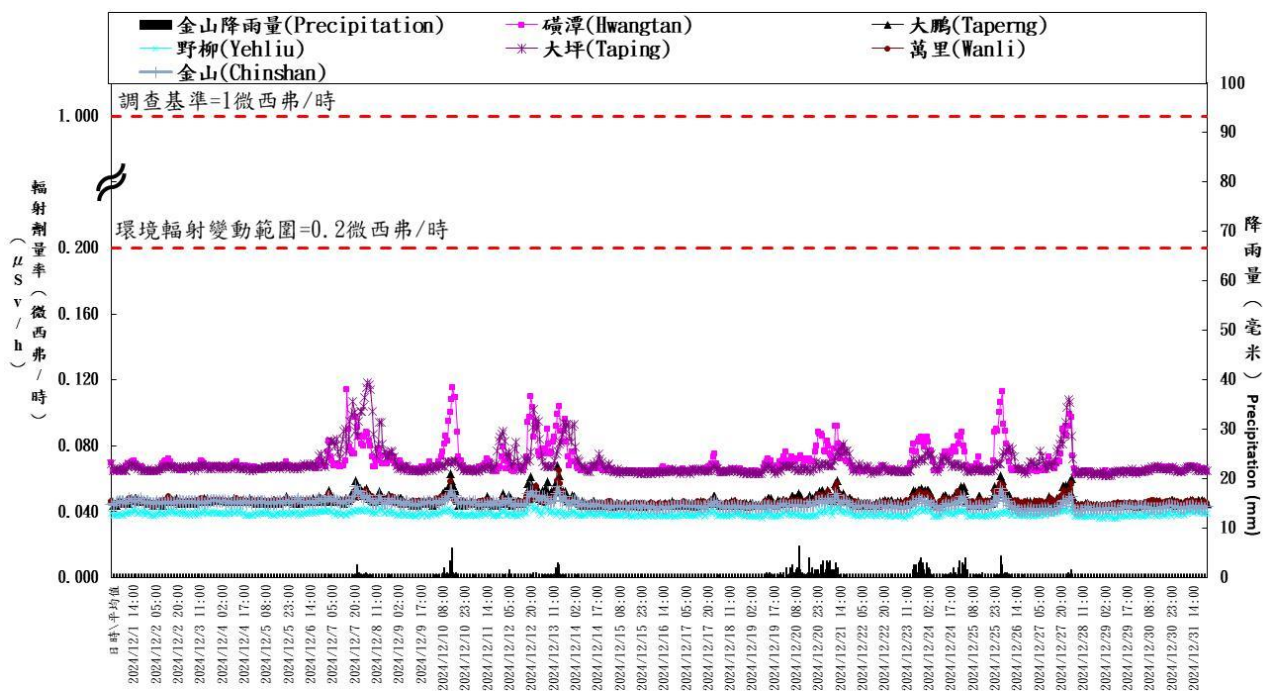
核二廠輻安預警自動監測時平均劑量率(中華民國一百一十三年十二月) Hourly average dose rates around NPP2 in Taiwan (December, 2024)
