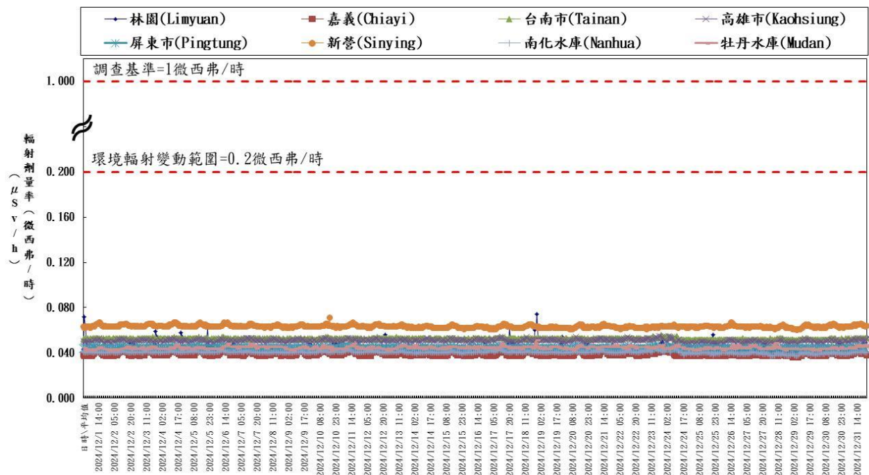
台灣南區輻安預警自動監測時平均劑量率(中華民國一百一十三年十二月) Hourly average dose rates in cities in southern Taiwan (December, 2024)
