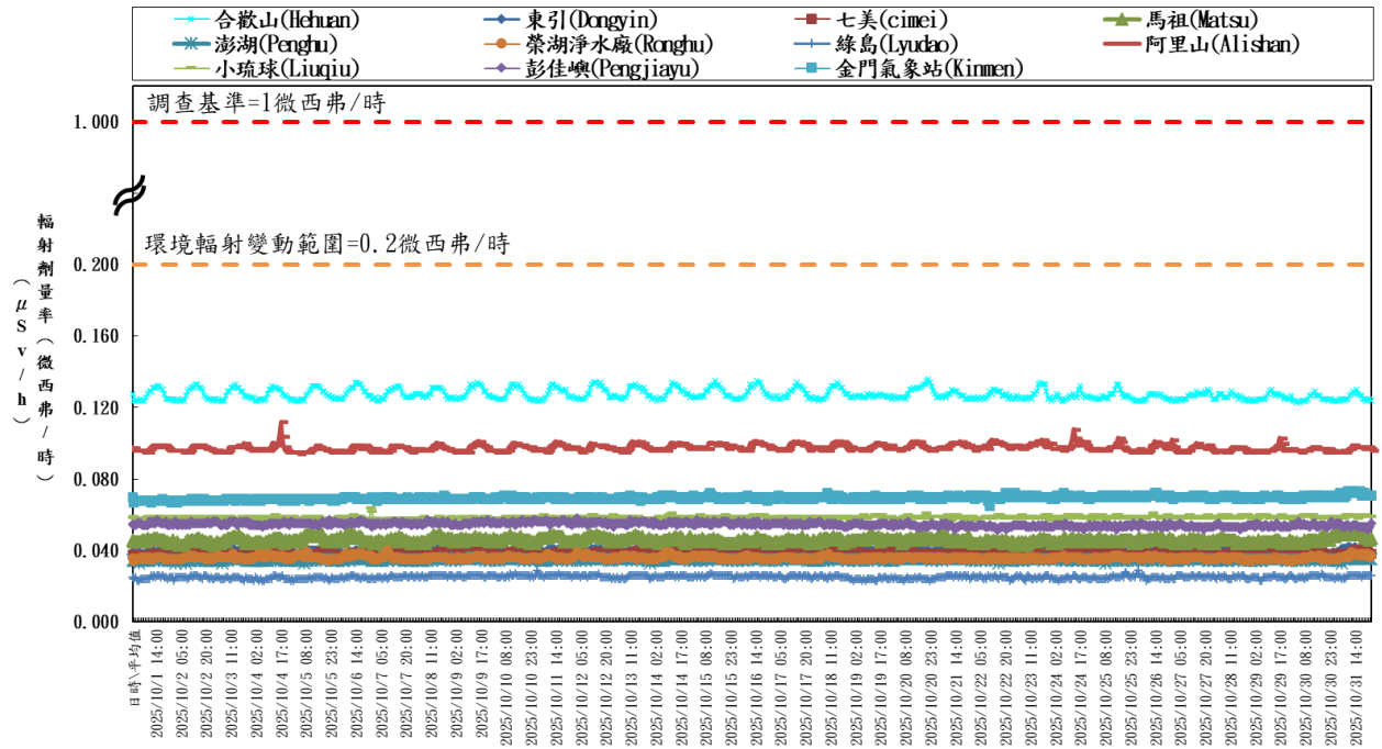
圖 11 台灣外島高山地區輻安預警自動監測劑量率時變動圖
