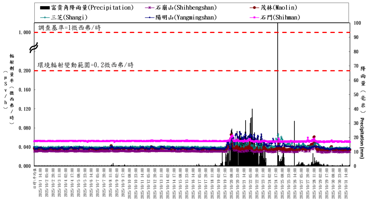
核一廠輻安預警自動監測時平均劑量率(中華民國一百一十四年十月) Hourly average dose rates around NPP1 in Taiwan (October, 2025)
