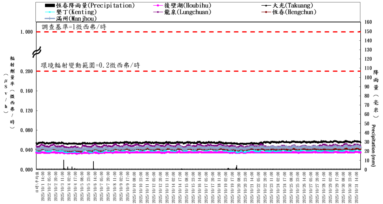
核三廠輻安預警自動監測時平均劑量率(中華民國一百一十四年十月) Hourly average dose rates around NPP3 in Taiwan (October, 2025)
