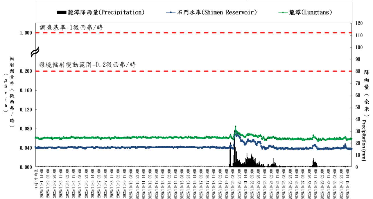
國原院輻安預警自動監測時平均劑量率(中華民國一百一十四年十月) Hourly average dose rates around NARI in Taiwan (October, 2025)
