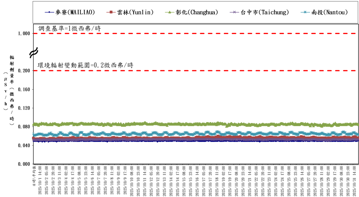
台灣中區輻安預警自動監測時平均劑量率(中華民國一百一十四年十月) Hourly average dose rates in cities in central Taiwan (October, 2025)
