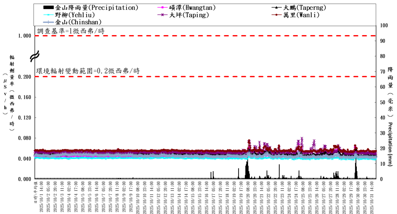
核二廠輻安預警自動監測時平均劑量率(中華民國一百一十四年十月) Hourly average dose rates around NPP2 in Taiwan (October, 2025)
