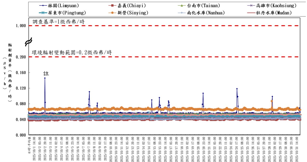
台灣南區輻安預警自動監測時平均劑量率(中華民國一百一十四年十月) Hourly average dose rates in cities in southern Taiwan (October, 2025)
