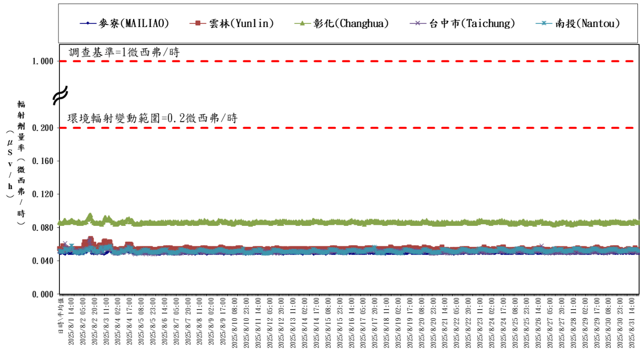
台灣中區輻安預警自動監測時平均劑量率(中華民國一百一十四年八月) Hourly average dose rates in cities in central Taiwan (August, 2025)
