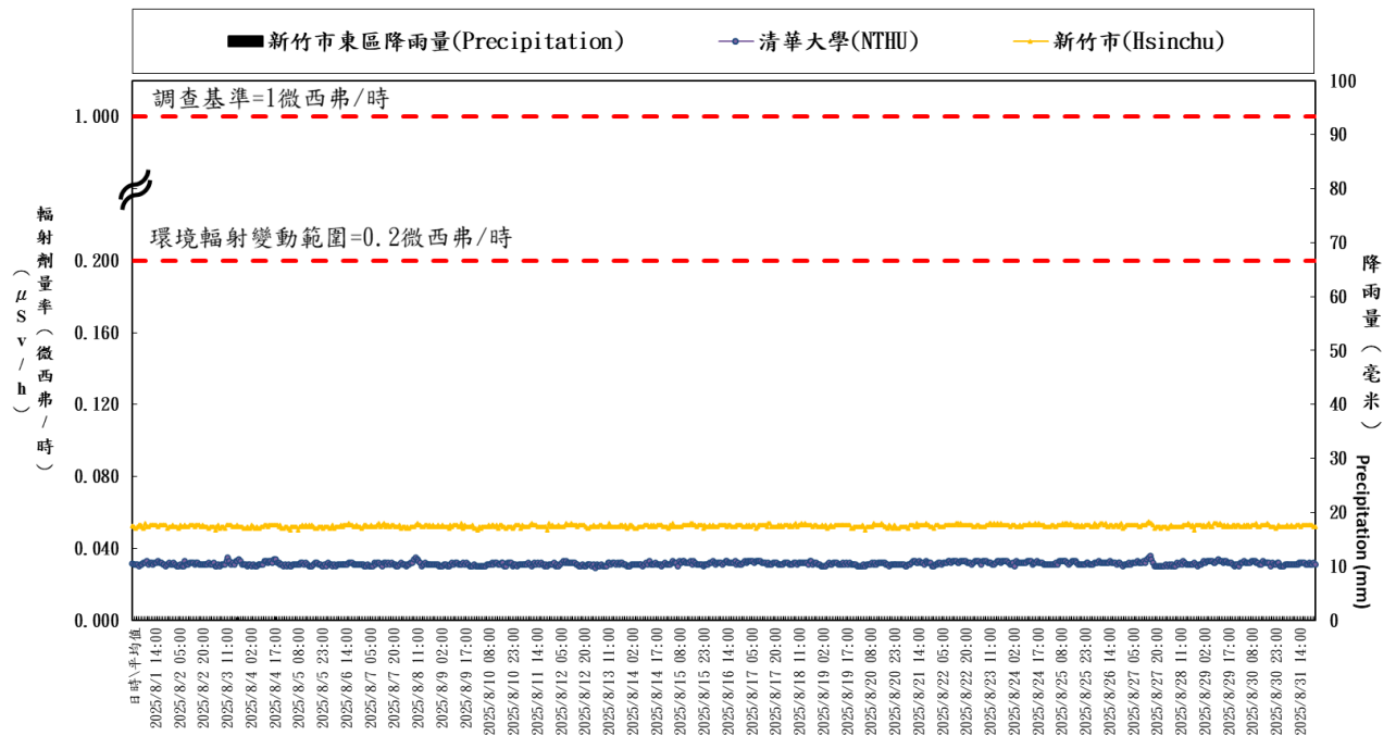
清華大學輻安預警自動監測時平均劑量率(中華民國一百一十四年八月) Hourly average dose rates around NTHU in Taiwan (August, 2025)
