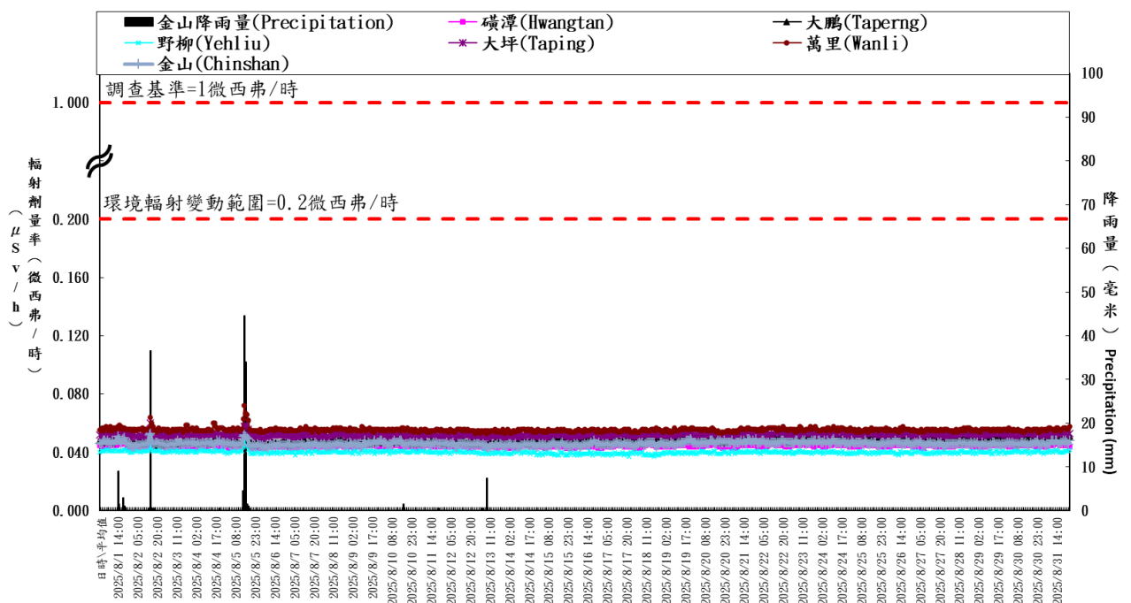
核二廠輻安預警自動監測時平均劑量率(中華民國一百一十四年八月)
