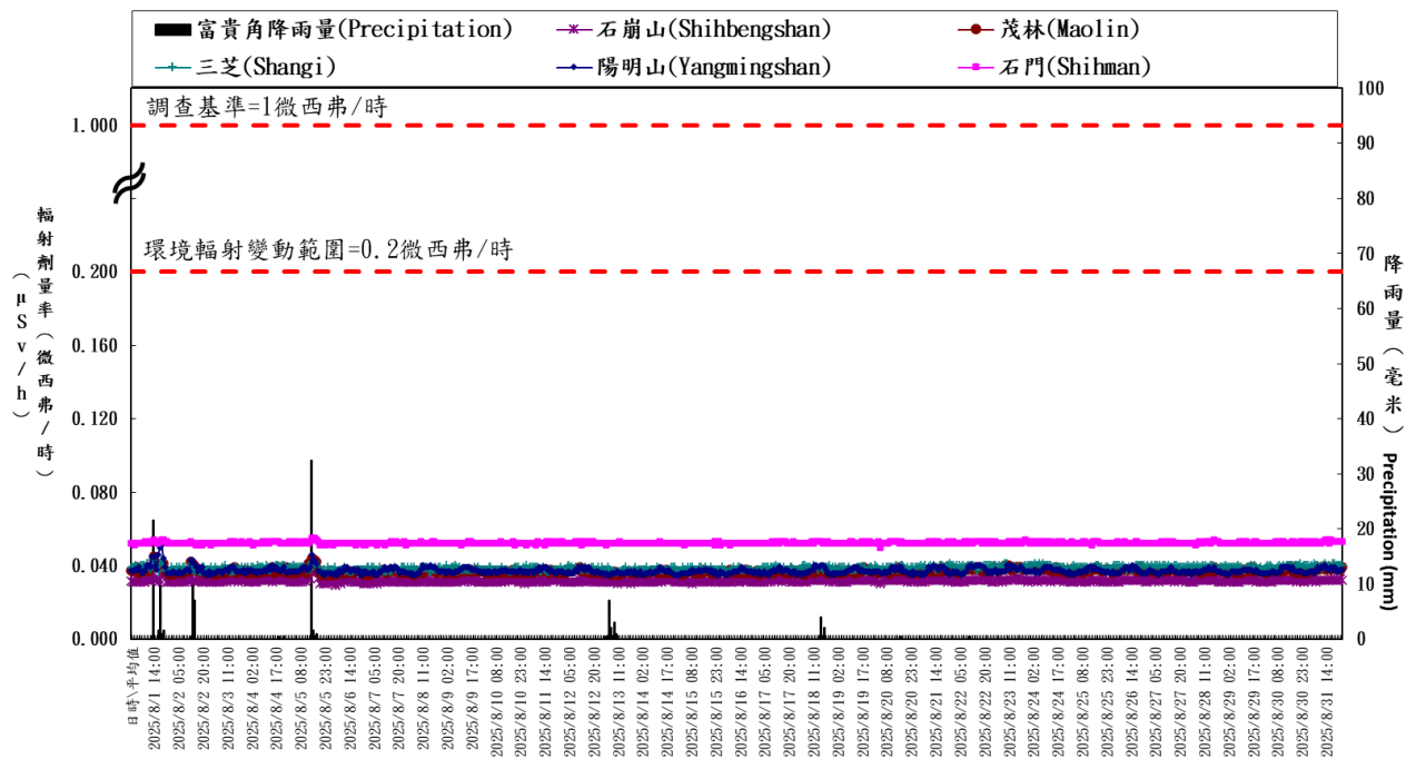
核一廠輻安預警自動監測時平均劑量率(中華民國一百一十四年八月)
