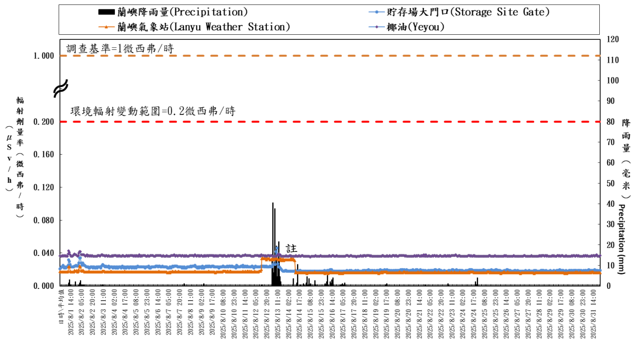
蘭嶼地區輻安預警自動監測時平均劑量率(中華民國一百一十四年八月) Hourly average dose rates in Lanyu island (August, 2025)
