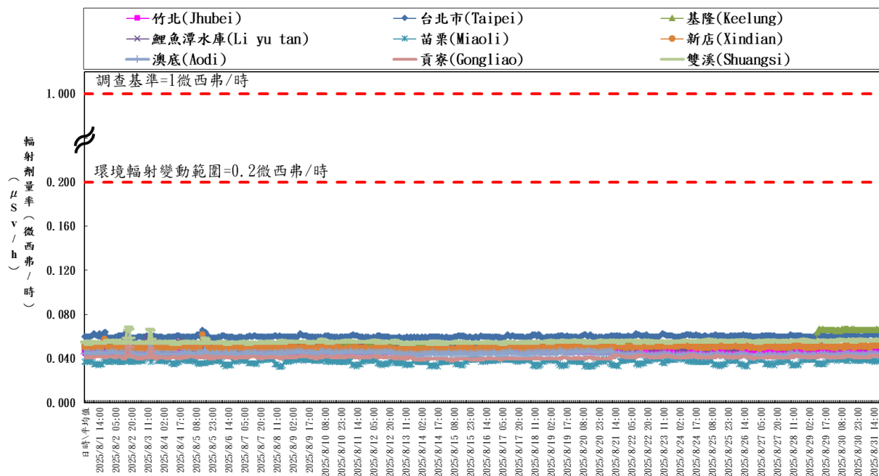
台灣北區輻安預警自動監測時平均劑量率(中華民國一百一十四年八月) Hourly average dose rates in cities in northern Taiwan(August, 2025)
