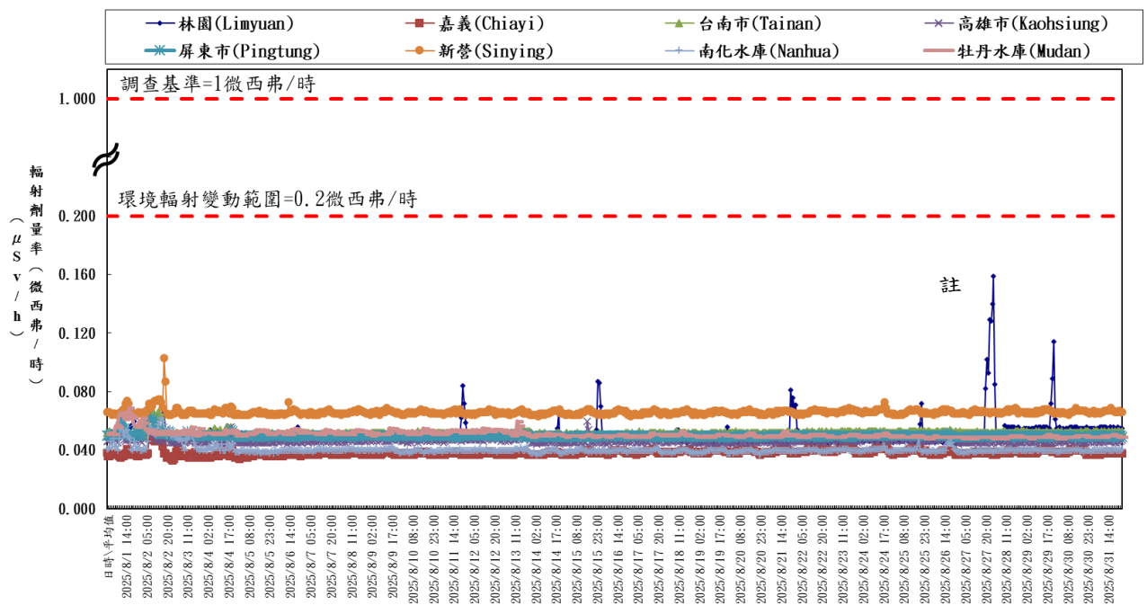
台灣南區輻安預警自動監測時平均劑量率(中華民國一百一十四年八月) Hourly average dose rates in cities in southern Taiwan (August, 2025)
