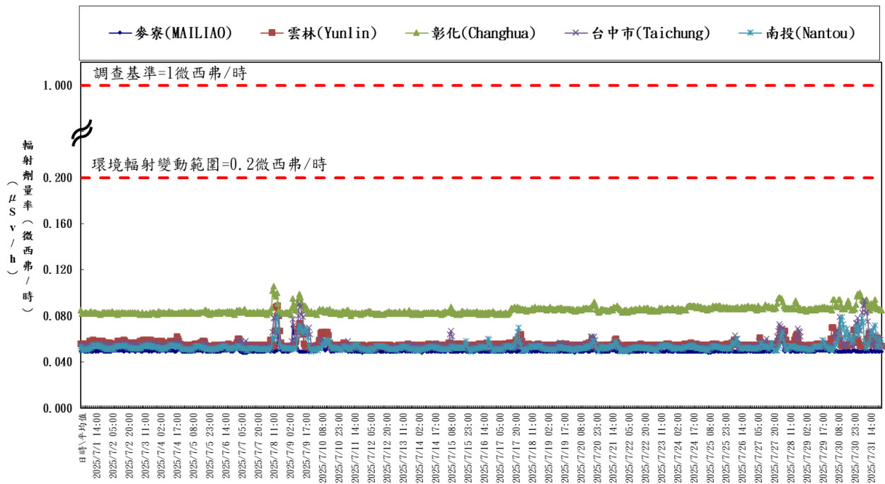
台灣中區輻安預警自動監測時平均劑量率(中華民國一百一十四年七月) Hourly average dose rates in cities in central Taiwan (July, 2025)
