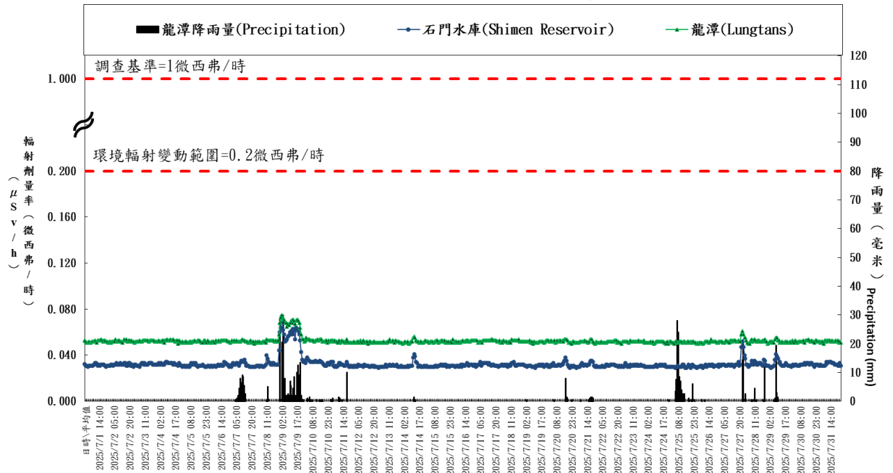
國原院輻安預警自動監測時平均劑量率(中華民國一百一十四年七月) Hourly average dose rates around NARI in Taiwan (July, 2025)
