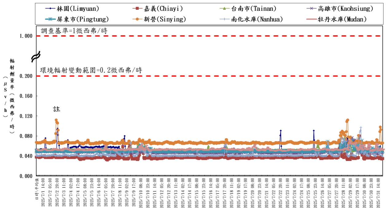
台灣南區輻安預警自動監測時平均劑量率(中華民國一百一十四年七月) Hourly average dose rates in cities in southern Taiwan (July, 2025)
