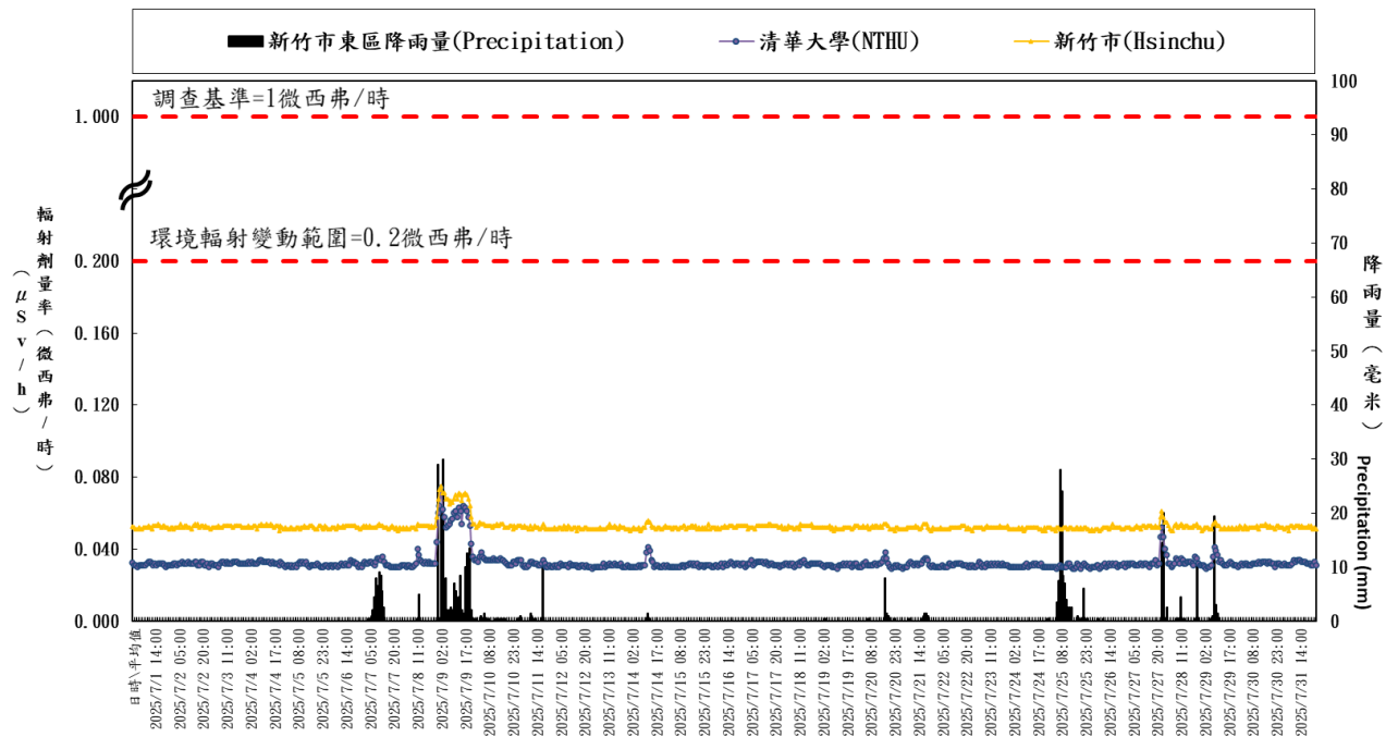
清華大學輻安預警自動監測時平均劑量率(中華民國一百一十四年七月)
