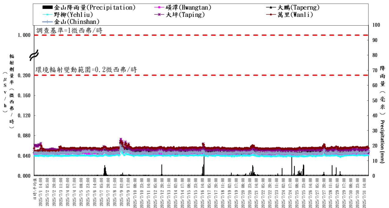
核二廠輻安預警自動監測時平均劑量率(中華民國一百一十四年七月) Hourly average dose rates around NPP2 in Taiwan (July, 2025)
