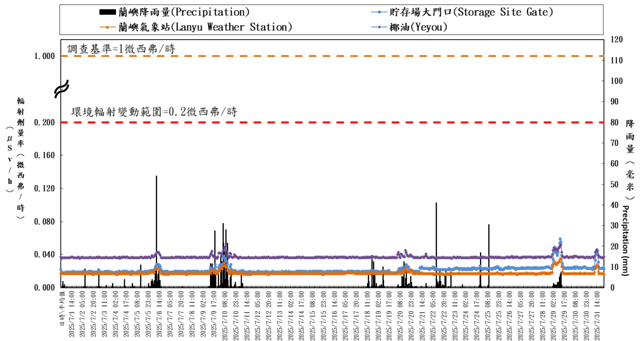
蘭嶼地區輻安預警自動監測時平均劑量率(中華民國一百一十四年七月)
