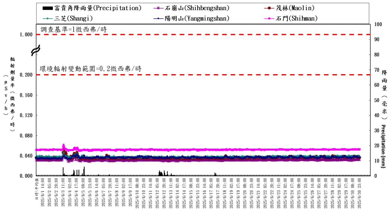
核一廠輻安預警自動監測時平均劑量率(中華民國一百一十四年六月)
