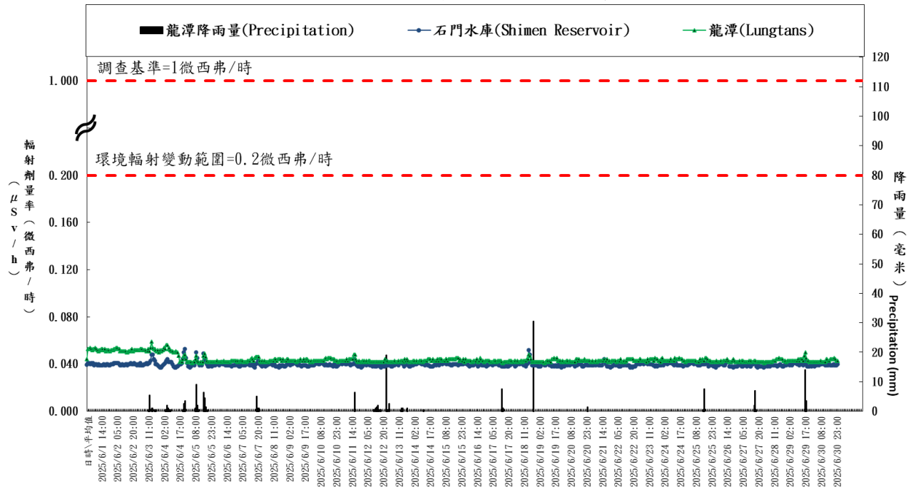
國原院輻安預警自動監測時平均劑量率(中華民國一百一十四年六月) Hourly average dose rates around NARI in Taiwan (June, 2025)
