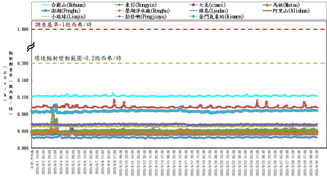
台灣外島與高山地區輻安預警自動監測時平均劑量率(中華民國一百一十四年六月) Hourly average dose rates in mountain and islands in Taiwan (June, 2025)
