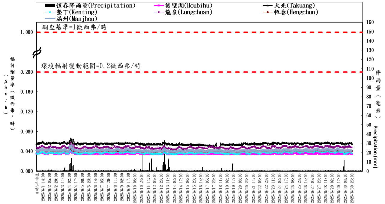
核三廠輻安預警自動監測時平均劑量率(中華民國一百一十四年六月) Hourly average dose rates around NPP3 in Taiwan (June, 2025)
