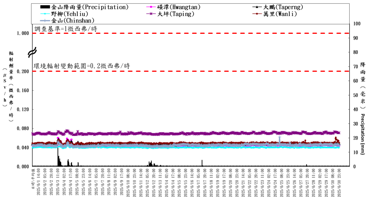
核二廠輻安預警自動監測時平均劑量率(中華民國一百一十四年六月)
