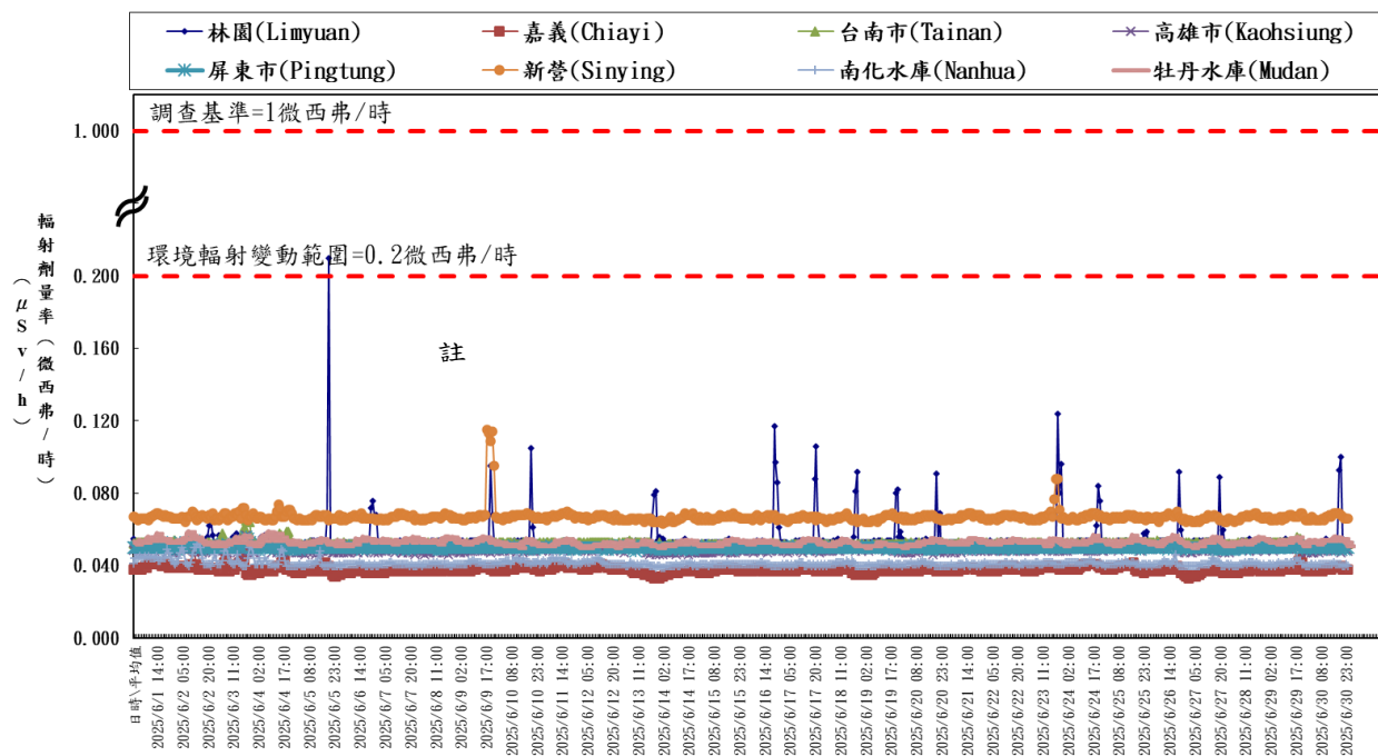
台灣南區輻安預警自動監測時平均劑量率(中華民國一百一十四年六月) Hourly average dose rates in cities in southern Taiwan (June, 2025)
