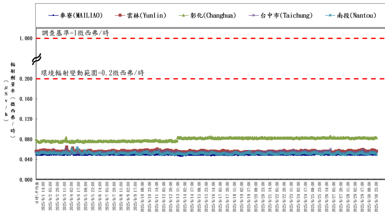
台灣中區輻安預警自動監測時平均劑量率(中華民國一百一十四年六月) Hourly average dose rates in cities in central Taiwan (June, 2025)
