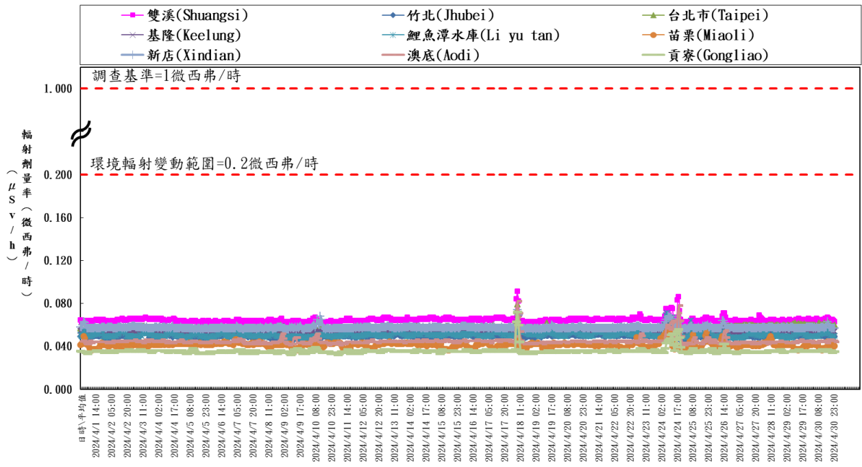
台灣北區輻安預警自動監測時平均劑量率(中華民國一百一十三年四月) Hourly average dose rates in cities in northern Taiwan(April, 2024)
