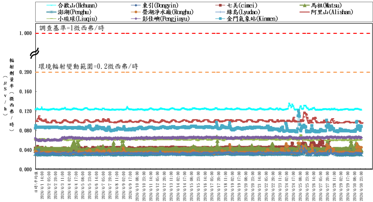
台灣外島與高山地區輻安預警自動監測時平均劑量率(中華民國一百一十三年四月) Hourly average dose rates in mountain and islands in Taiwan (April, 2024)
