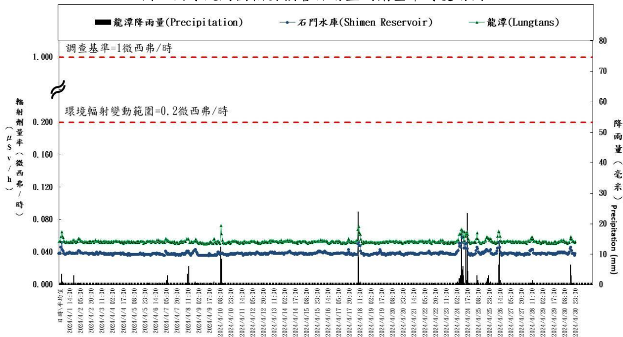
國原院輻安預警自動監測時平均劑量率(中華民國一百一十三年四月) Hourly average dose rates around NARI in Taiwan (April, 2024)
