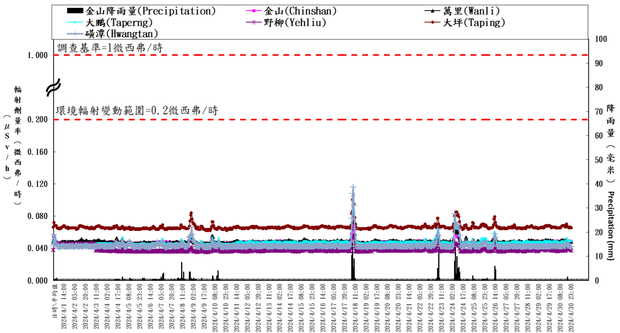
核二廠輻安預警自動監測時平均劑量率(中華民國一百一十三年四月) Hourly average dose rates around NPP2 in Taiwan (April, 2024)
