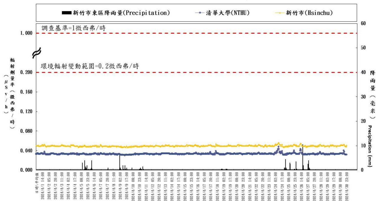
清華大學輻安預警自動監測時平均劑量率(中華民國一百一十三年四月) Hourly average dose rates around NTHU in Taiwan (April, 2024)
