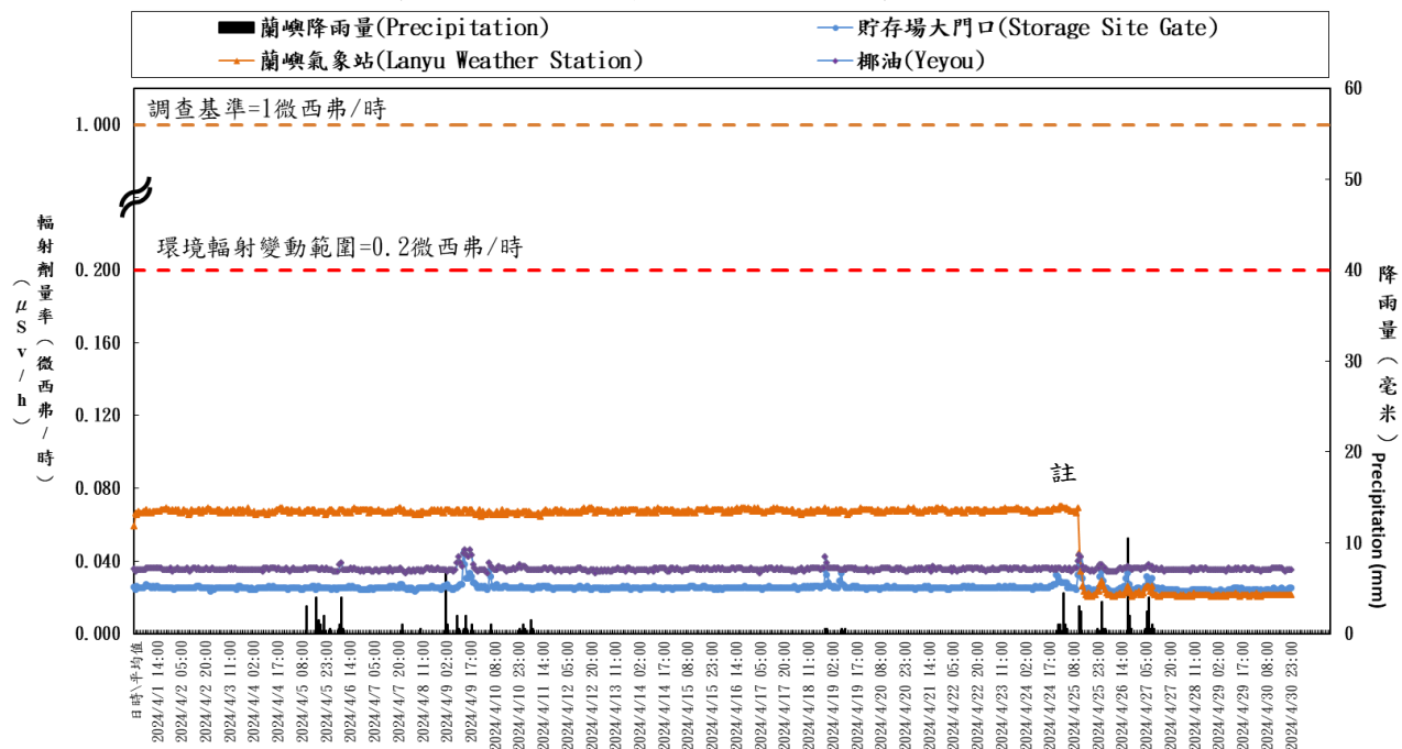
蘭嶼地區輻安預警自動監測時平均劑量率(中華民國一百一十三年四月) Hourly average dose rates in Lanyu island (April, 2024)
