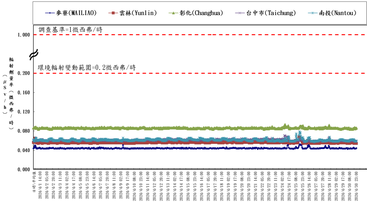
台灣中區輻安預警自動監測時平均劑量率(中華民國一百一十三年四月) Hourly average dose rates in cities in central Taiwan (April, 2024)
