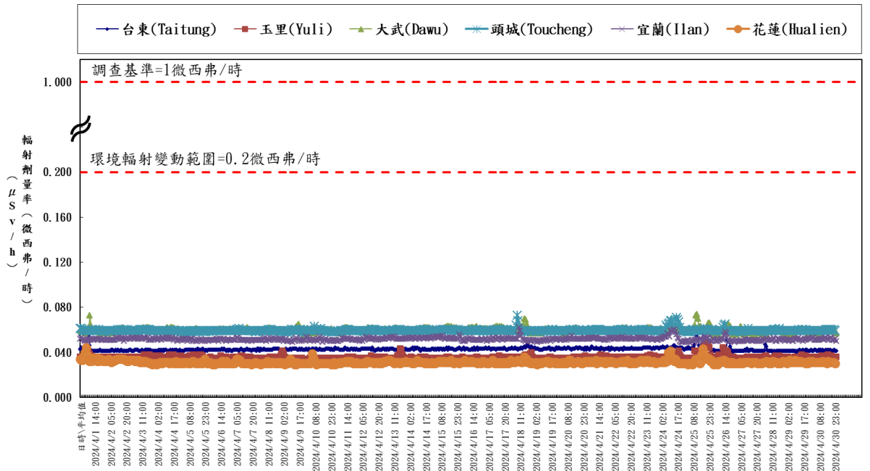
台灣東區輻安預警自動監測時平均劑量率(中華民國一百一十三年四月) Hourly average dose rates in cities in eastern Taiwan (April, 2024)
