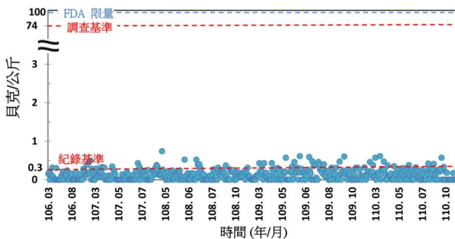
圖 26 106 年至 110 年台灣周邊海域岸沙銫-137 背景數據
