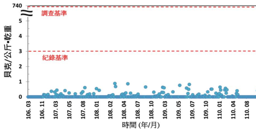
圖 26 106 年至 110 年台灣周邊海域岸沙銫-137 背景數據
