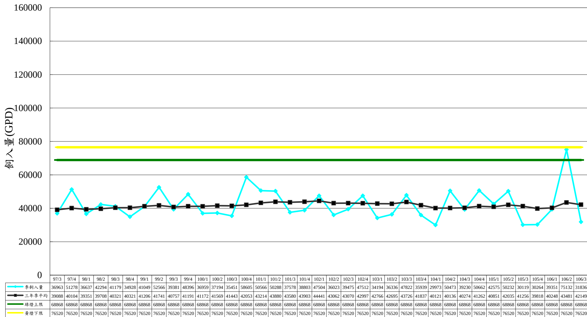
圖1-1 核二廠97~106年廢液飼入量圖
