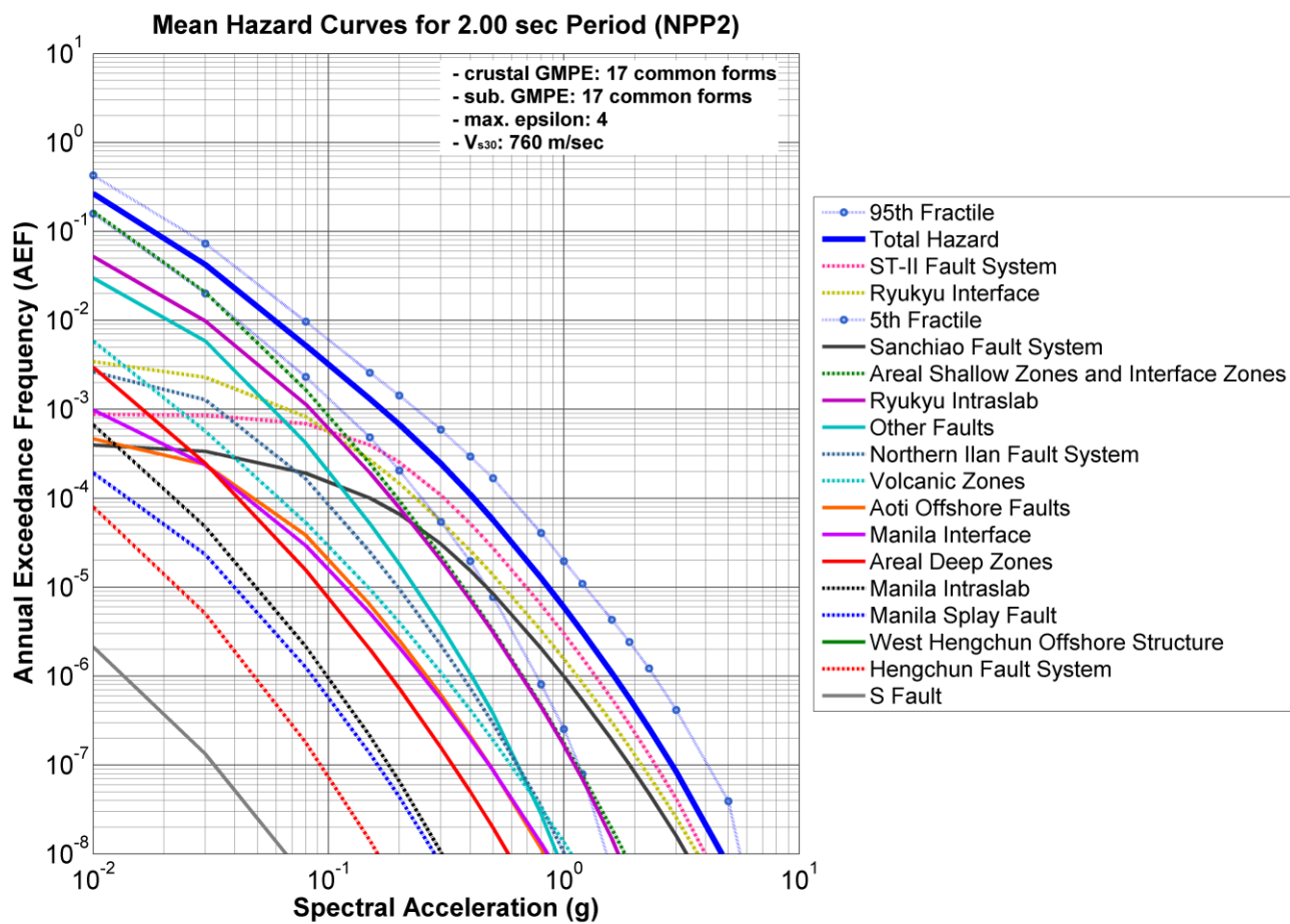
圖 3 核二廠 2.0 秒週期之參考岩盤均值地震危害度曲線
