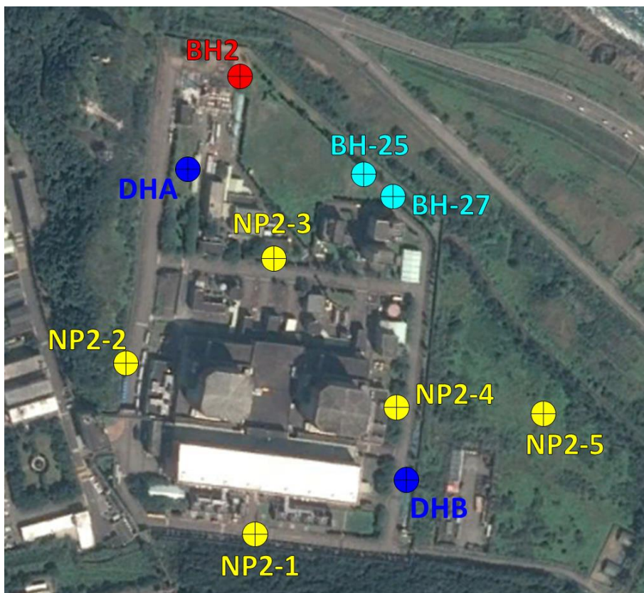
圖 15 核二廠速度井測鑽孔位置圖
