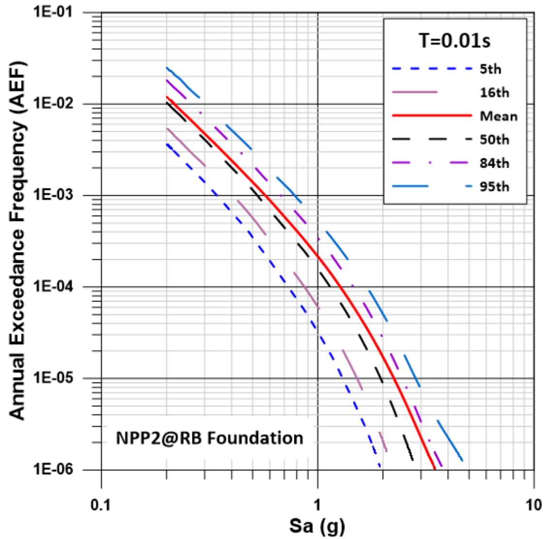
圖 43 核二廠控制點 0.01 秒週期地震危害度曲線
