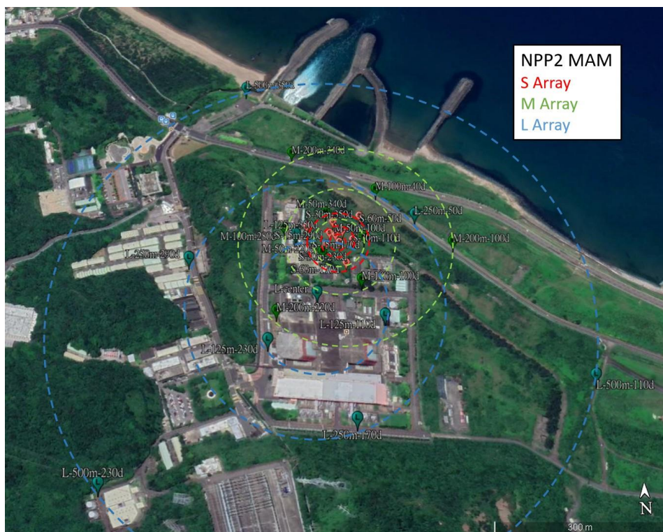
圖 19 核二廠大(藍圈)、中(綠圈)、小(紅圈)陣列量測配置
