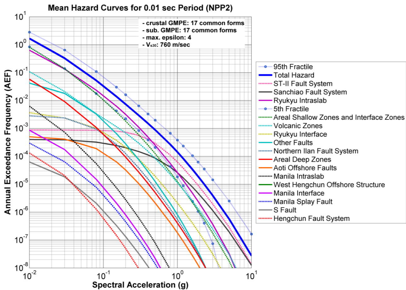
圖 2 核二廠 0.01 秒週期之參考岩盤均值地震危害度曲線
