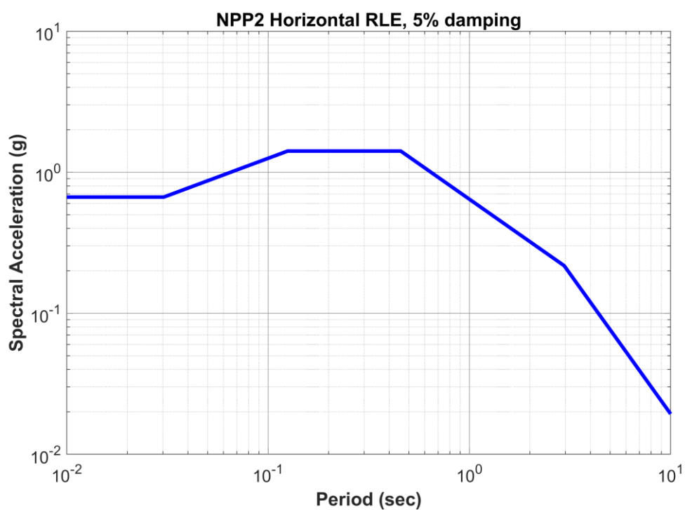
圖 49 核二廠 5%阻尼比評估基準地震(RLE)反應譜
