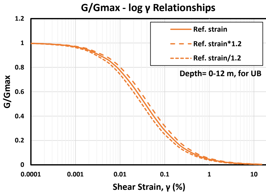
(a) 剪力模數折減曲線
