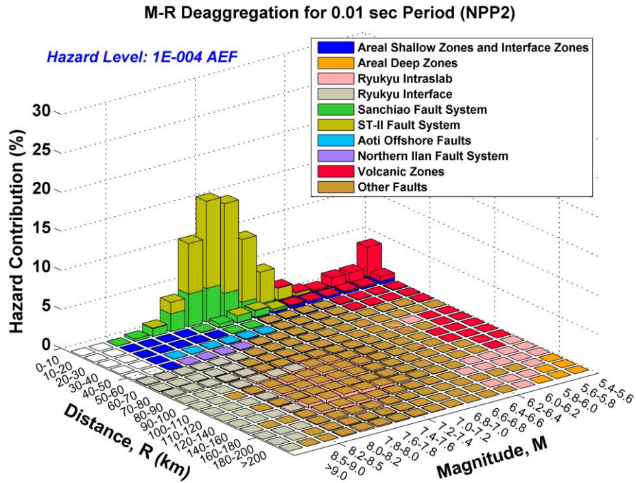
圖 8 核二廠 0.01 秒週期在 1E-04 年超越頻率水準之參考岩盤 均值地震危害度參數拆解
