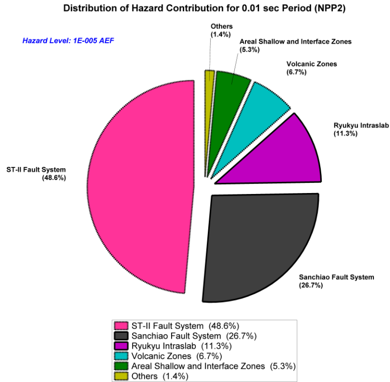
圖 6 核二廠 0.01 秒週期在 1E-05 年超越頻率水準之參考岩盤 均值地震危害度主要貢獻震源百分比
