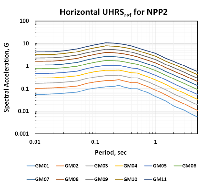
圖 35 核二廠 11 個危害水準之 5%阻尼比參考岩盤均佈危害度反應譜 ( UHRS_{ref} )
