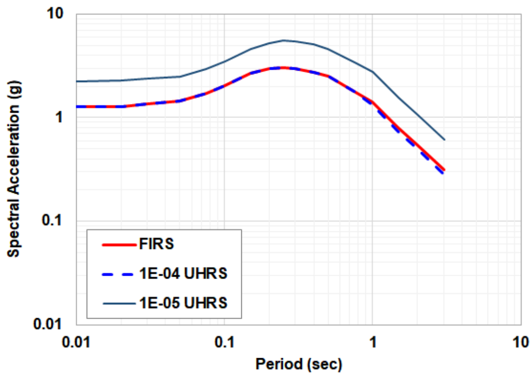
圖 47 核二廠反應器廠房基礎輸入地震反應譜(FIRS)
