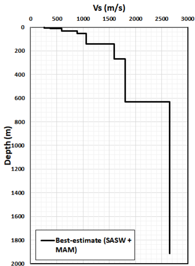
圖 22 由頻散曲線估算之核二廠最佳估值(BE)淺部剪力波速基準剖面
