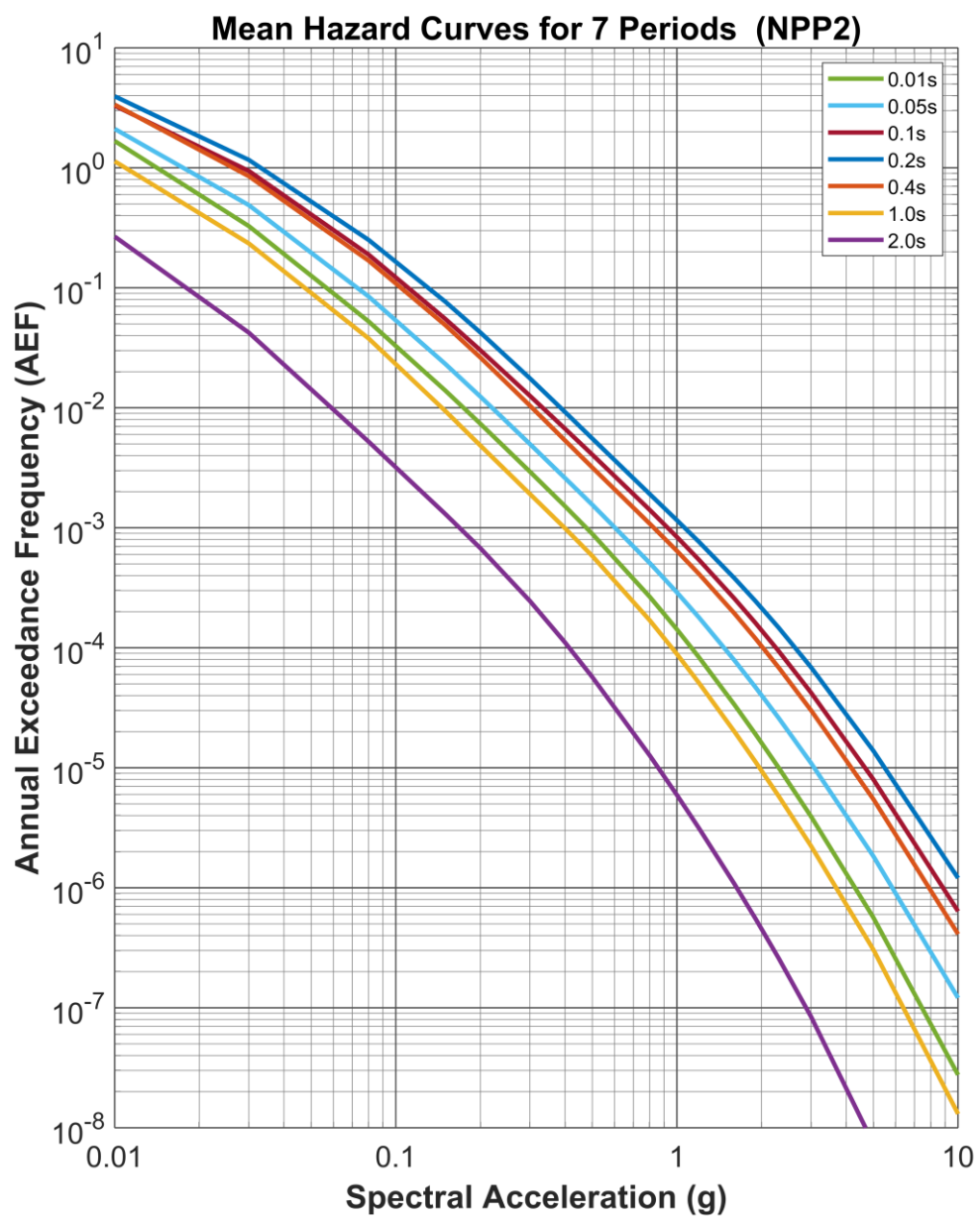
圖 12 核二廠 7 個週期之參考岩盤均值譜加速度地震危害度曲線
