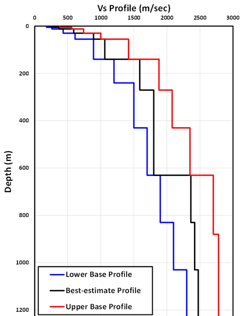
圖 23 核二廠 3 組淺部剪力波速基準剖面
