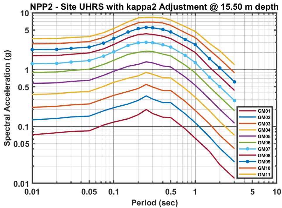
圖 46 核二廠控制點 11 個危害水準之均佈危害度反應譜
