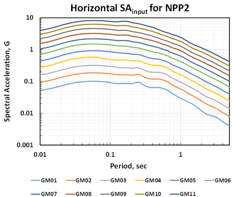
圖 35 核二廠 11 個危害水準之 5%阻尼比參考岩盤均佈危害度反應譜 ( UHRS_{ref} )
