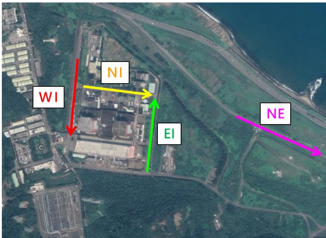
圖 17 核二廠表面波譜分析(SASW)試驗測線佈設位置圖
