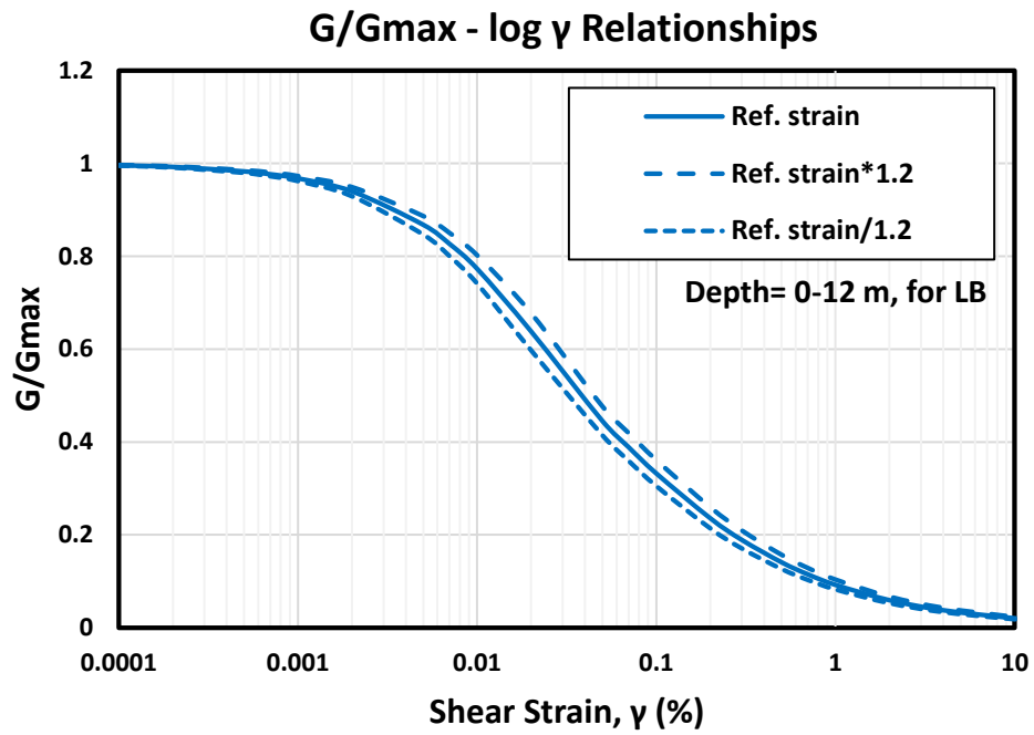
(a) 剪力模數折減曲線
