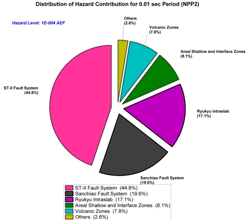
圖 4 核二廠 0.01 秒週期在 1E-04 年超越頻率水準之參考岩盤 均值地震危害度主要貢獻震源百分比
