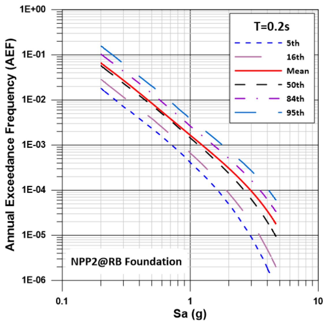
圖 44 核二廠控制點 0.2 秒週期地震危害度曲線
