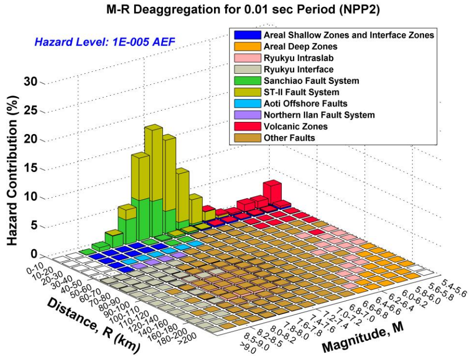
圖 10 核二廠 0.01 秒週期在 1E-05 年超越頻率水準之參考岩盤 均值地震危害度參數拆解
