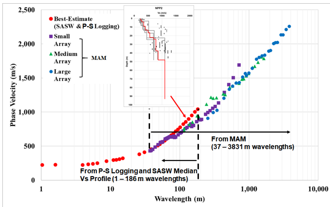
圖 20 核二廠 MAM 頻散曲線(紅實心圓以外)以及 SASW 與可用 P-S Logging 資料估算之頻散曲線(紅實心圓)
