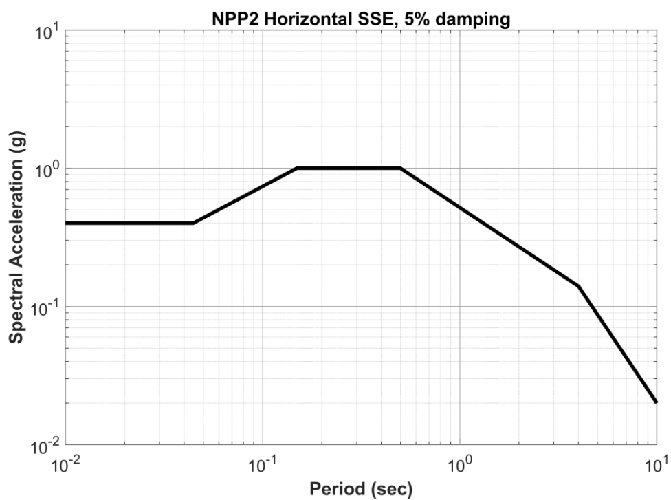
圖 48 核二廠 5%阻尼比安全停機地震(SSE)反應譜
