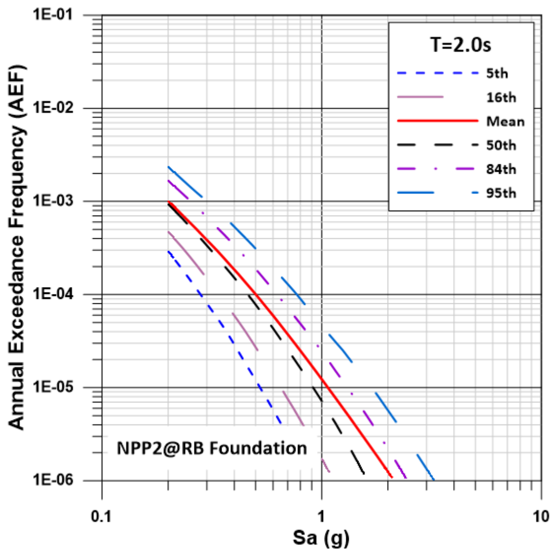
圖 45 核二廠控制點 2.0 秒週期地震危害度曲線
