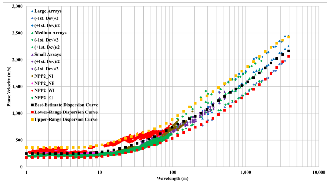
圖 21 核二廠 SASW、MAM 與 3 組淺部剪力波速基準剖面之頻散曲線
