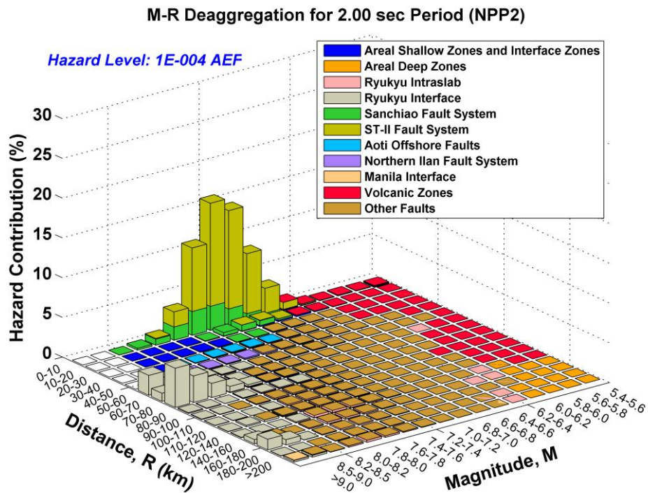
圖 9 核二廠 2.0 秒週期在 1E-04 年超越頻率水準之參考岩盤 均值地震危害度參數拆解
