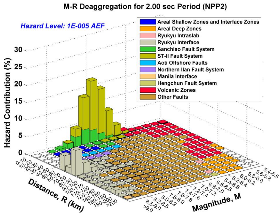
圖 11 核二廠 2.0 秒週期在 1E-05 年超越頻率水準之參考岩盤 均值地震危害度參數拆解
