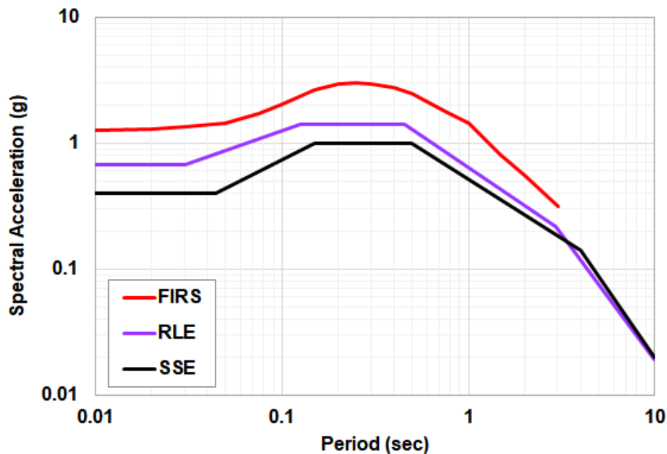
圖 51 核二廠 FIRS 與 SSE 及 RLE 反應譜比較(5%阻尼比)
