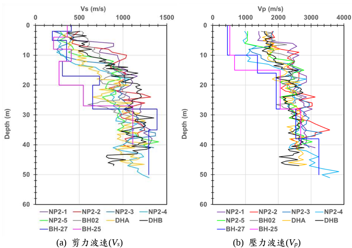
圖 16 核二廠速度井測波速剖面
