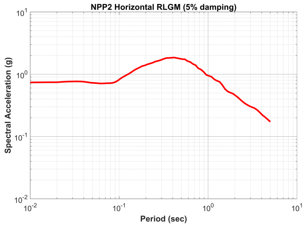
圖 50 核二廠 5%阻尼比評估基準地震動(RLGM)反應譜
