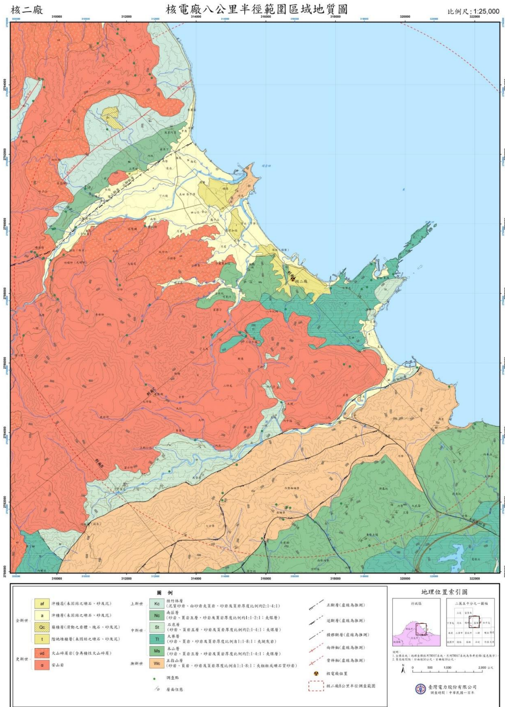
圖 1 核二廠周遭區域地質及斷層圖
