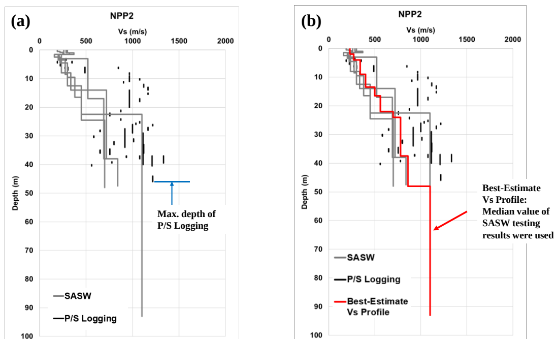
圖 18 依據表面波譜分析(SASW)與可用速度井測試驗量測資料所得波速剖面建立之核二廠最佳估值(BE)基準波速剖面
