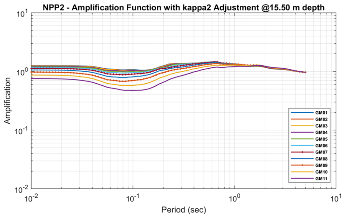
圖 42 核二廠控制點 11 個危害水準之權重後中值放大係數
