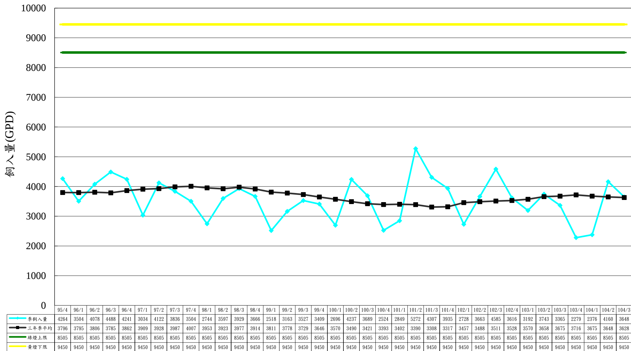
圖3-1 核三廠95~103年廢液飼入量圖
