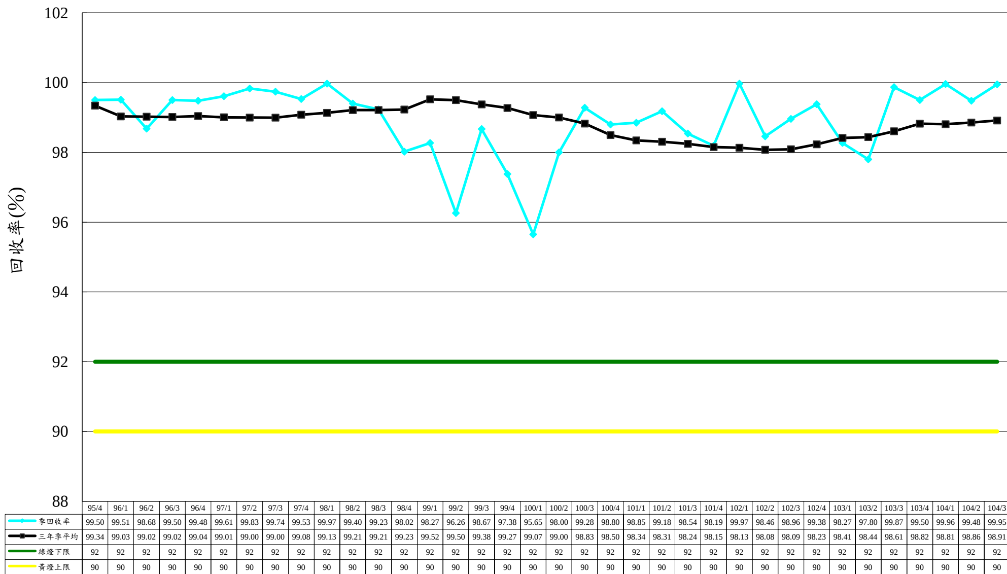
圖1-2 核一廠95~104年廢液回收率圖
