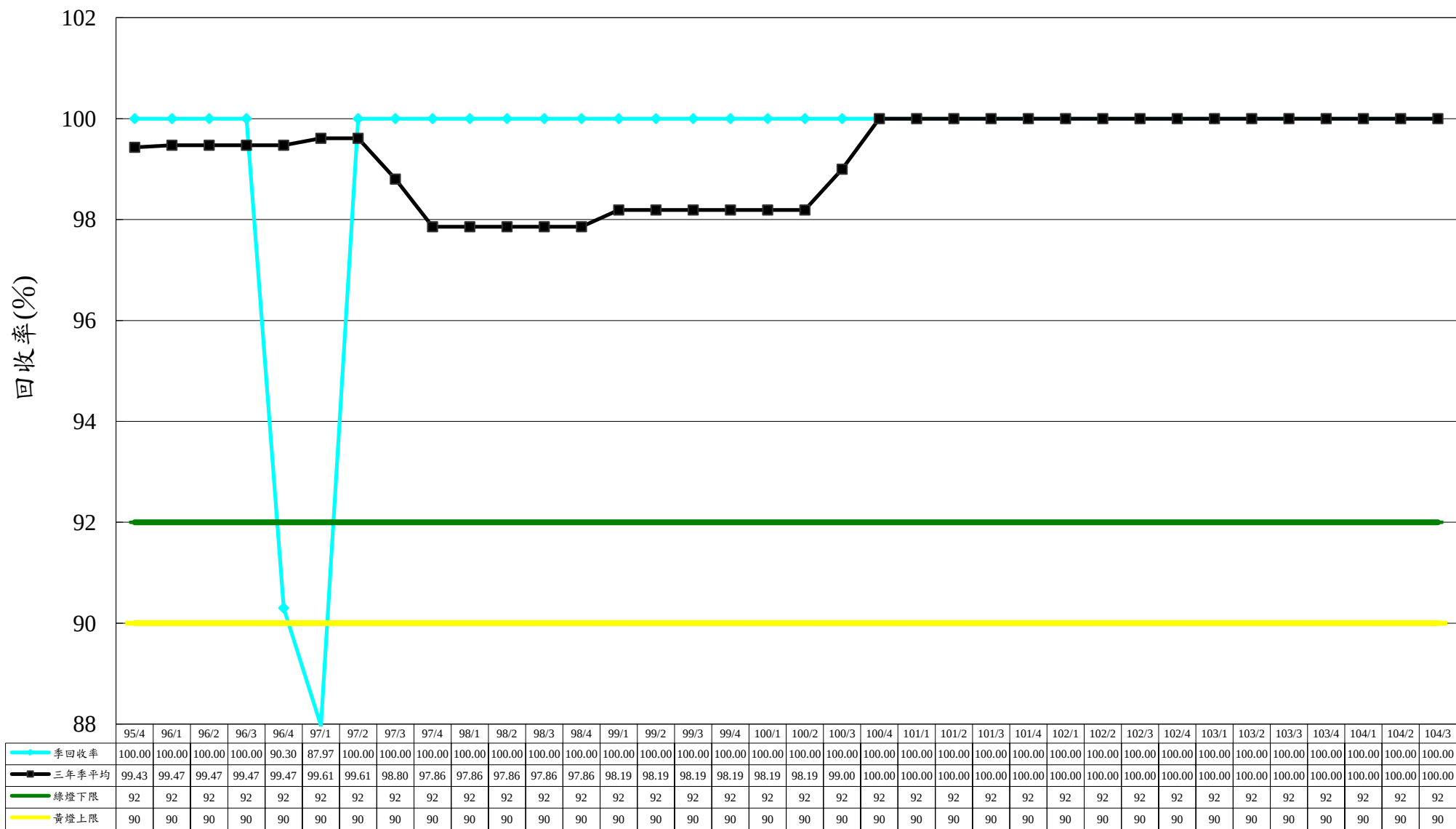
圖2-2 核二廠95~104年廢液回收率圖
