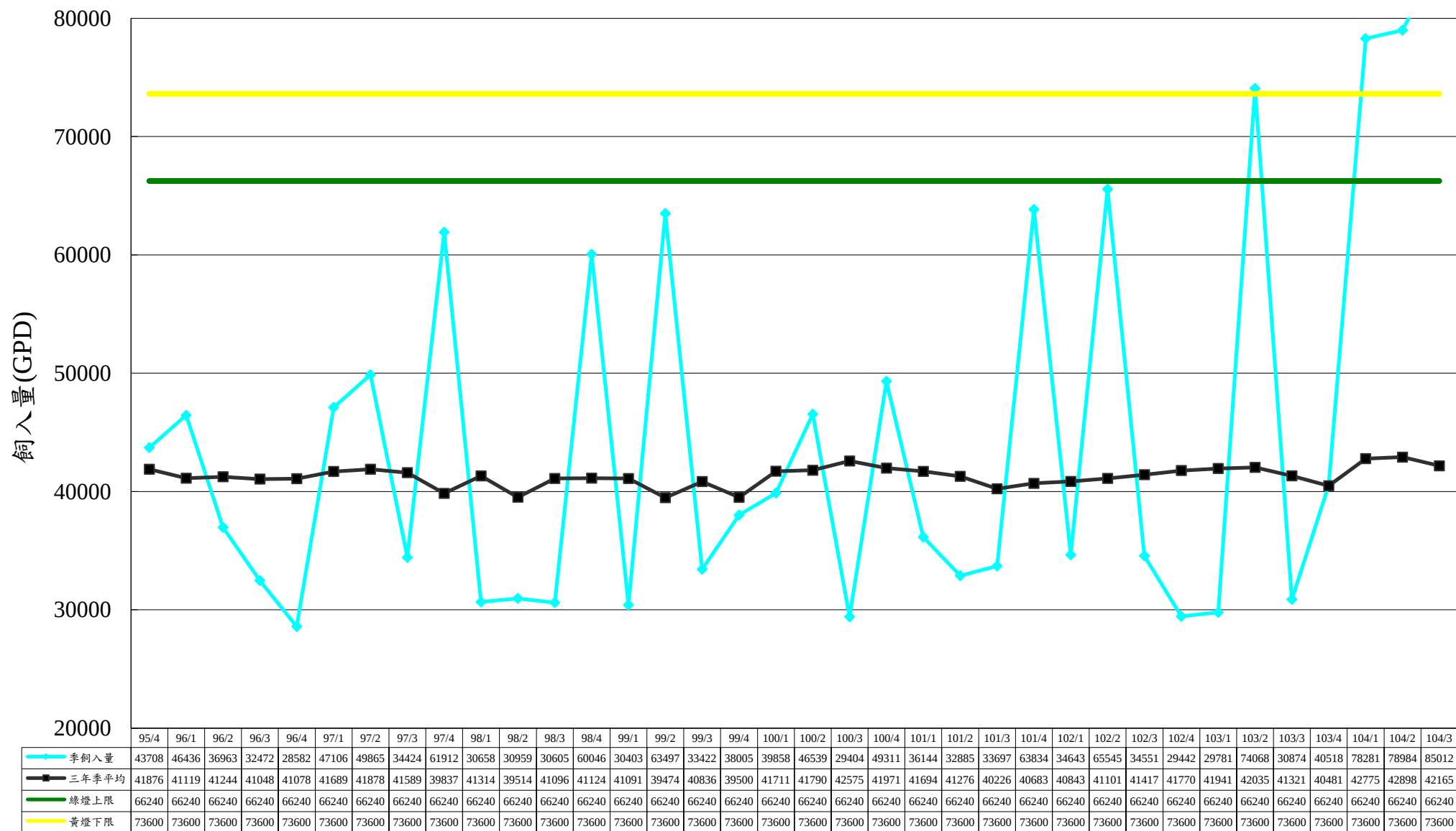
圖1-1 核一廠95~104年廢液飼入量圖
