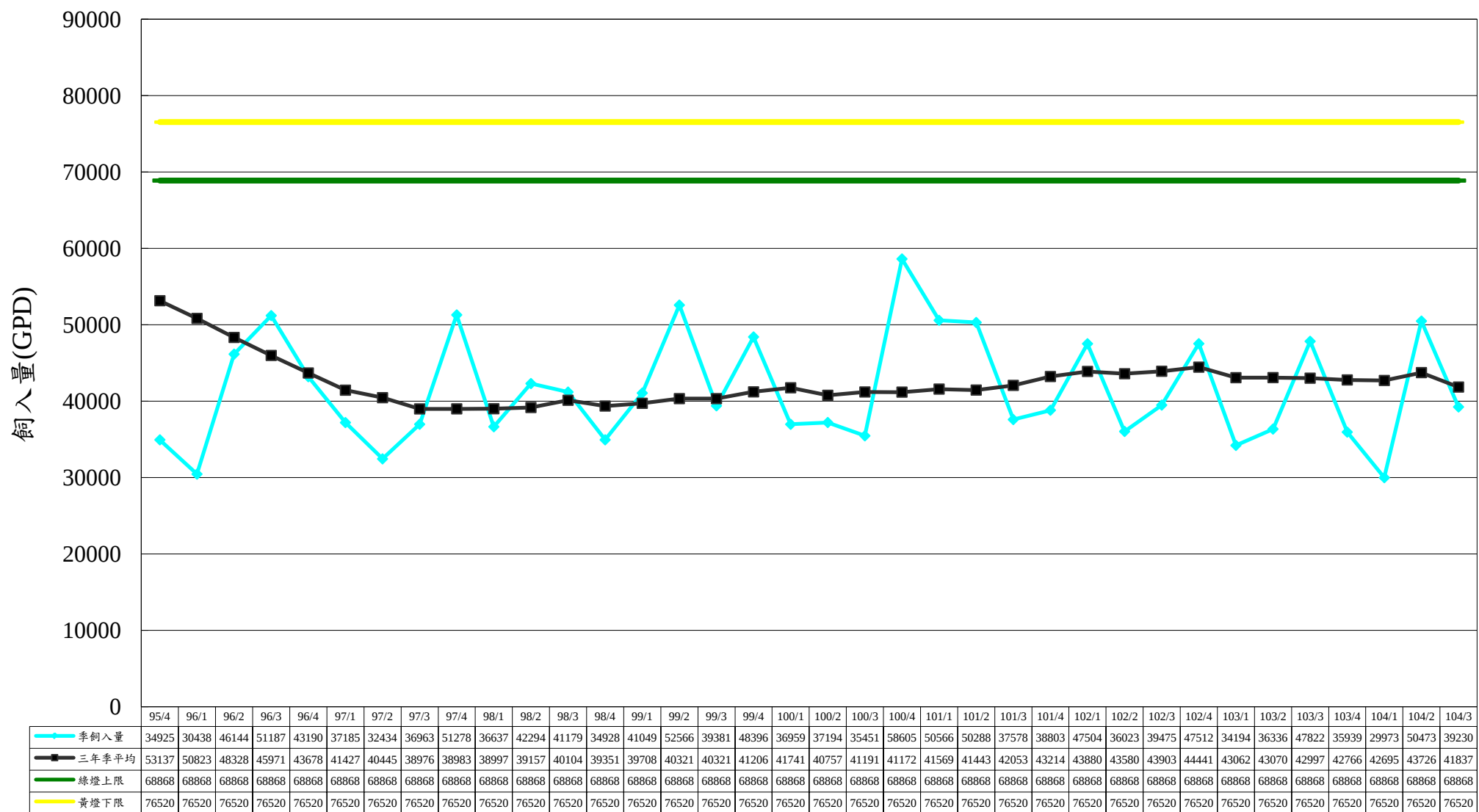
圖2-1 核二廠95~104年廢液飼入量圖
