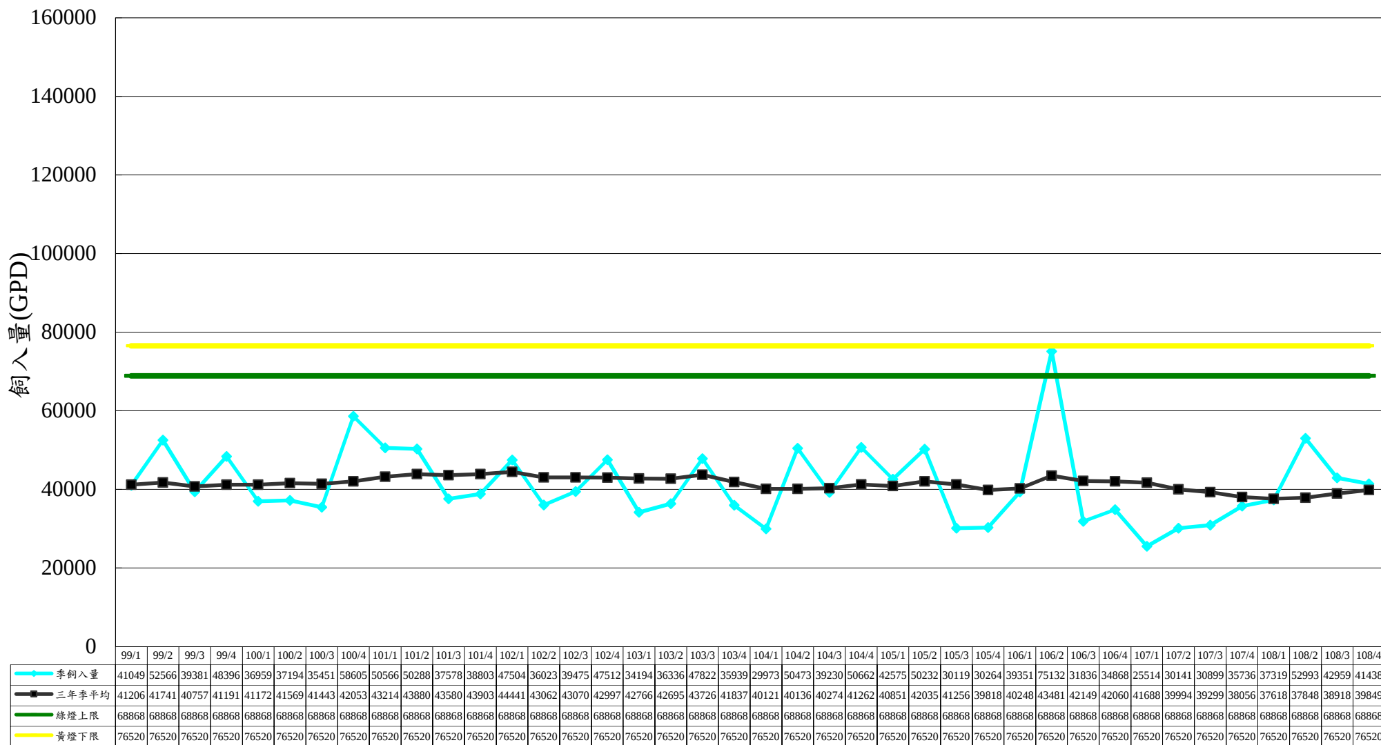
圖1-1 核二廠99~108年廢液飼入量圖
