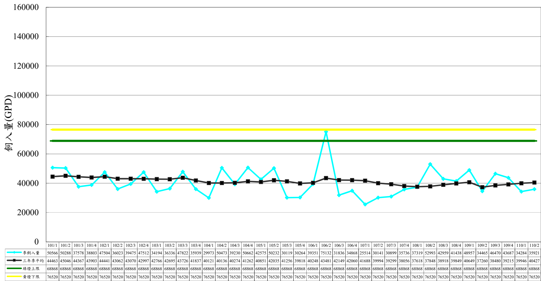
圖1-1 核二廠101~110年廢液飼入量圖
