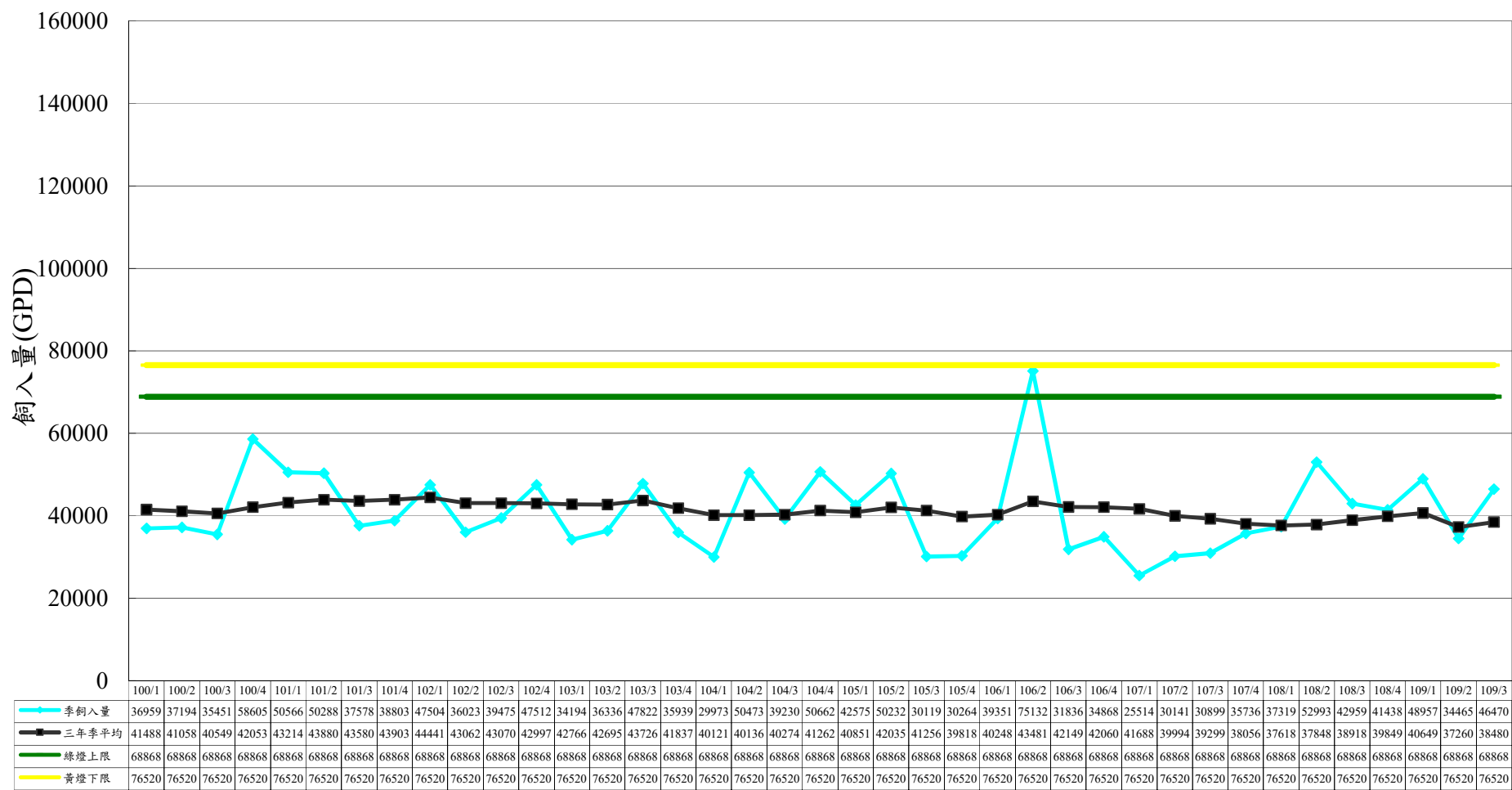
圖1-1 核二廠100~109年廢液飼入量圖
