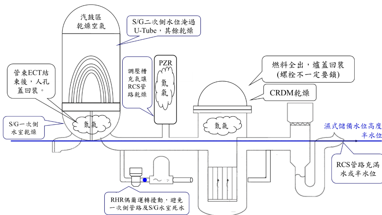
圖 3-1 反應爐冷卻水系統儲備水位高度圖
