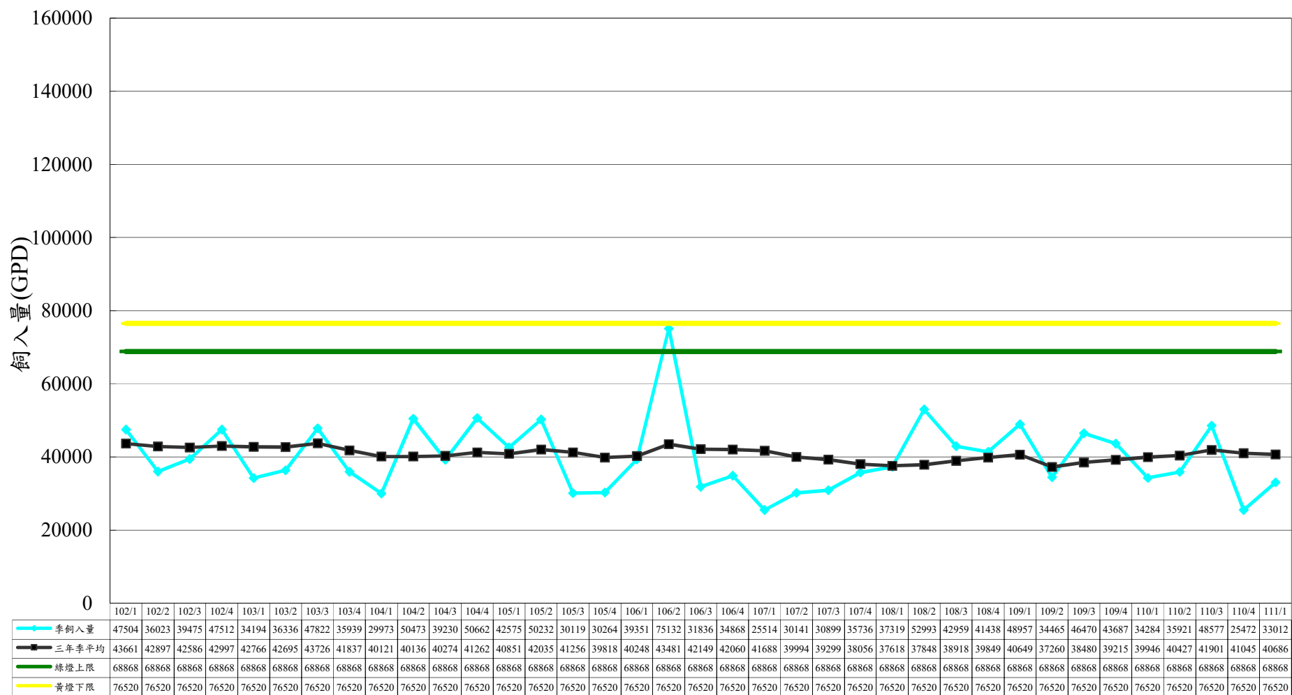
圖1-1 核二廠102~111年廢液飼入量圖
