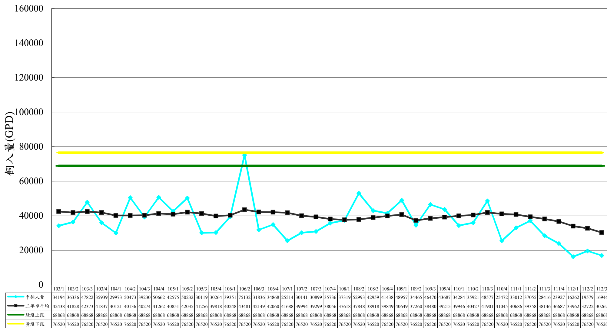
圖1-1 核二廠103~112年廢液飼入量圖
