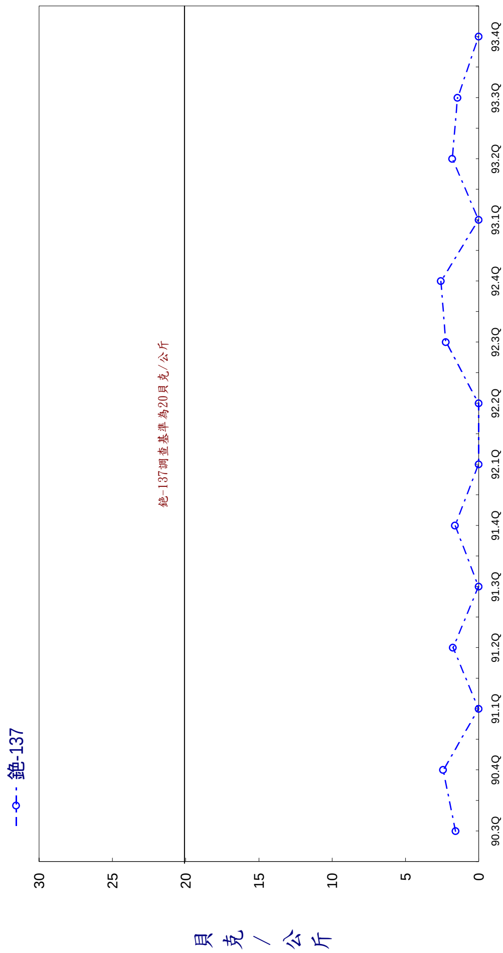
圖4 蘭嶼貯存場排水口岸沙加馬能譜分析結果
