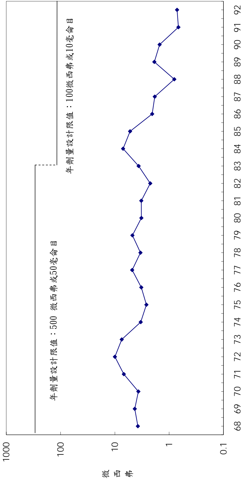
圖17 核能一廠歷年外釋氣體造成廠外民眾之最大個人輻射劑量 年
