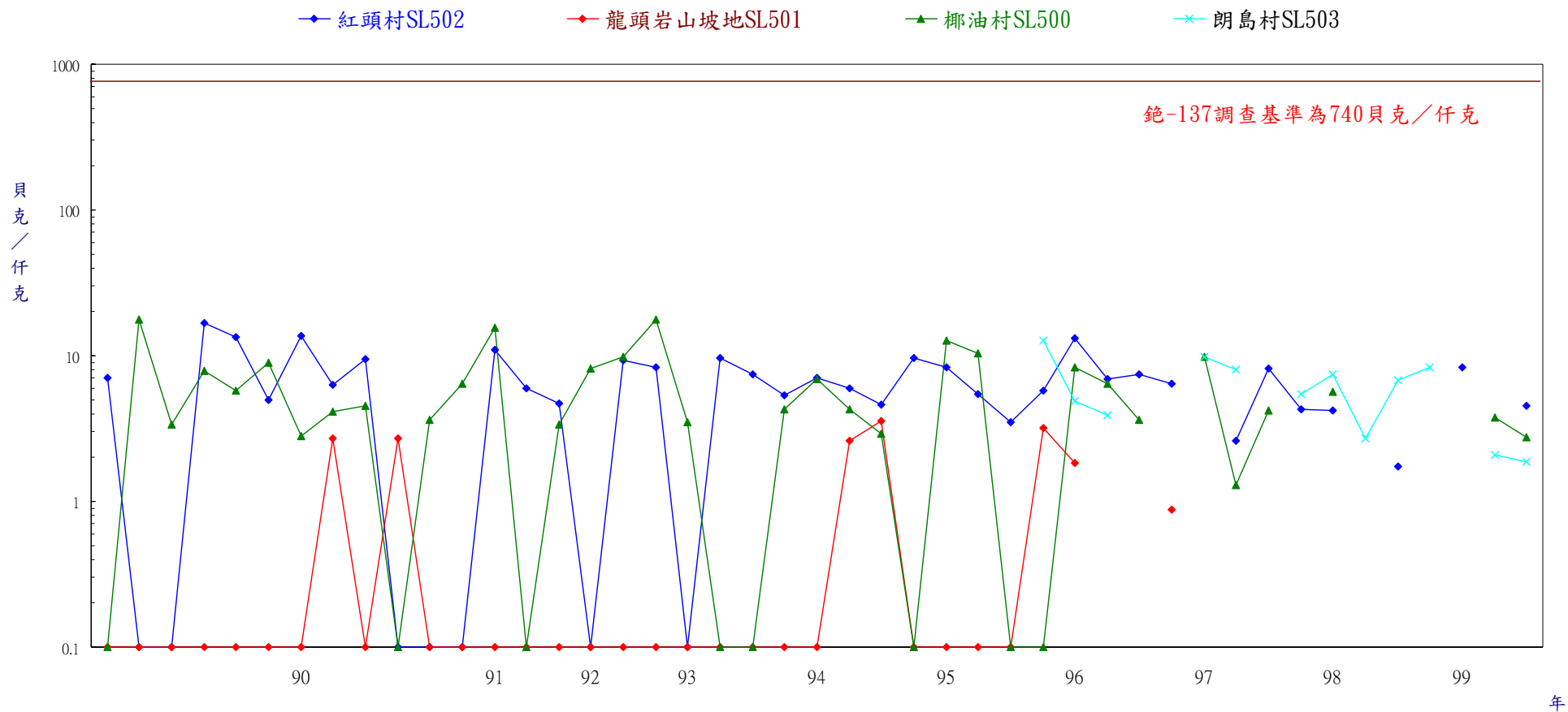
圖3 蘭嶼貯存場土壤鈉-137加馬能譜分析結果
