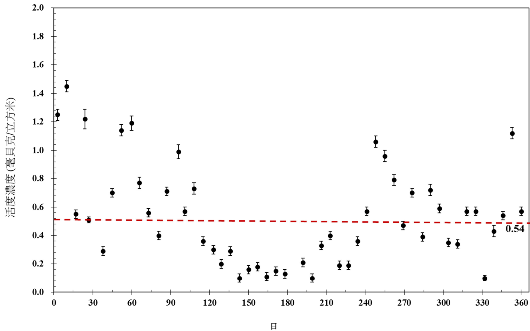
圖7 111年空浮微粒活度濃度變動圖(加速器館)
