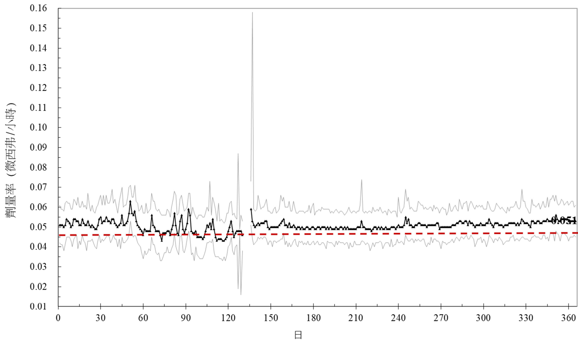
圖 4 111 年連續輻射偵測劑量率變動圖(李存敏館)
