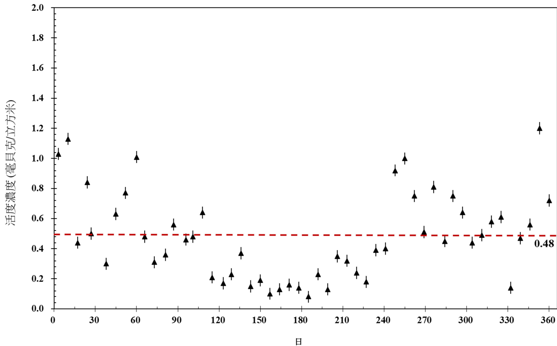
圖6 111年空浮微粒活度濃度變動圖(李存敏館)
