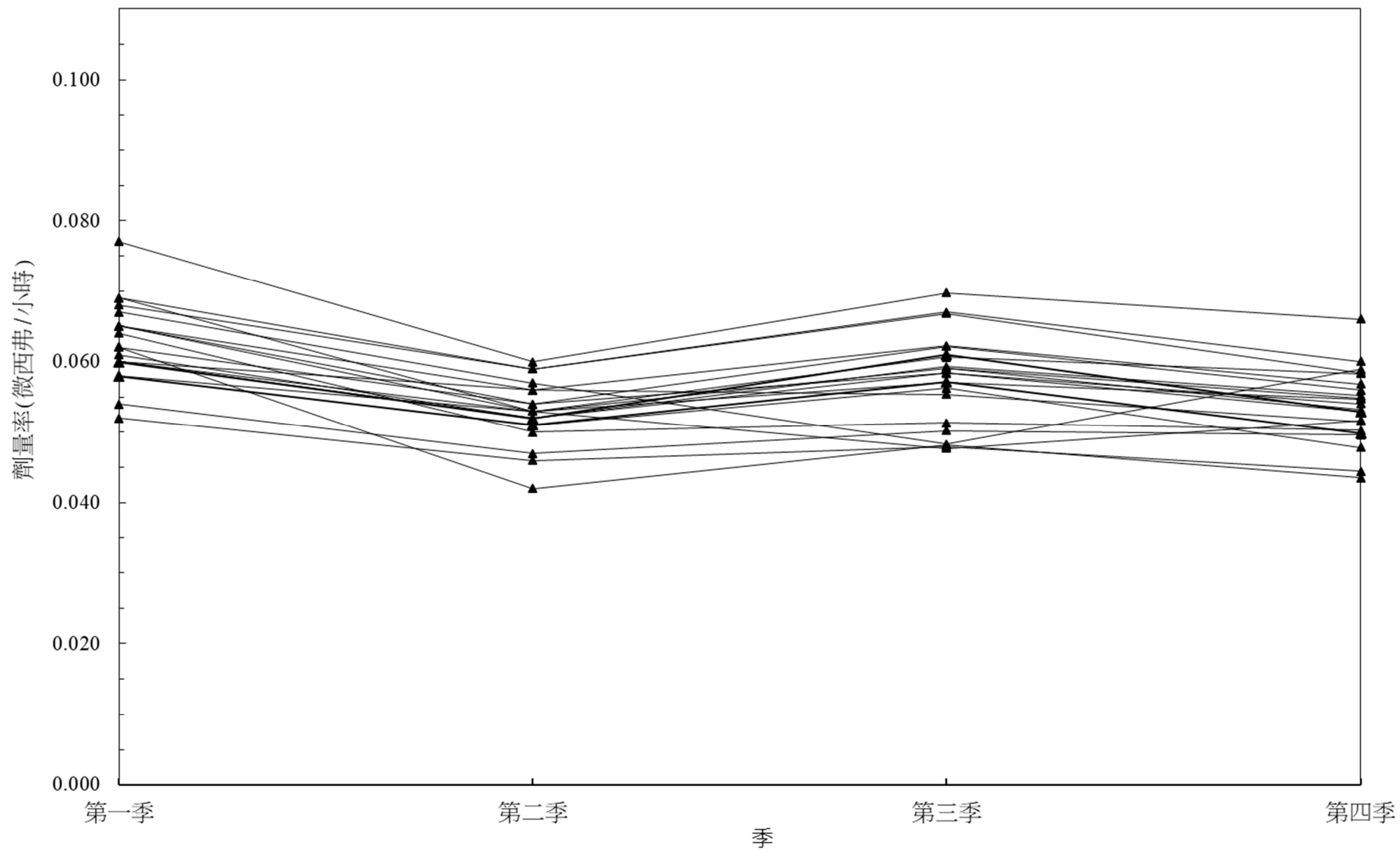
圖2 111年熱發光劑量計偵測站劑量率變動圖
