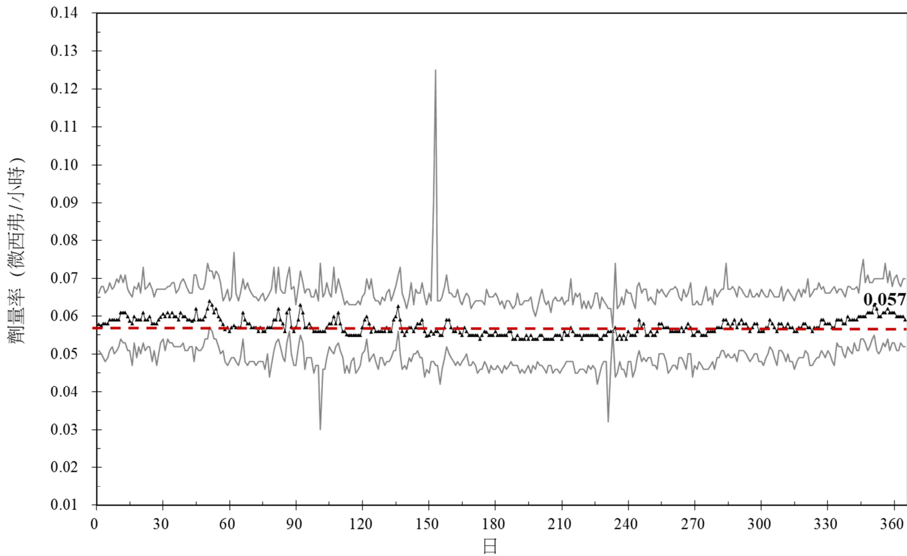
圖5 111年連續輻射偵測劑量率變動圖(加速器館)
