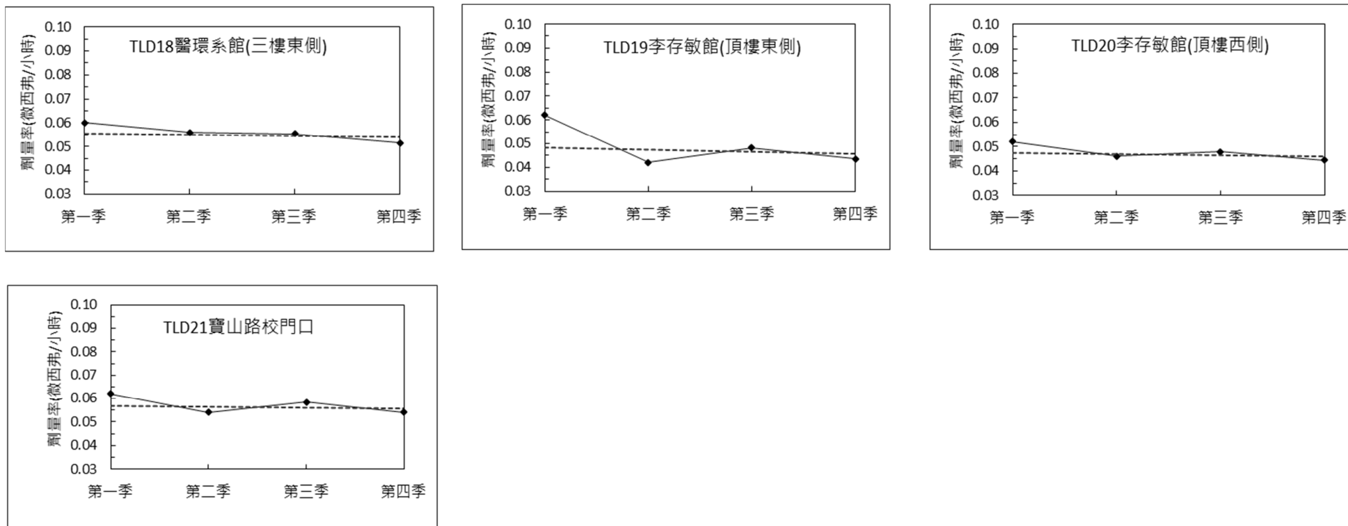
圖3 111年熱發光劑量計各偵測站劑量率變動圖
