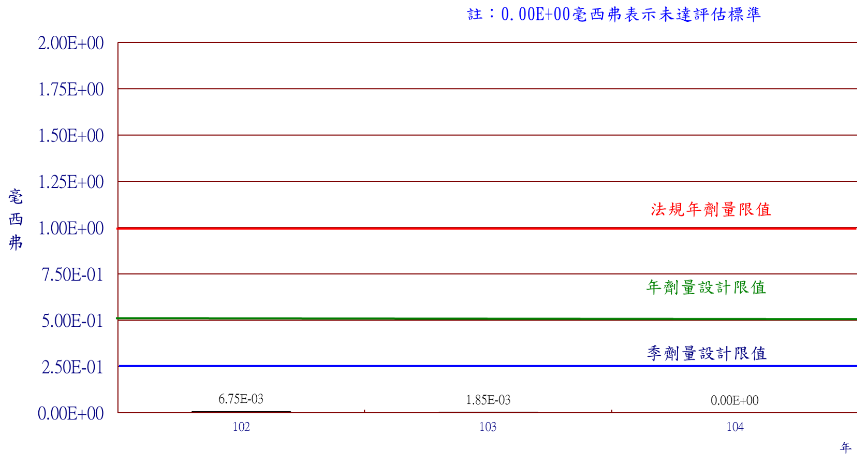
圖18 核能一廠104年民眾最大個人全身劑量
