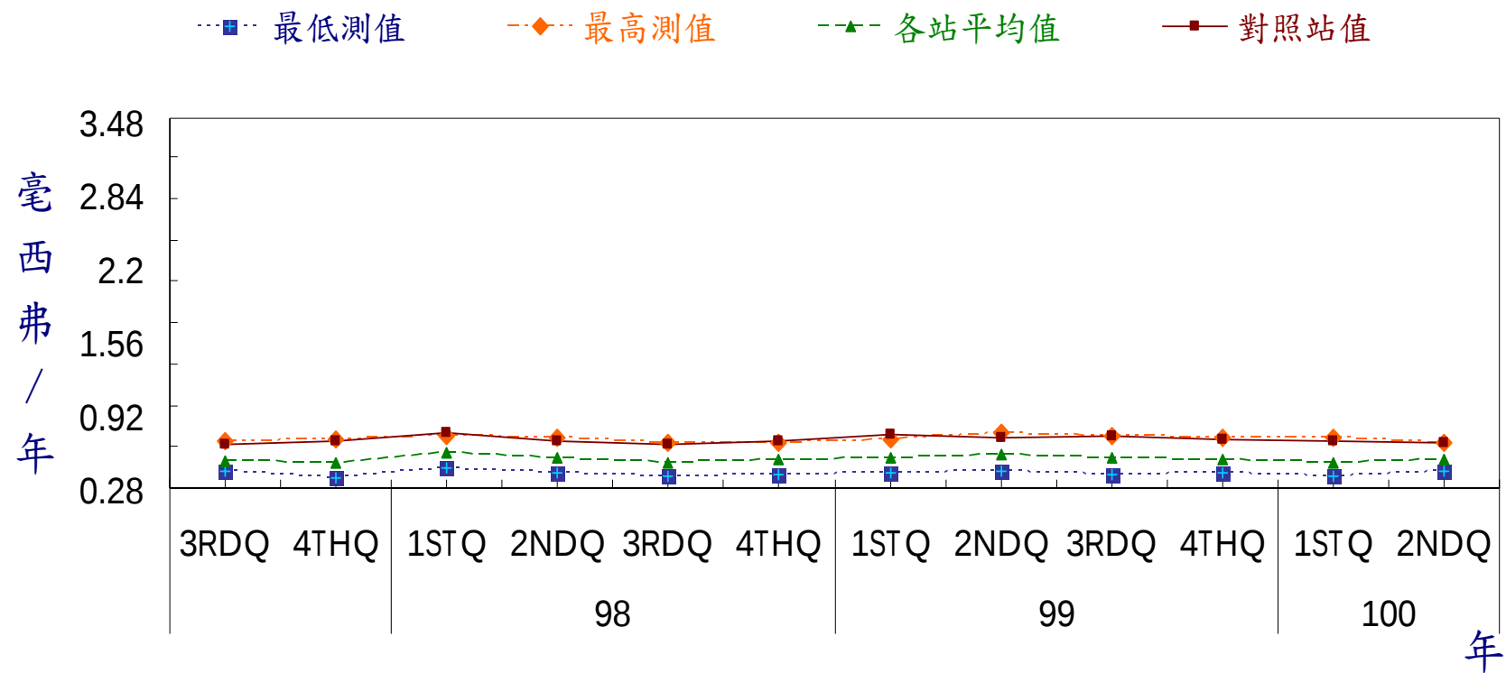
圖 14 核能一廠環境熱發光劑量計監測結果
