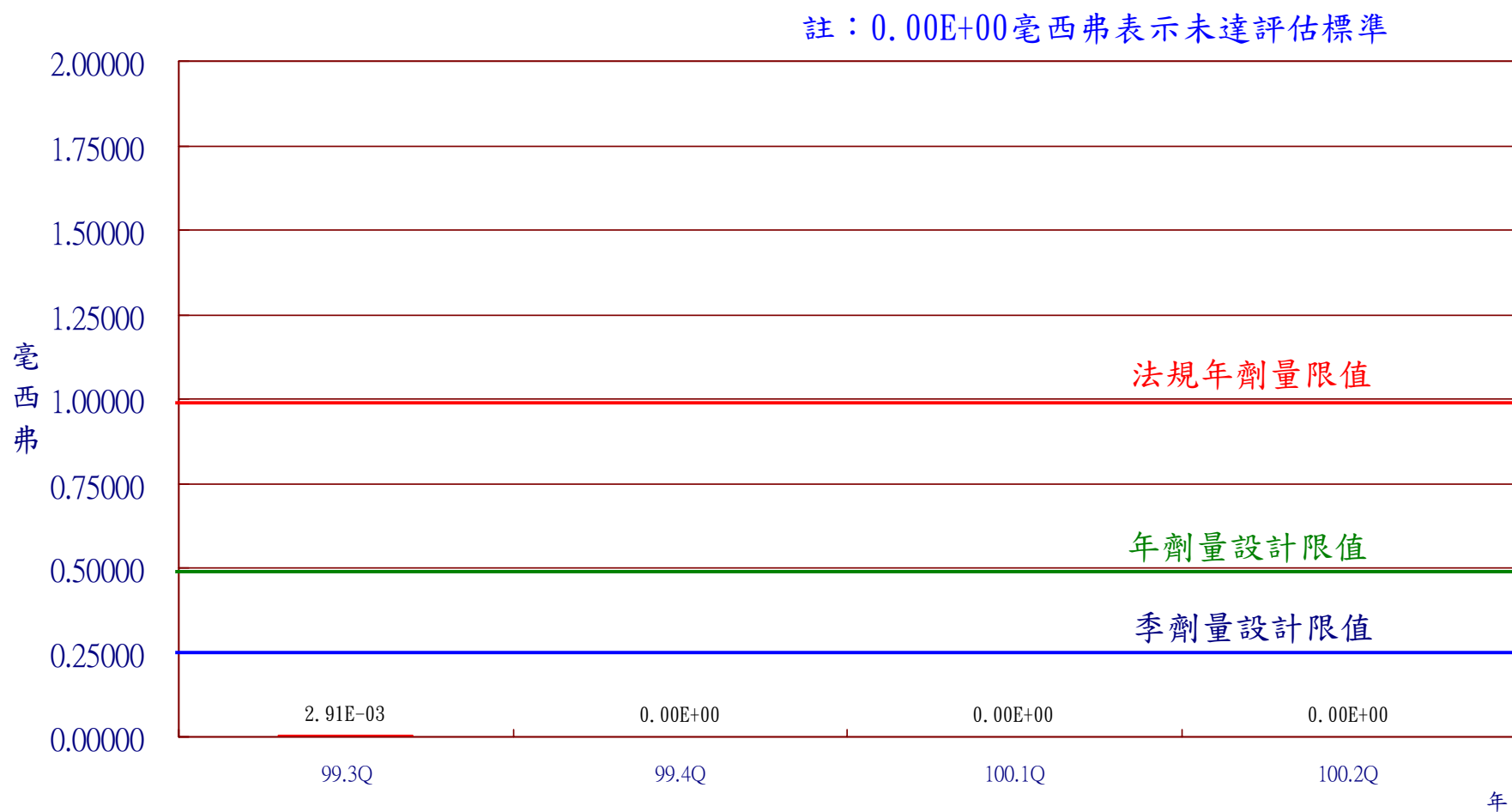
圖18 核能一廠100年第2季民眾最大個人全身劑量
