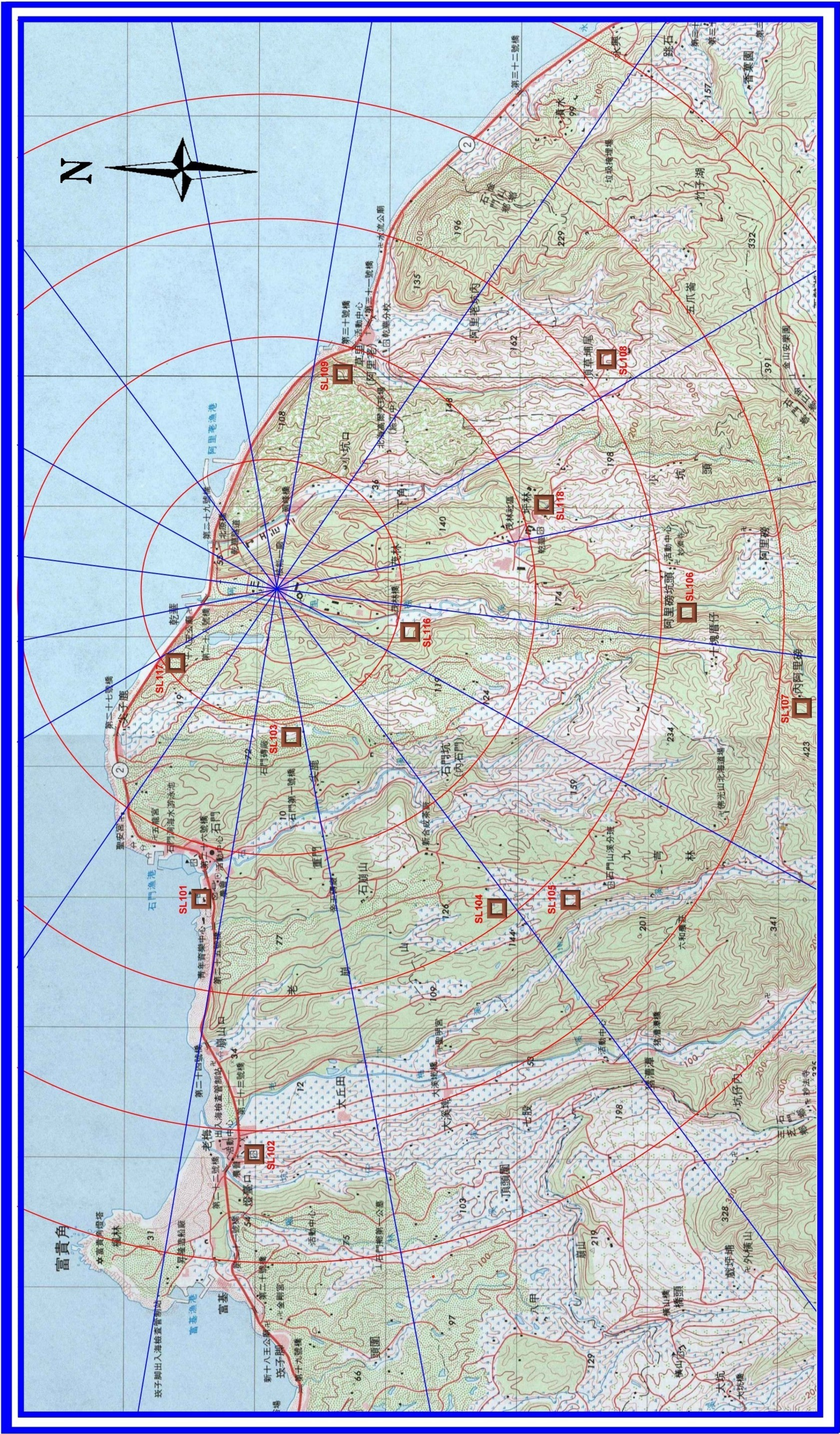
圖10 核能一廠土壤取樣站分佈圖(5公里內)
