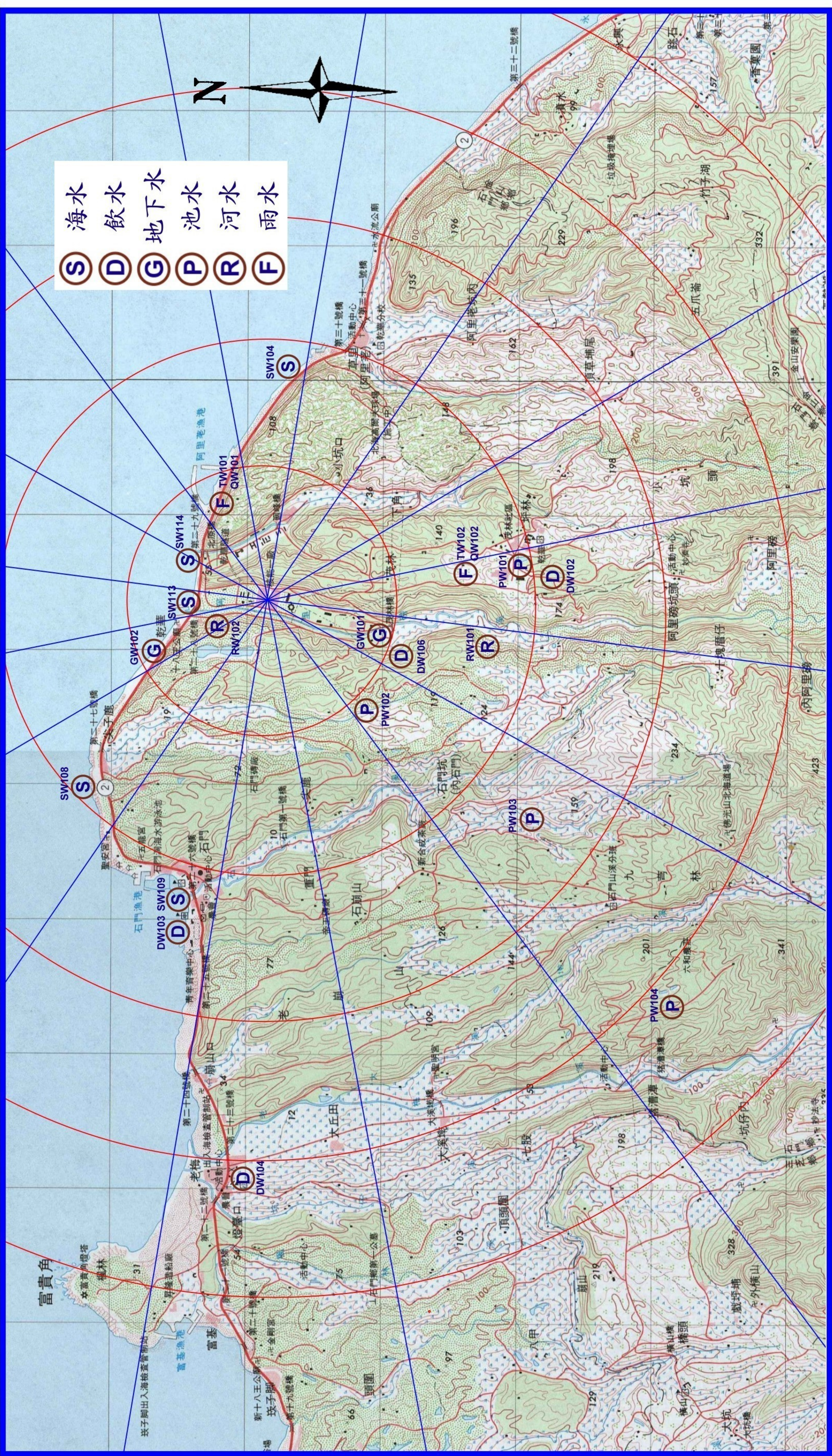
圖6 核能一廠各類水樣取樣站分佈圖(5公里內)
