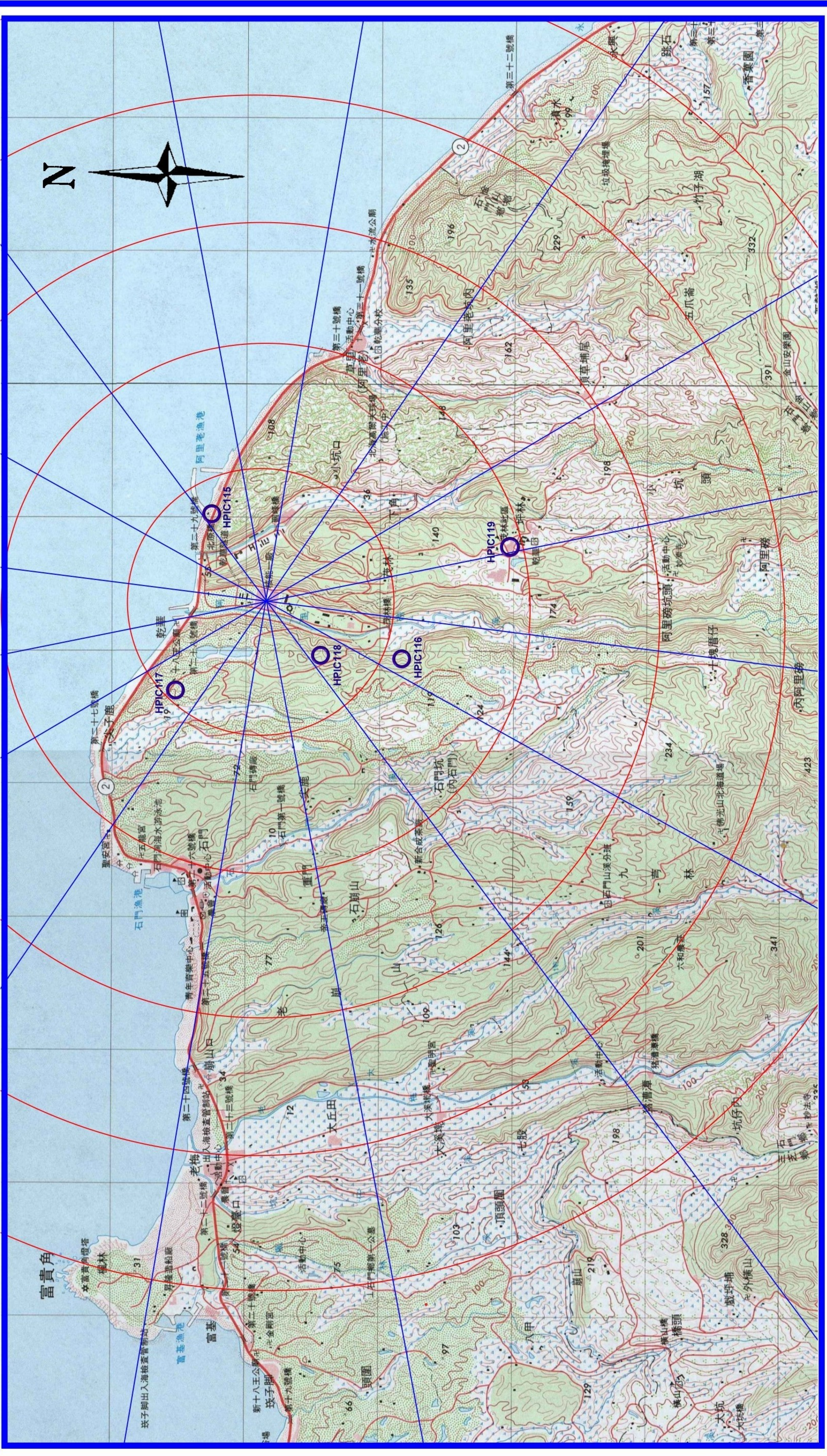
圖3 核能一廠高壓游離腔監測站分佈圖
