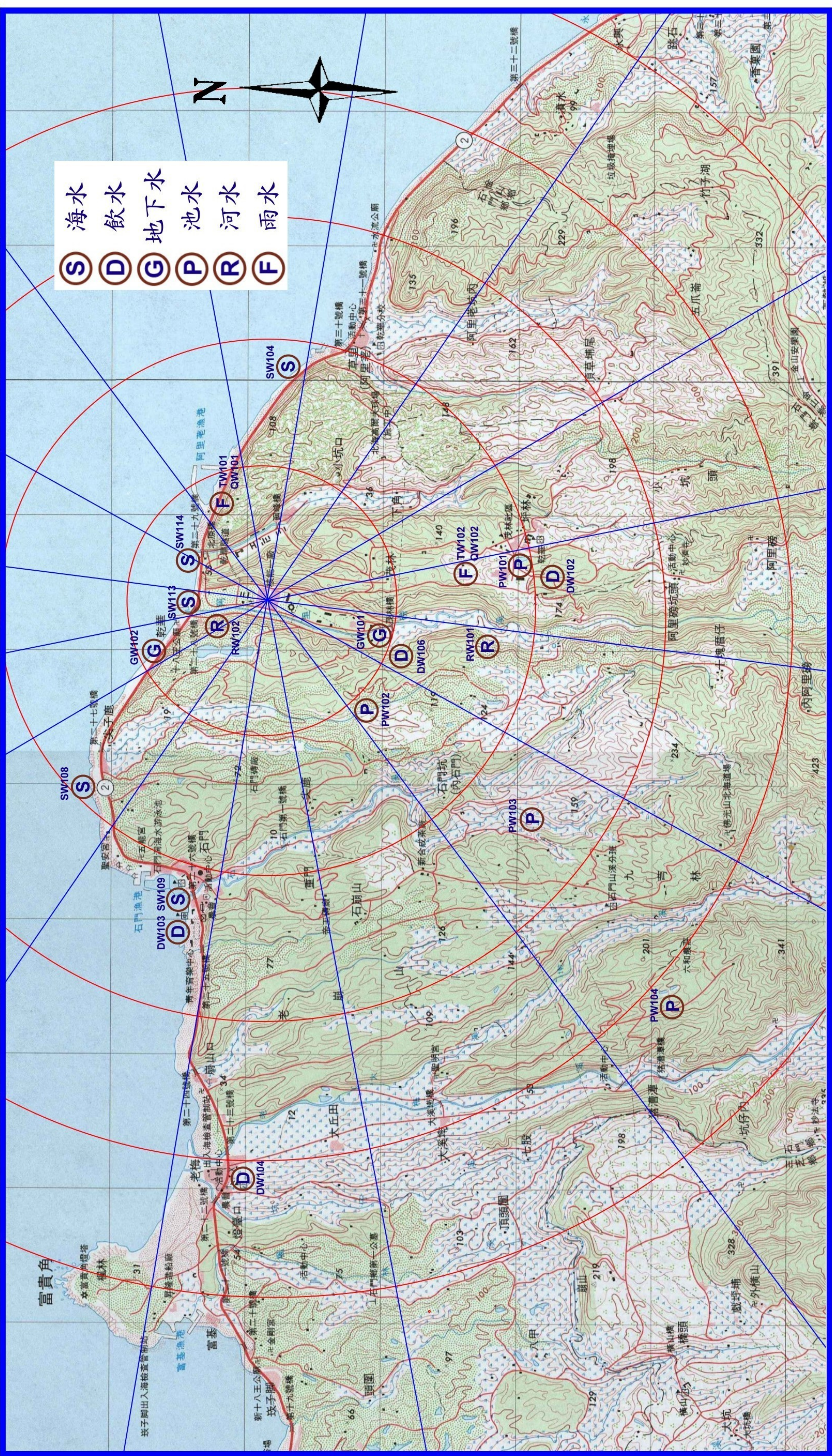
圖6 核能一廠各類水樣取樣站分佈圖(五公里內)
