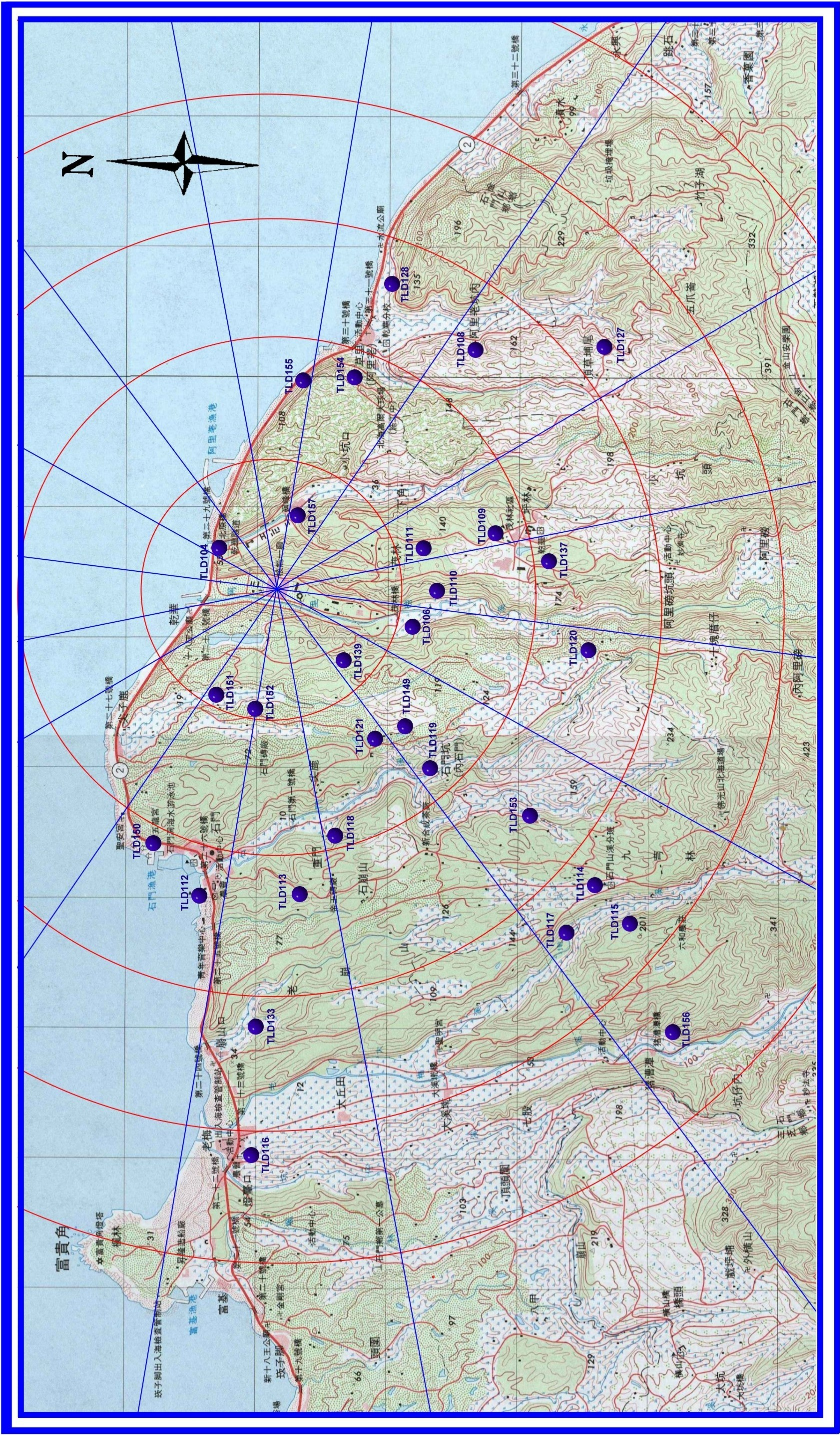
圖1 核能一廠熱發光劑量計監測站分佈圖(五公里內)
