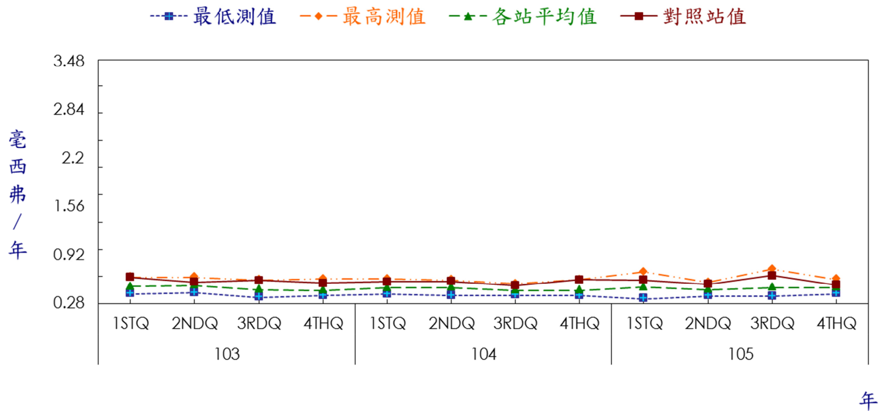
圖14 核能三廠環境熱發光劑量計監測結果
