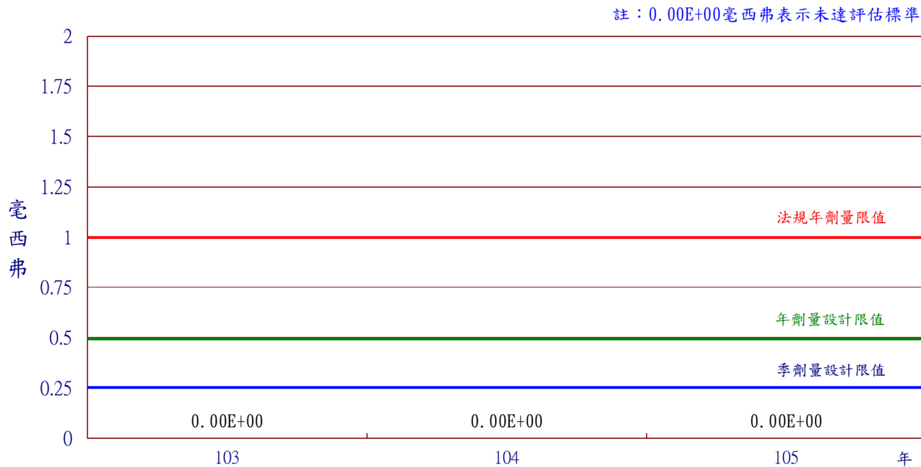
圖17 核能三廠105年民眾最大個人全身劑量
