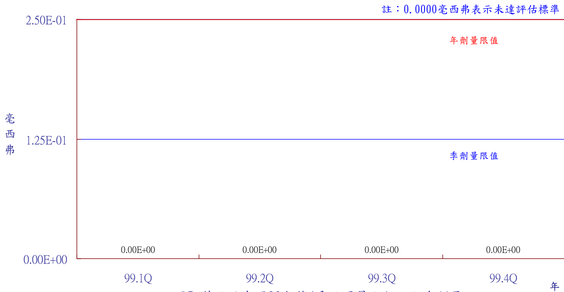
圖5 蘭嶼貯存場99年第4季民眾最大個人全身劑量
