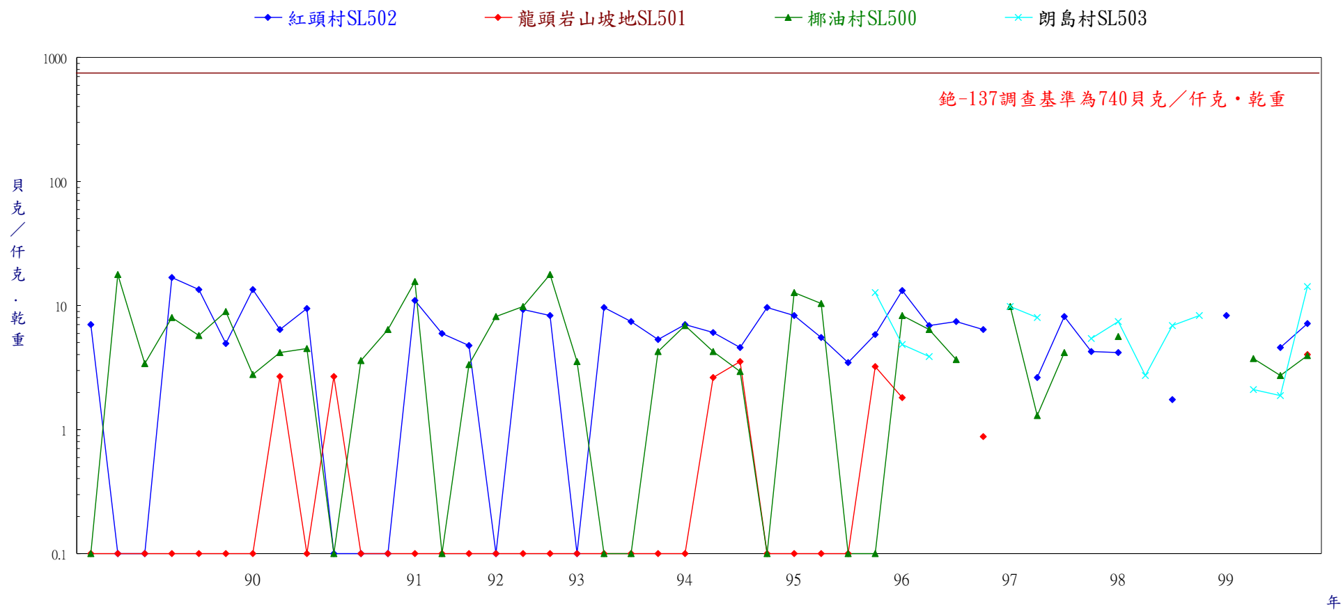
圖3 蘭嶼貯存場土壤鉅-137加馬能譜分析結果
