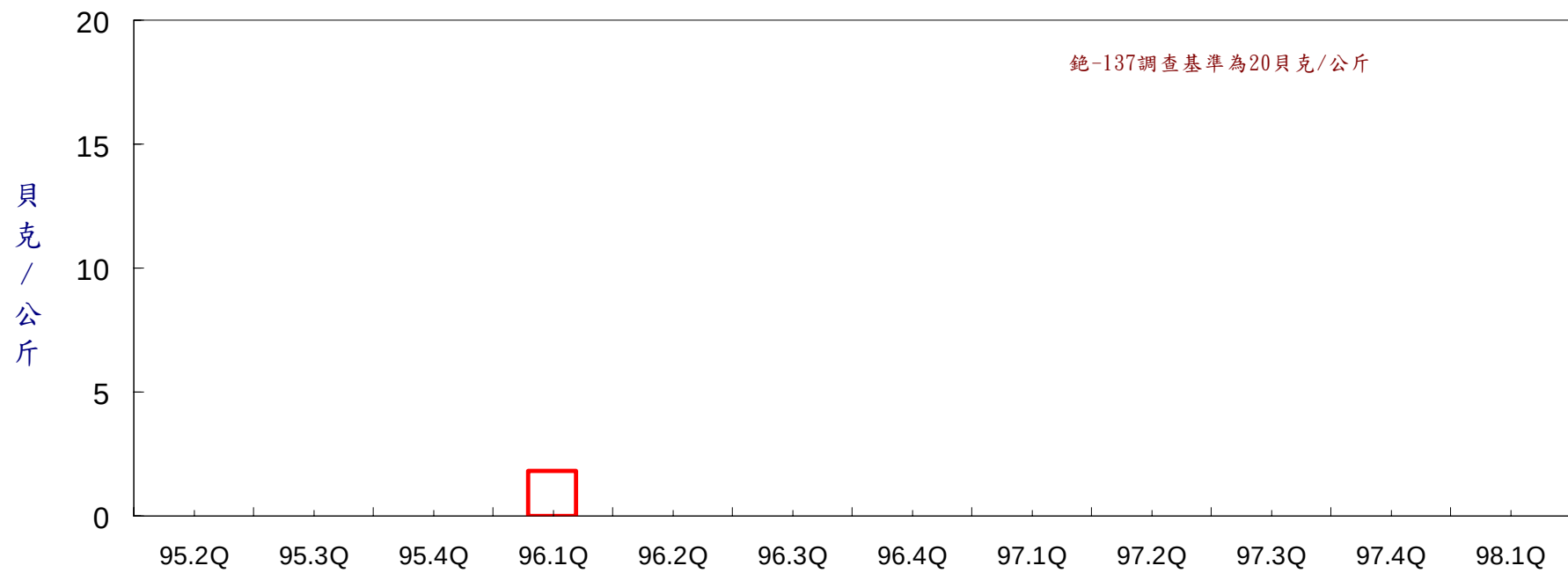
圖 17 核能一廠出水口岸沙加馬能譜監測結果
