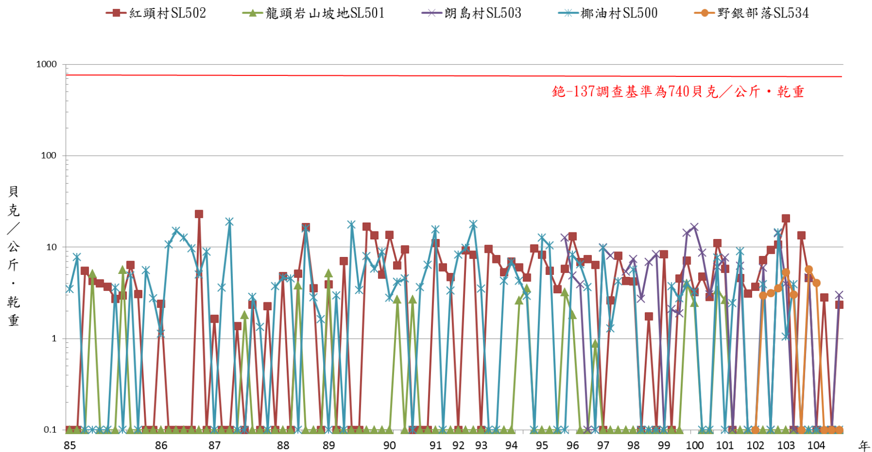
圖3 蘭嶼貯存場土壤鉅-137加馬能譜分析結果
