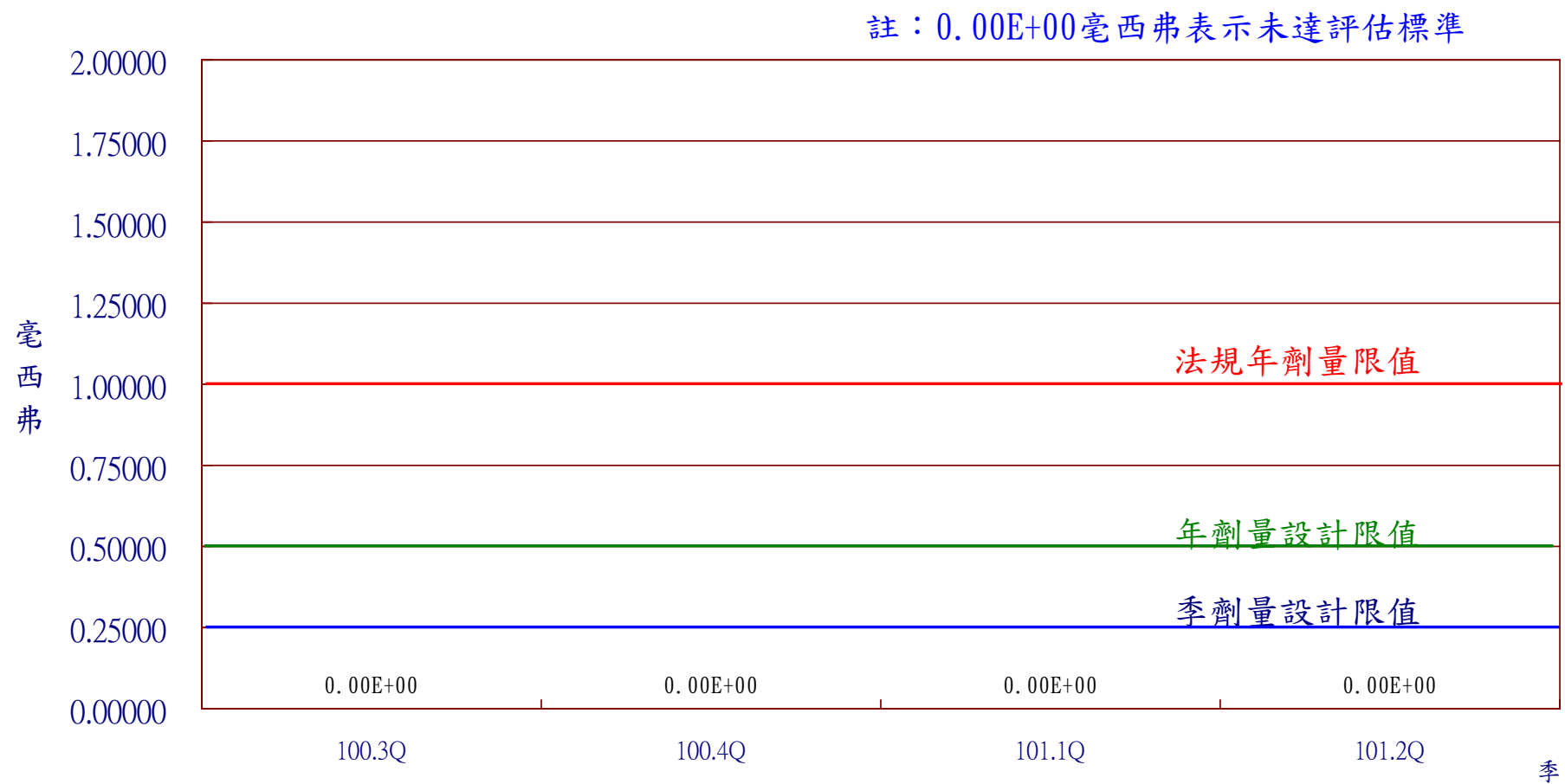
圖16 核能二廠101年第2季民眾最大個人全身劑量
