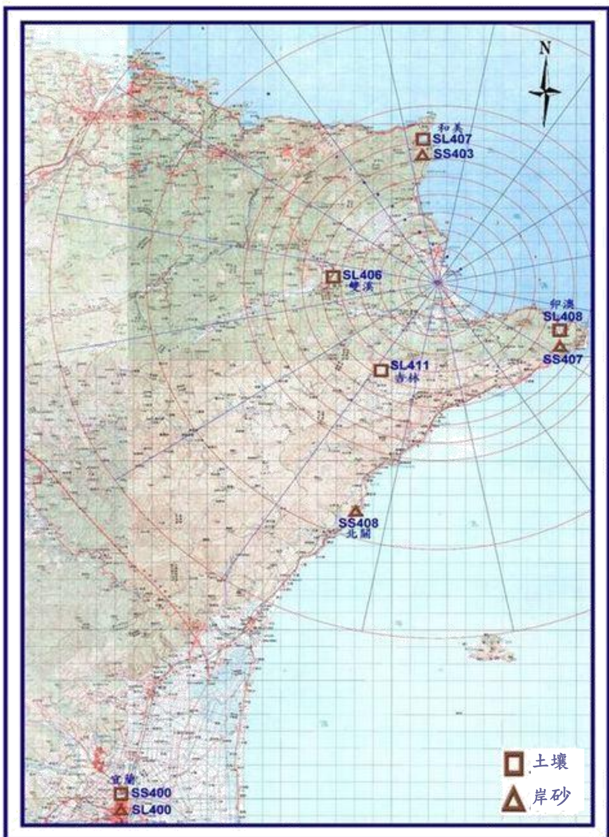
圖 11 核能四廠沉積物試樣取樣站分佈圖(5 公里外)
