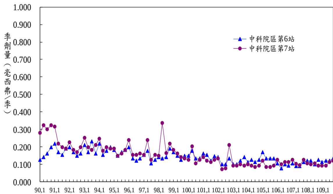
圖 3-1-2：中科院區第 6，7 站 TLD 季輻射劑量變化趨勢圖
