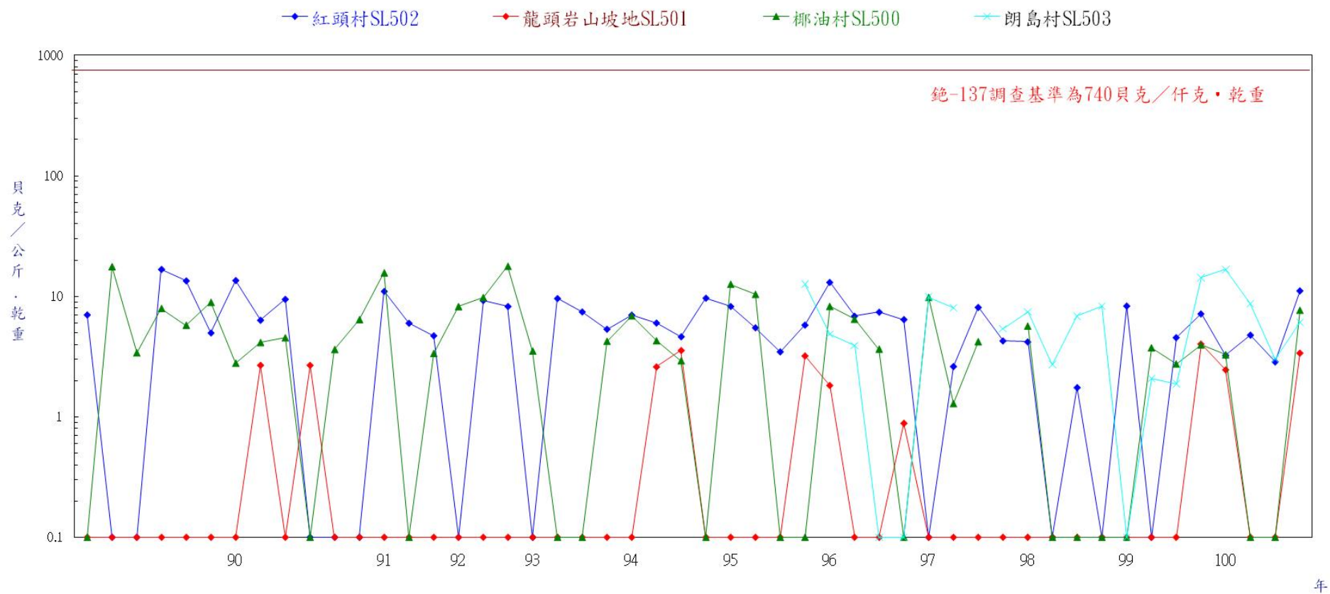
圖3 蘭嶼貯存場土壤鉈-137加馬能譜分析結果
