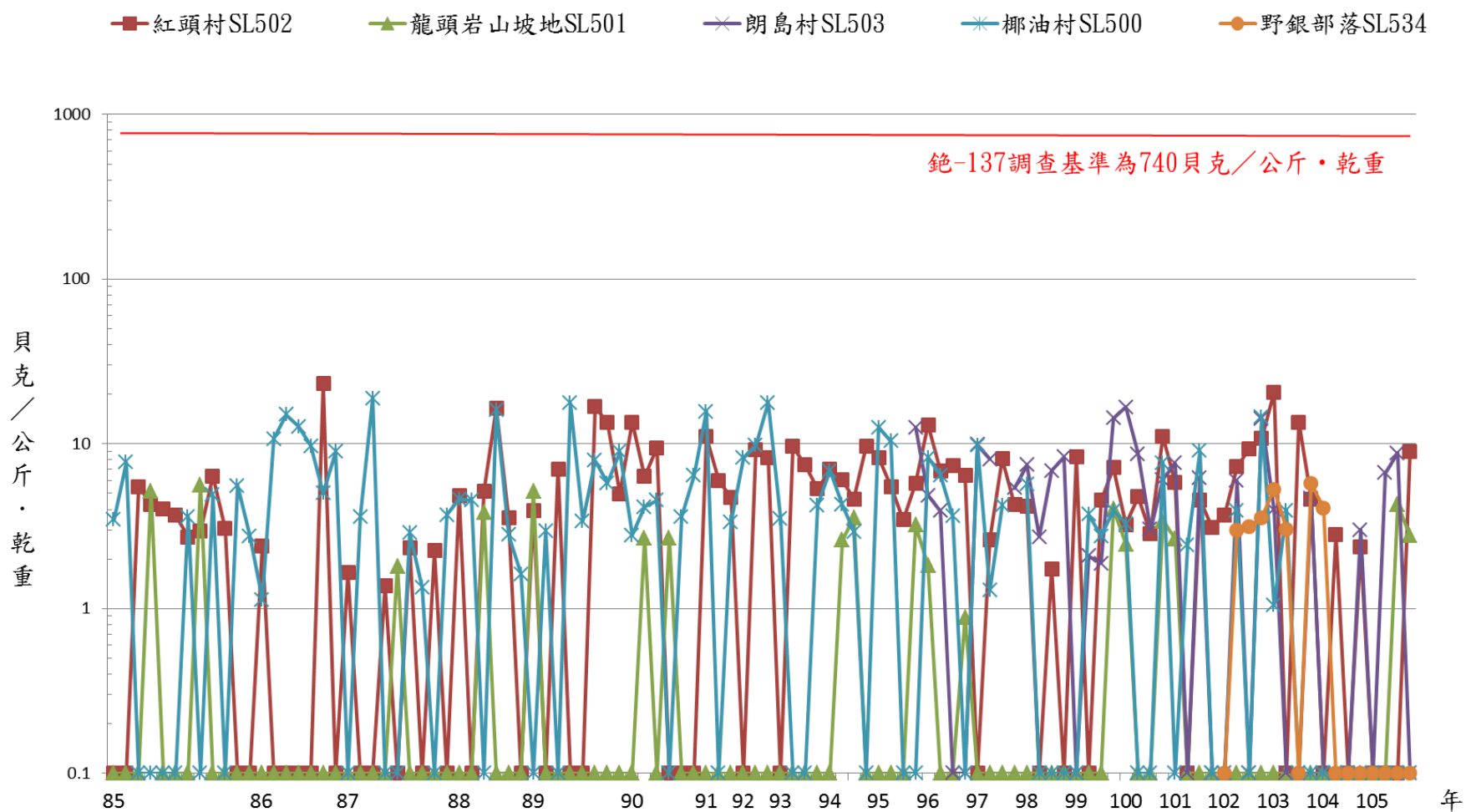
圖3 蘭嶼貯存場土壤鈉-137加馬能譜分析結果
