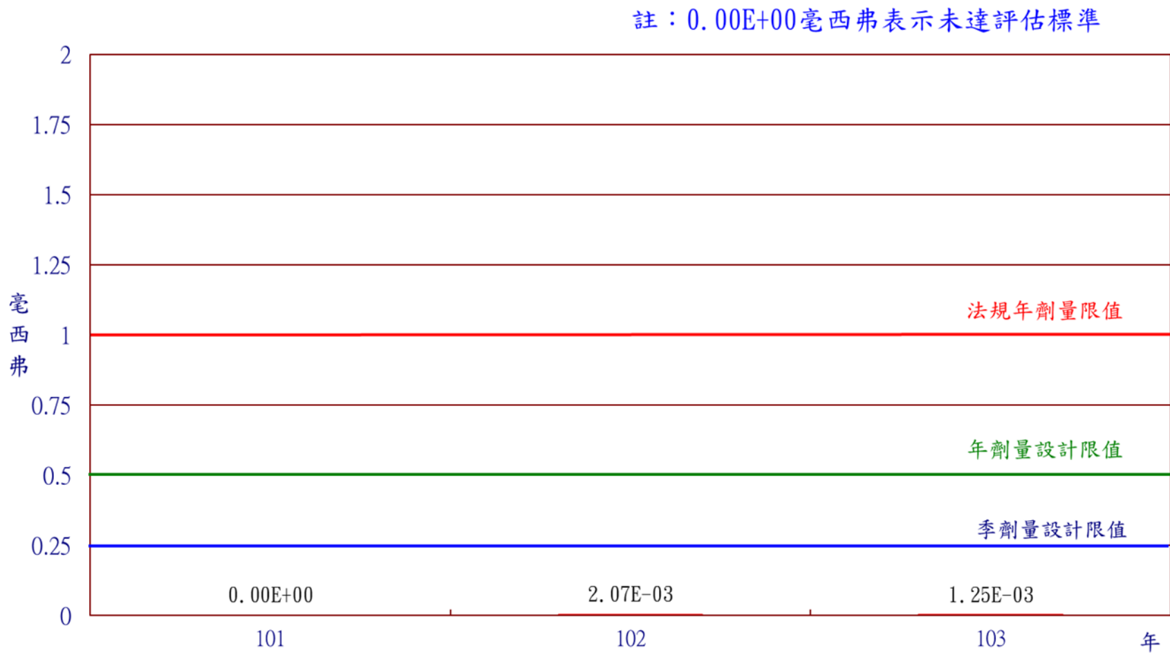
圖16 核能二廠103年民眾最大個人全身劑量
