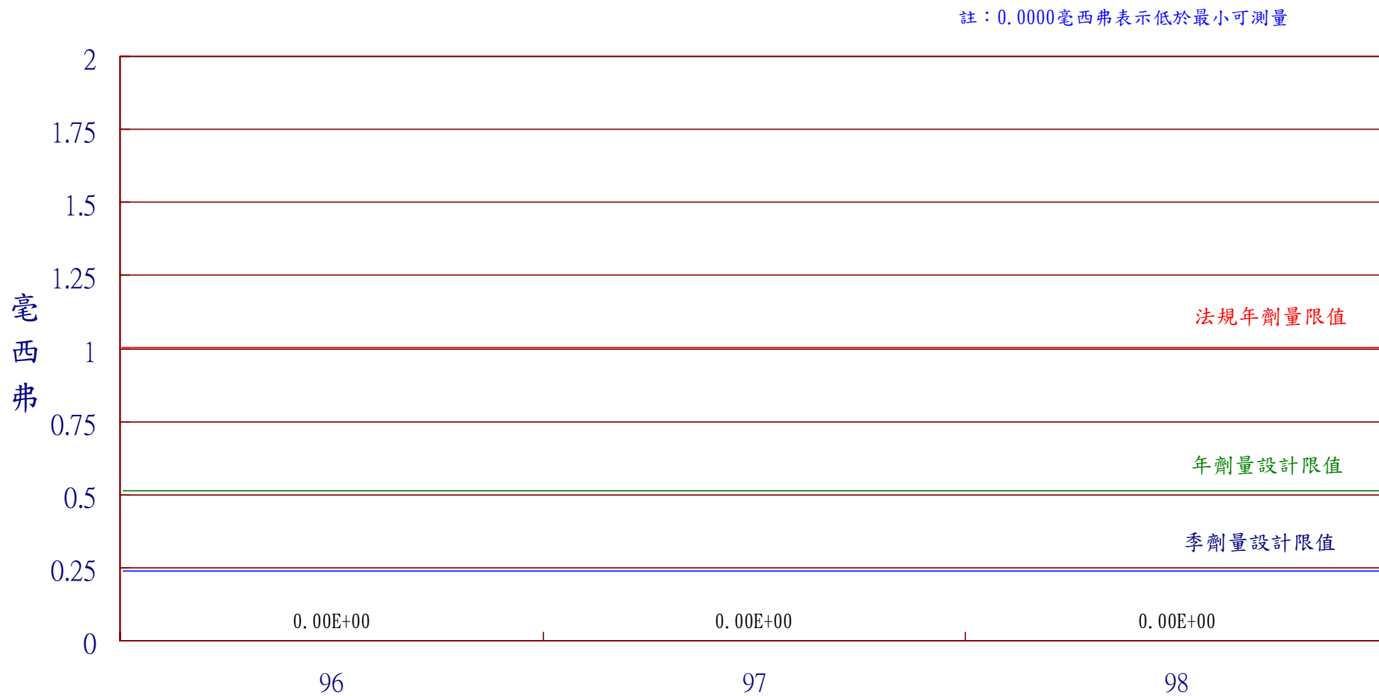
圖17 核能三廠98年民眾最大個人全身劑量 年
