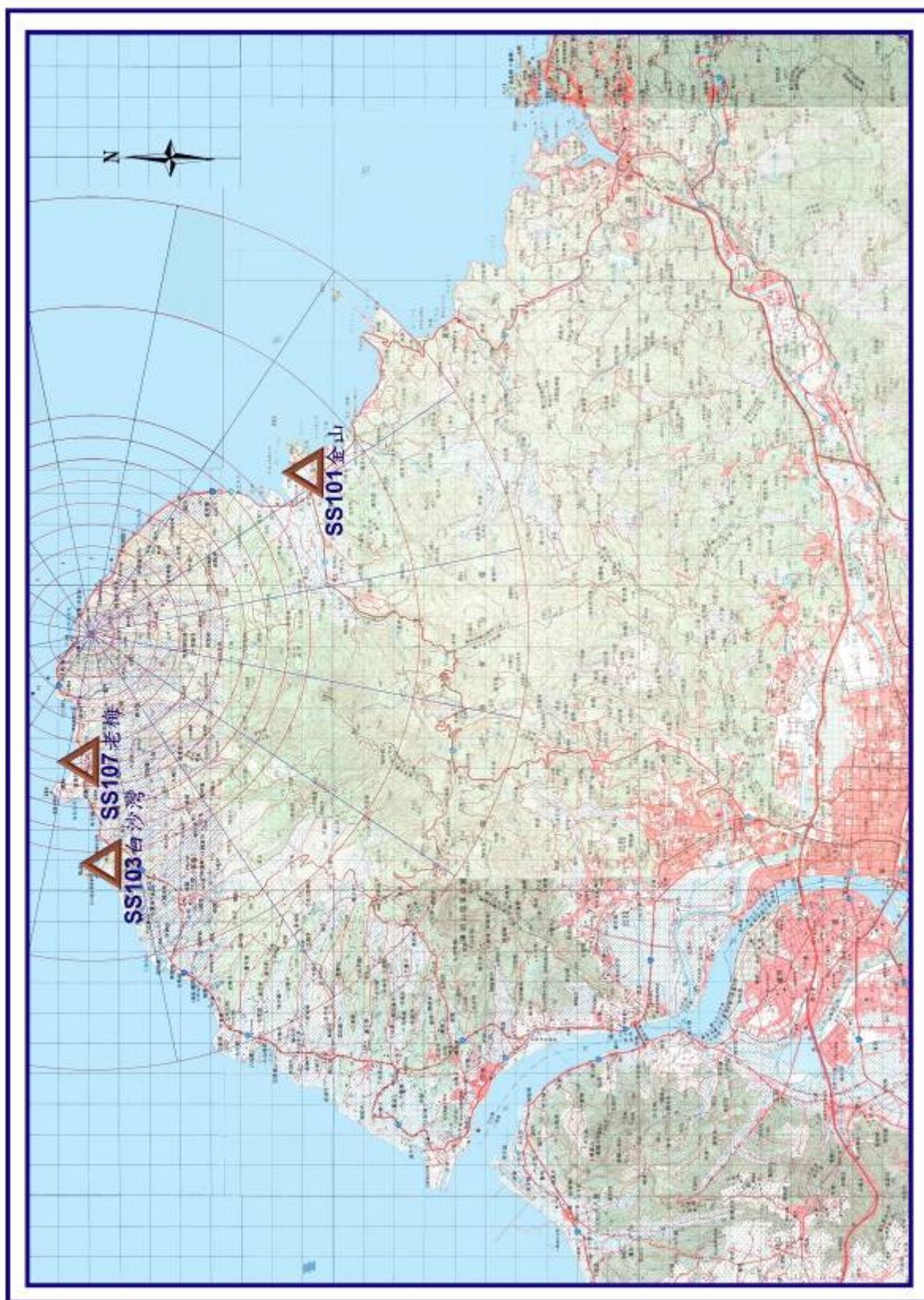
圖12 核能一廠岸砂取樣站分佈圖(5公里外)
