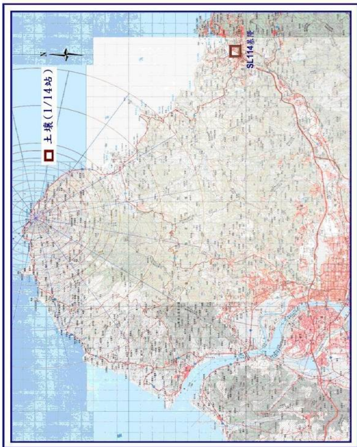
圖10 核能一廠土壤取樣站分佈圖(5公里外)
