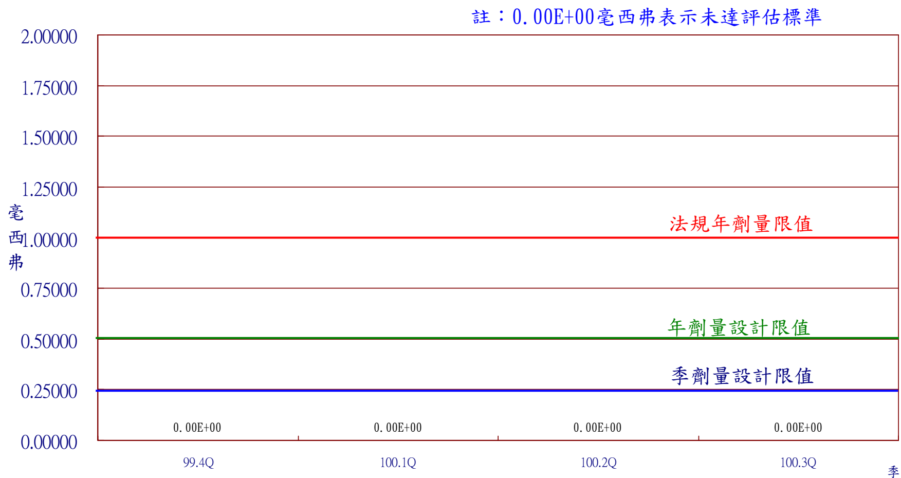
圖18 核能一廠100年第3季民眾最大個人全身劑量
