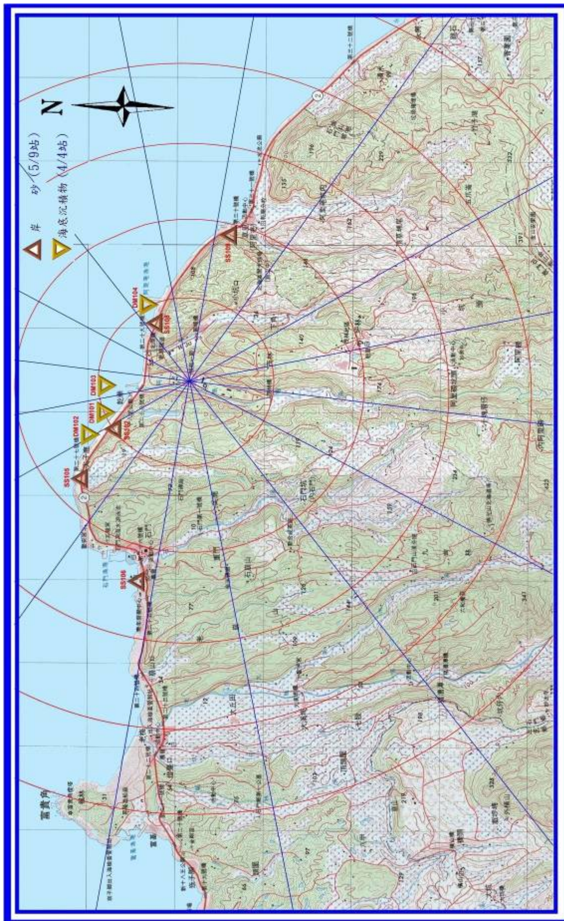
圖11 核能一廠岸砂取樣站分佈圖(5公里內)
