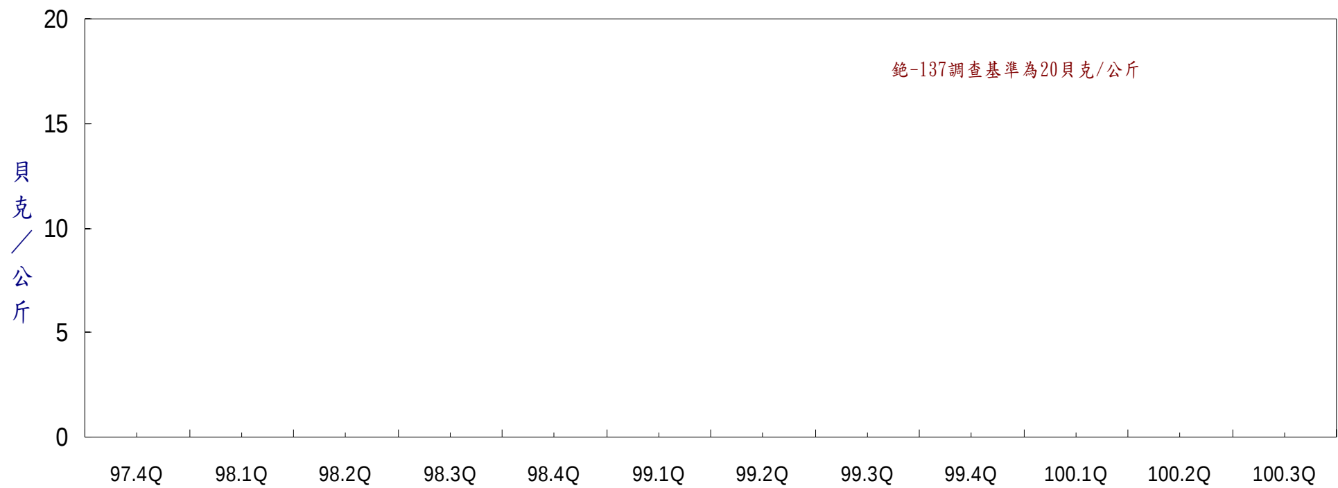
圖 17 核能一廠出水口岸砂加馬能譜監測結果
