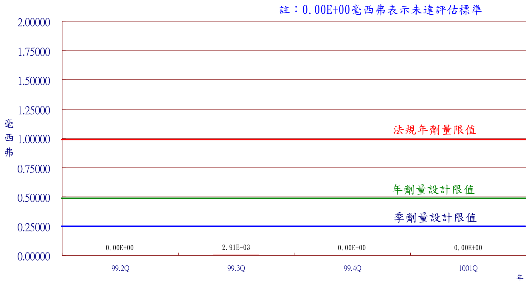
圖18 核能一廠100年第1季民眾最大個人全身劑量
