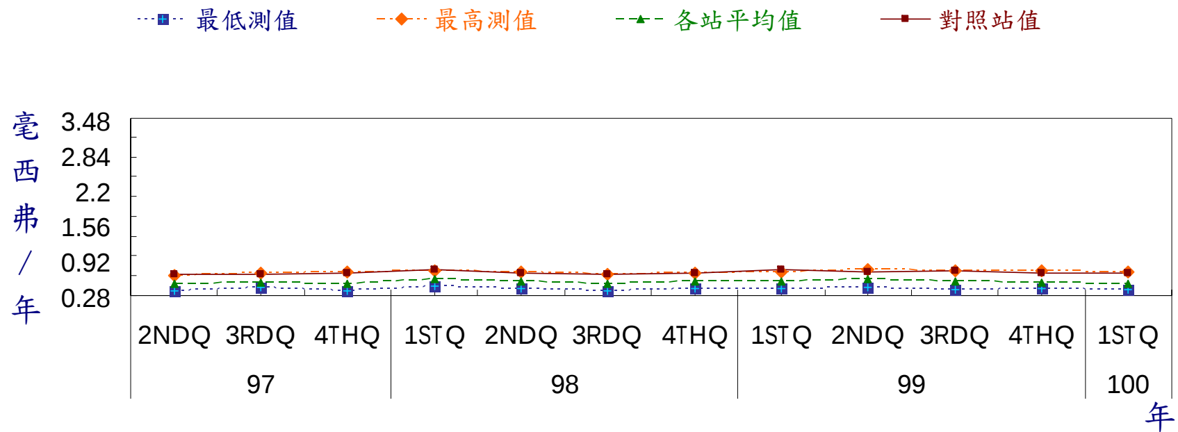
圖 14 核能一廠環境熱發光劑量計監測結果
