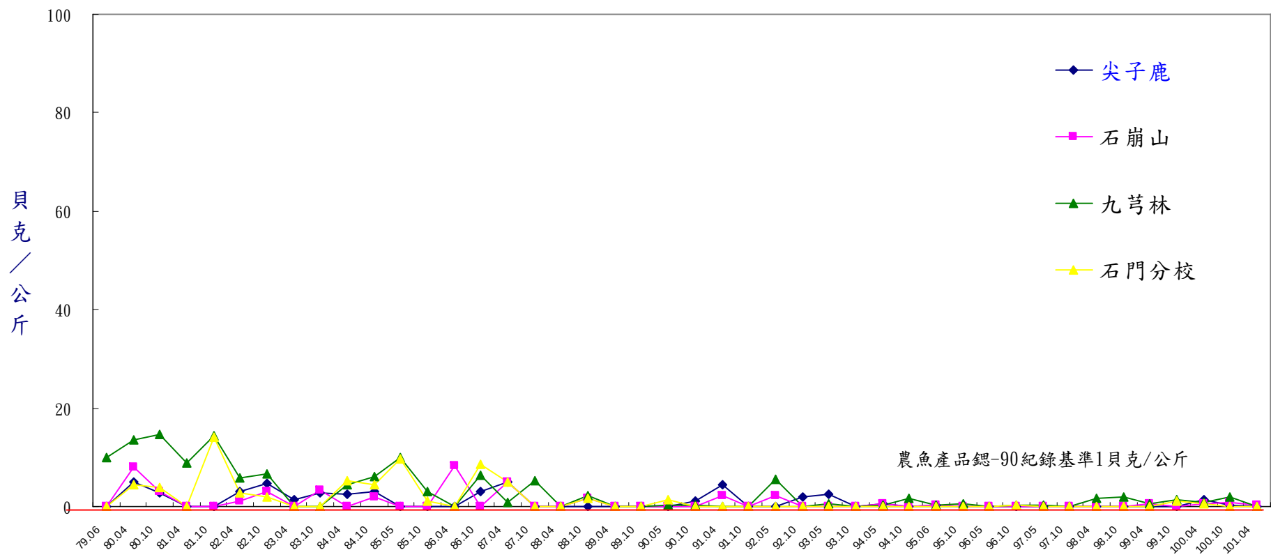
圖16 核能一廠茶葉 90 Sr活度歷年分析結果
