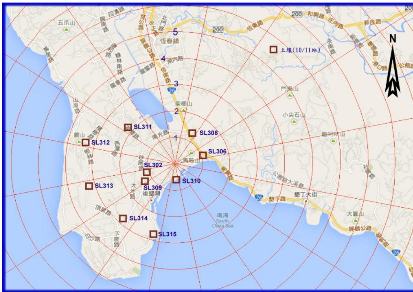
圖 9 核能三廠土壤取樣站分佈圖(5 公里內)
