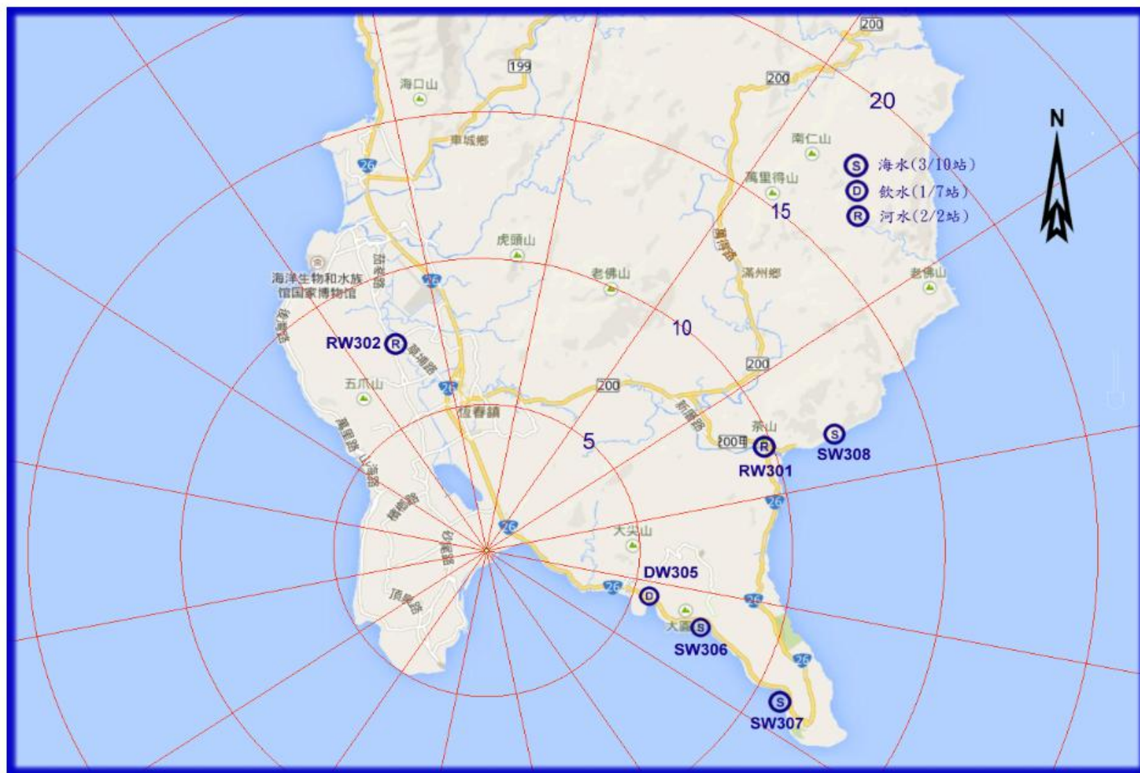
圖 6 核能三廠各類水樣取樣站分佈圖(5 公里外)
