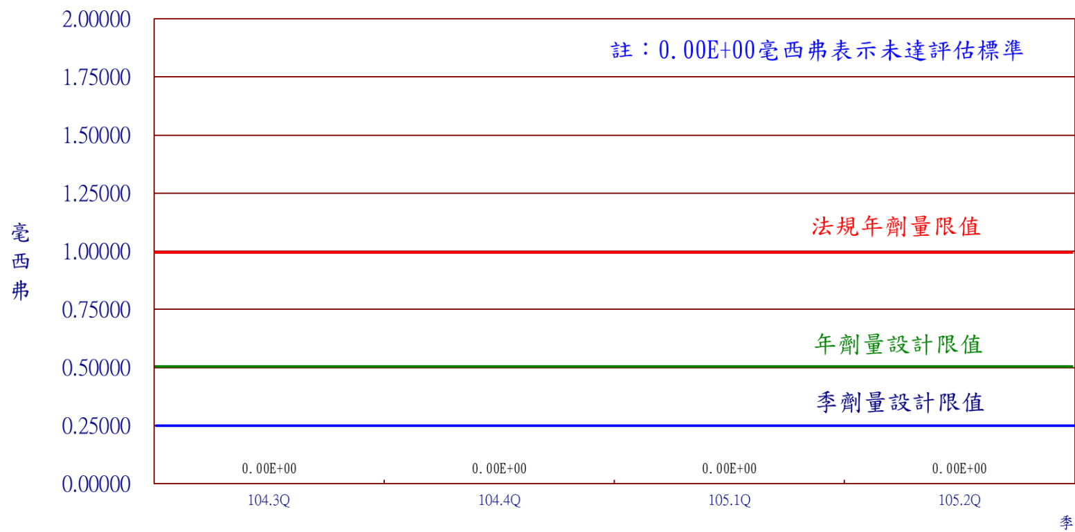
圖18 核能一廠105年第2季民眾最大個人全身劑量
