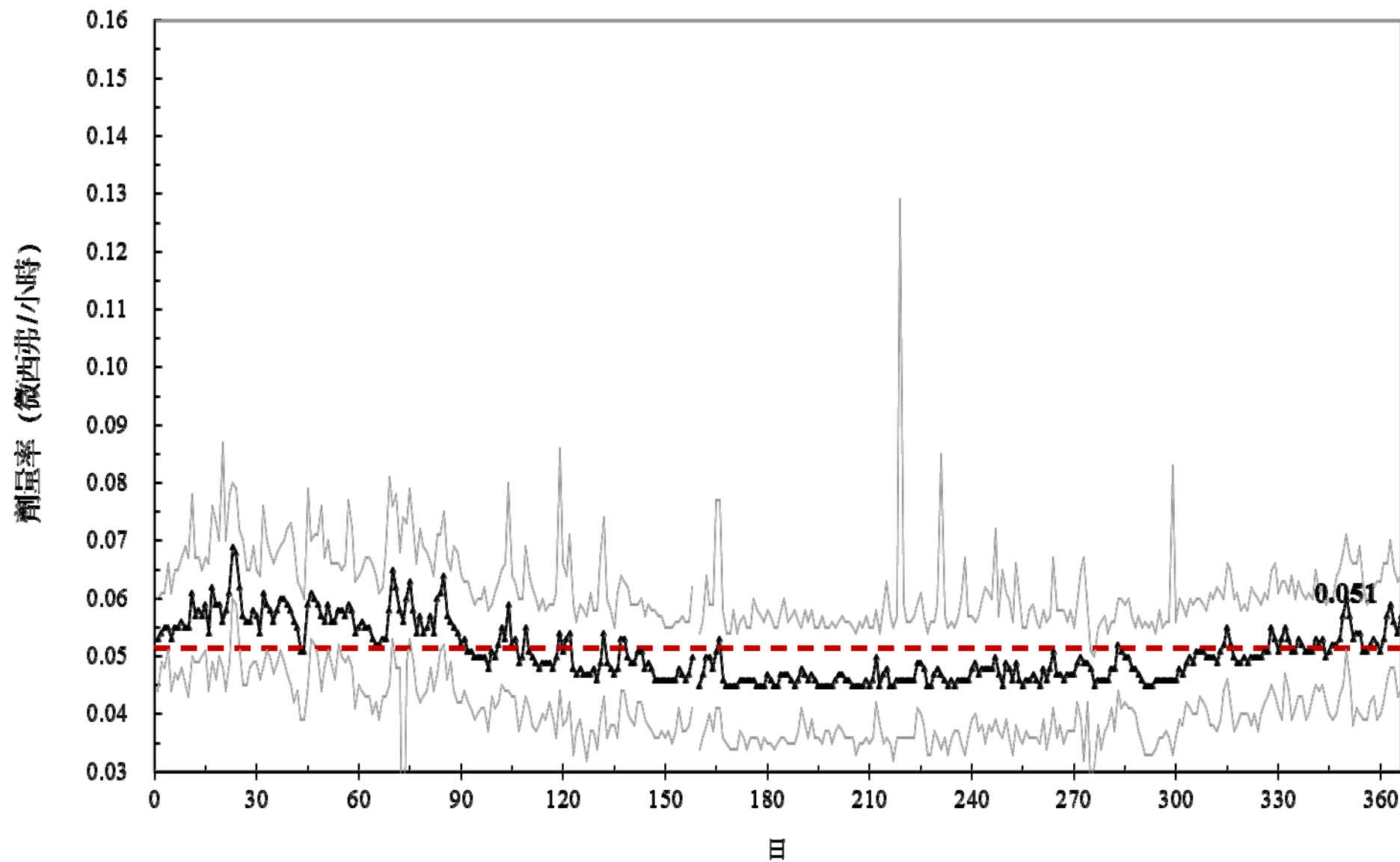
圖 4 105 年連續輻射偵測劑量率變動圖(生物科技館)
