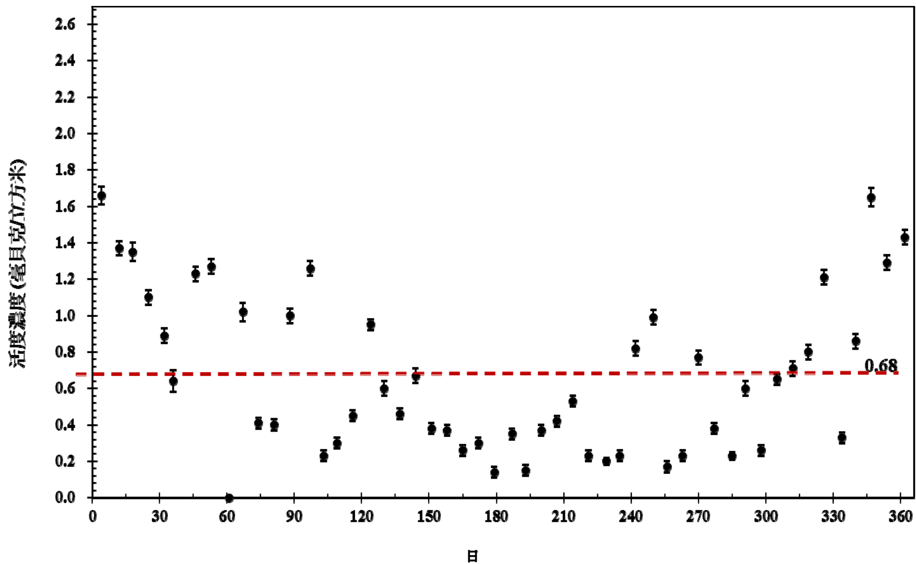
圖7 105年空浮微粒活度濃度變動圖(速器館側)
