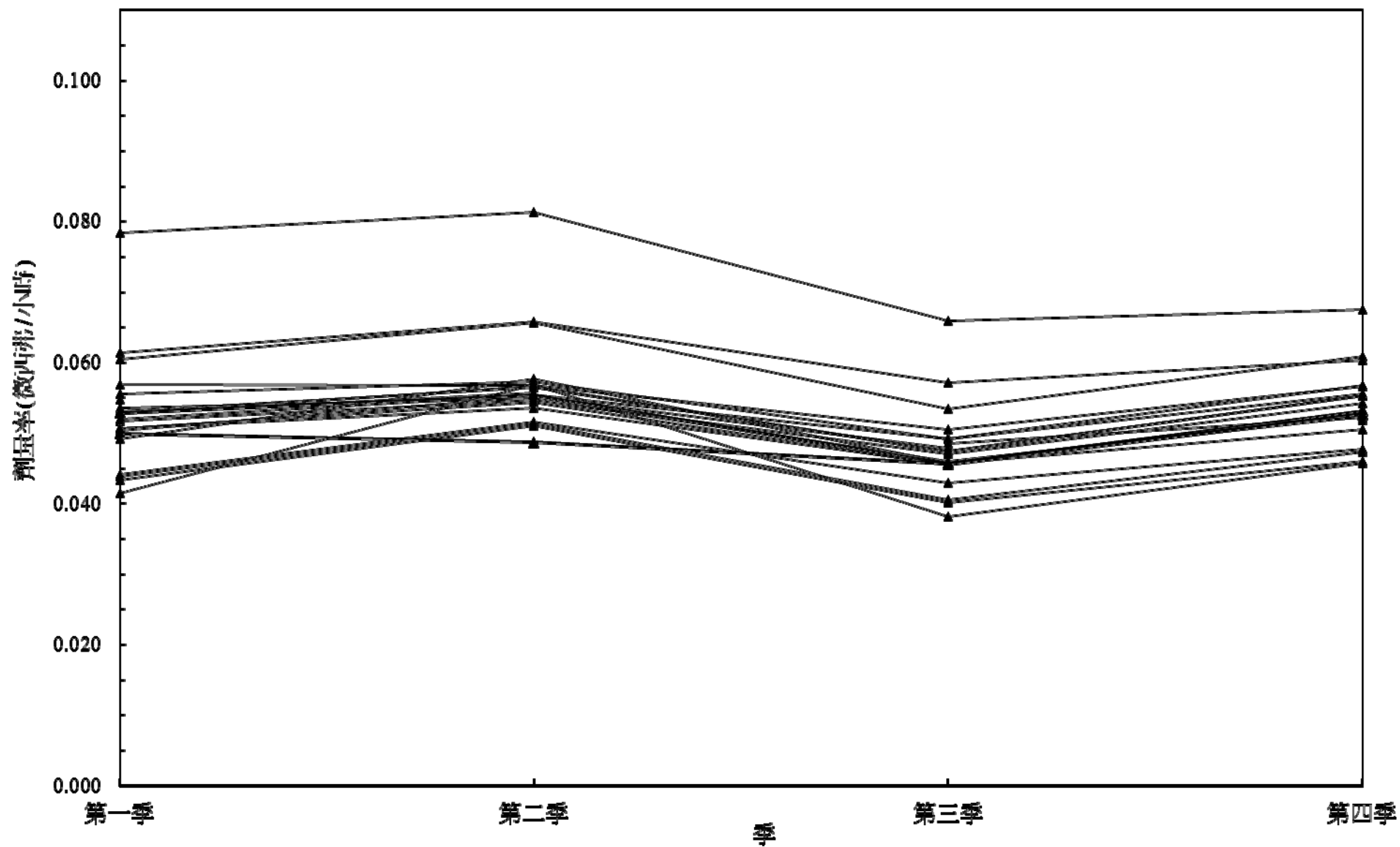
圖2 105年熱發光劑量計偵測站劑量率變動圖
