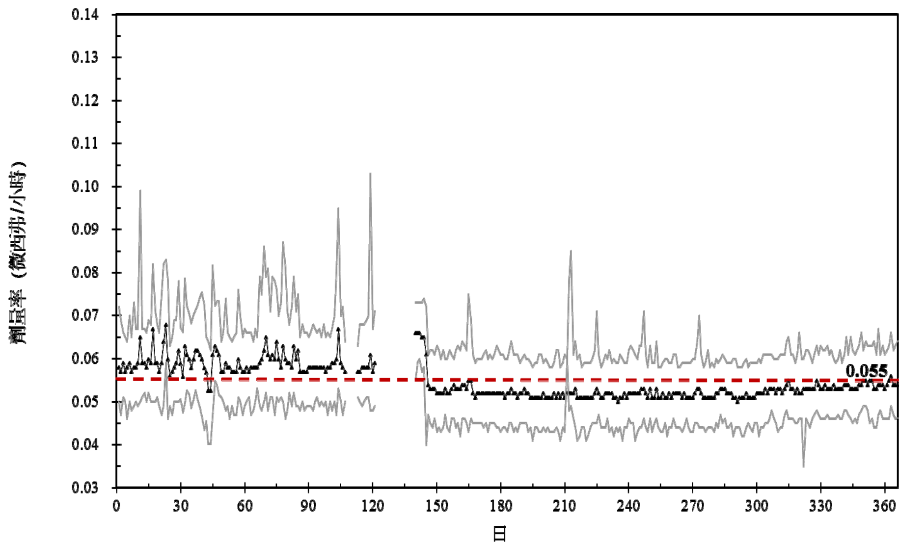
圖5 105年連續輻射偵測劑量率變動圖(加速器館側)
