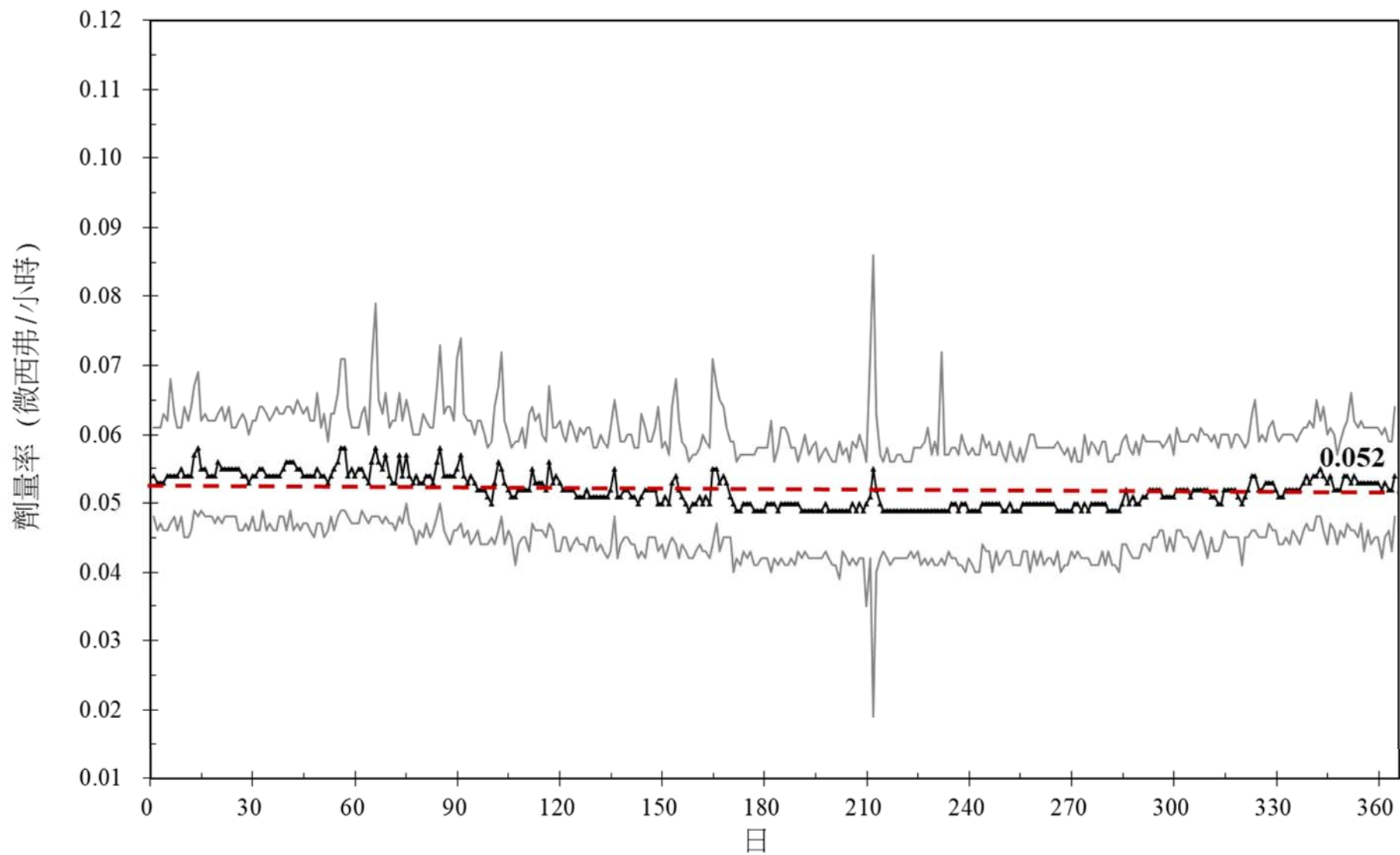
圖5 106年連續輻射偵測劑量率變動圖(加速器館)
