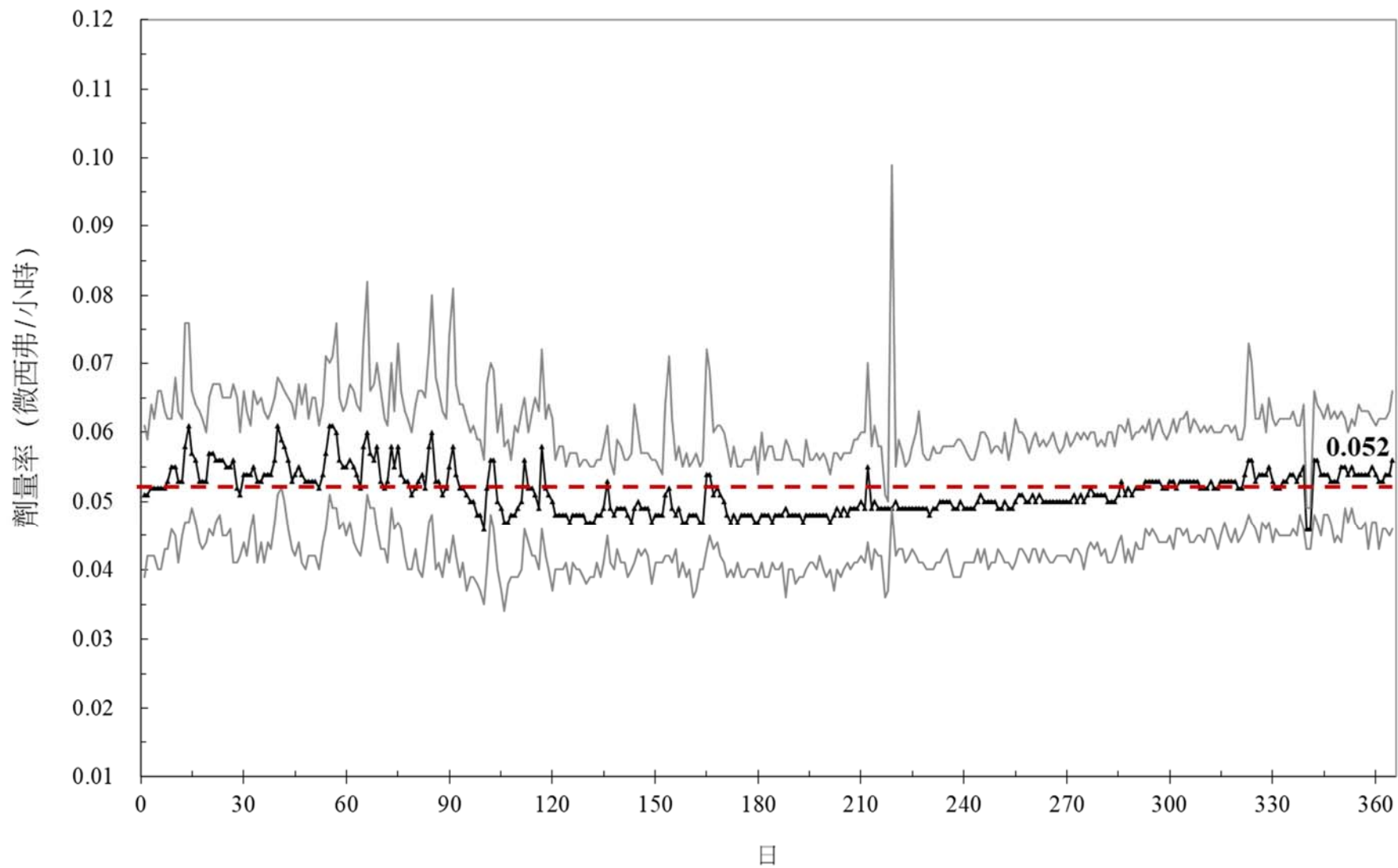
圖 4 106 年連續輻射偵測劑量率變動圖(生物科技館/李存敏館)
