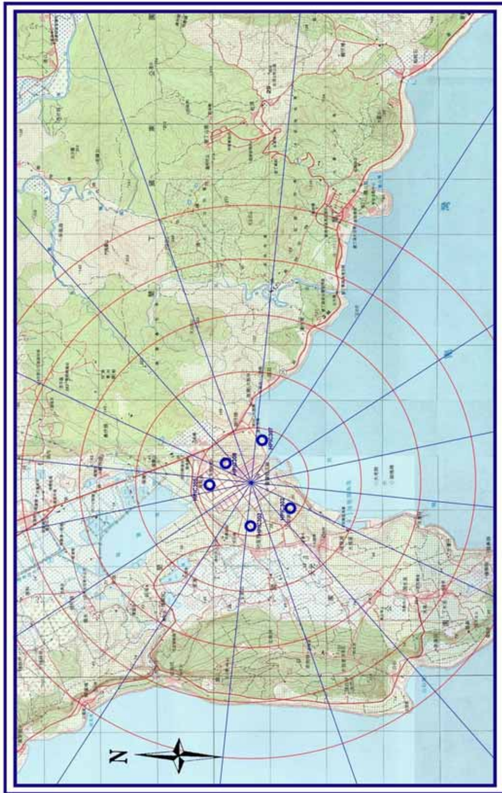
圖3 核能三廠高壓游離腔監測站分佈圖
