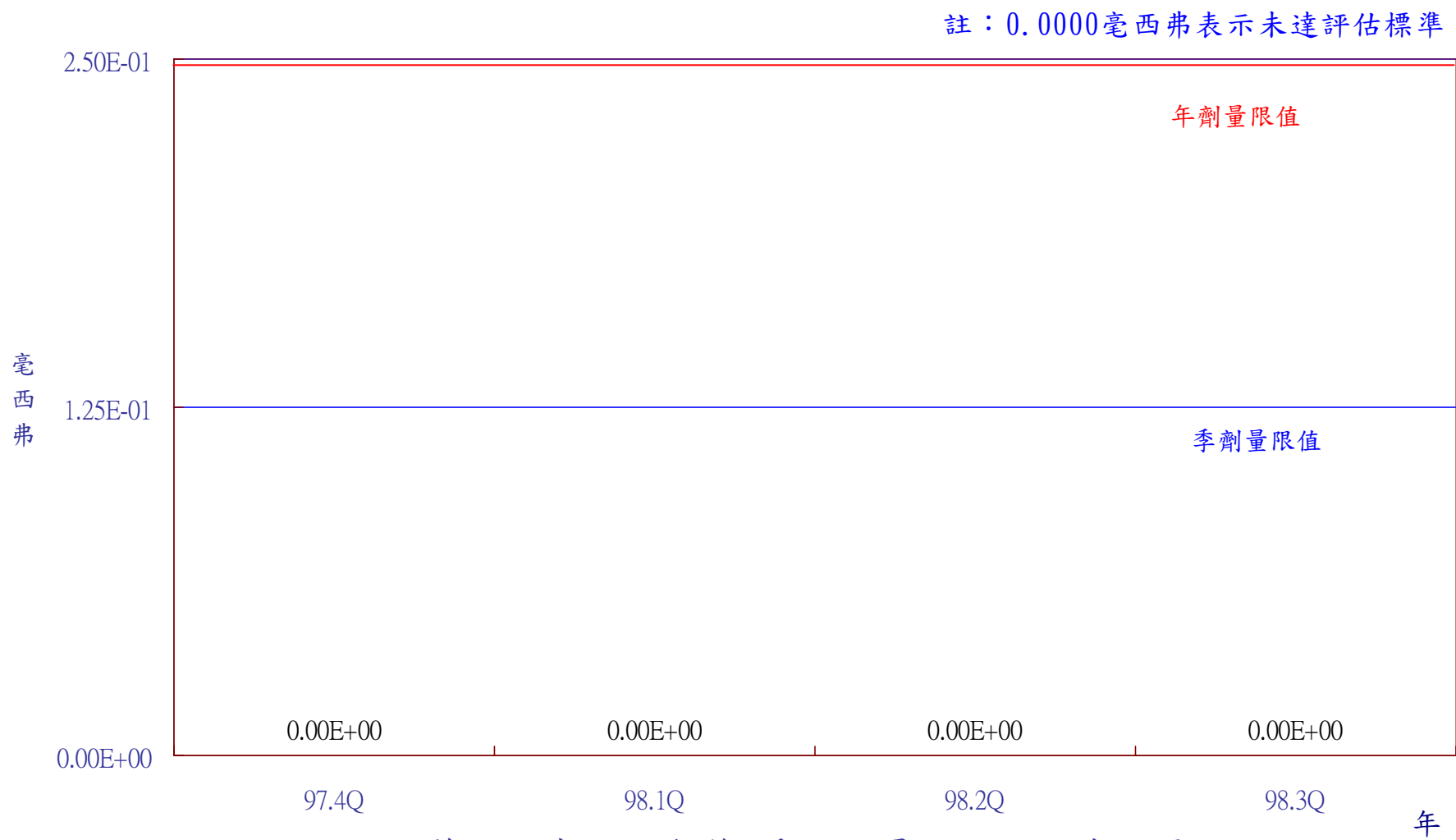
圖5 蘭嶼貯存場98年第3季民眾最大個人全身劑量
