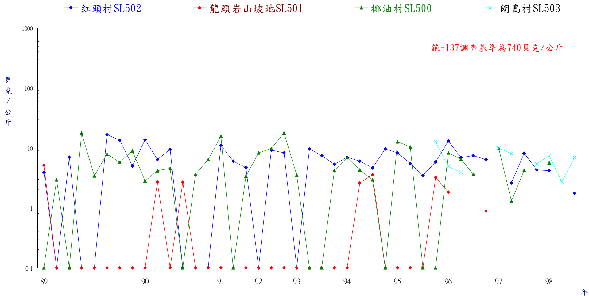
圖3 蘭嶼貯存場土壤銻-137加馬能譜分析結果
