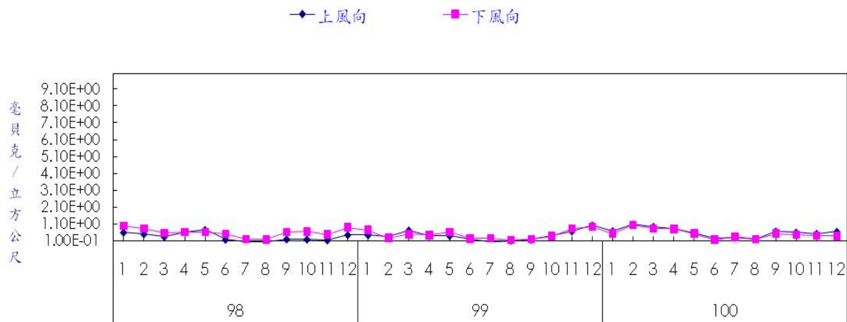
圖 15 核能一廠上下風向空氣微粒總貝他活度監測結果
