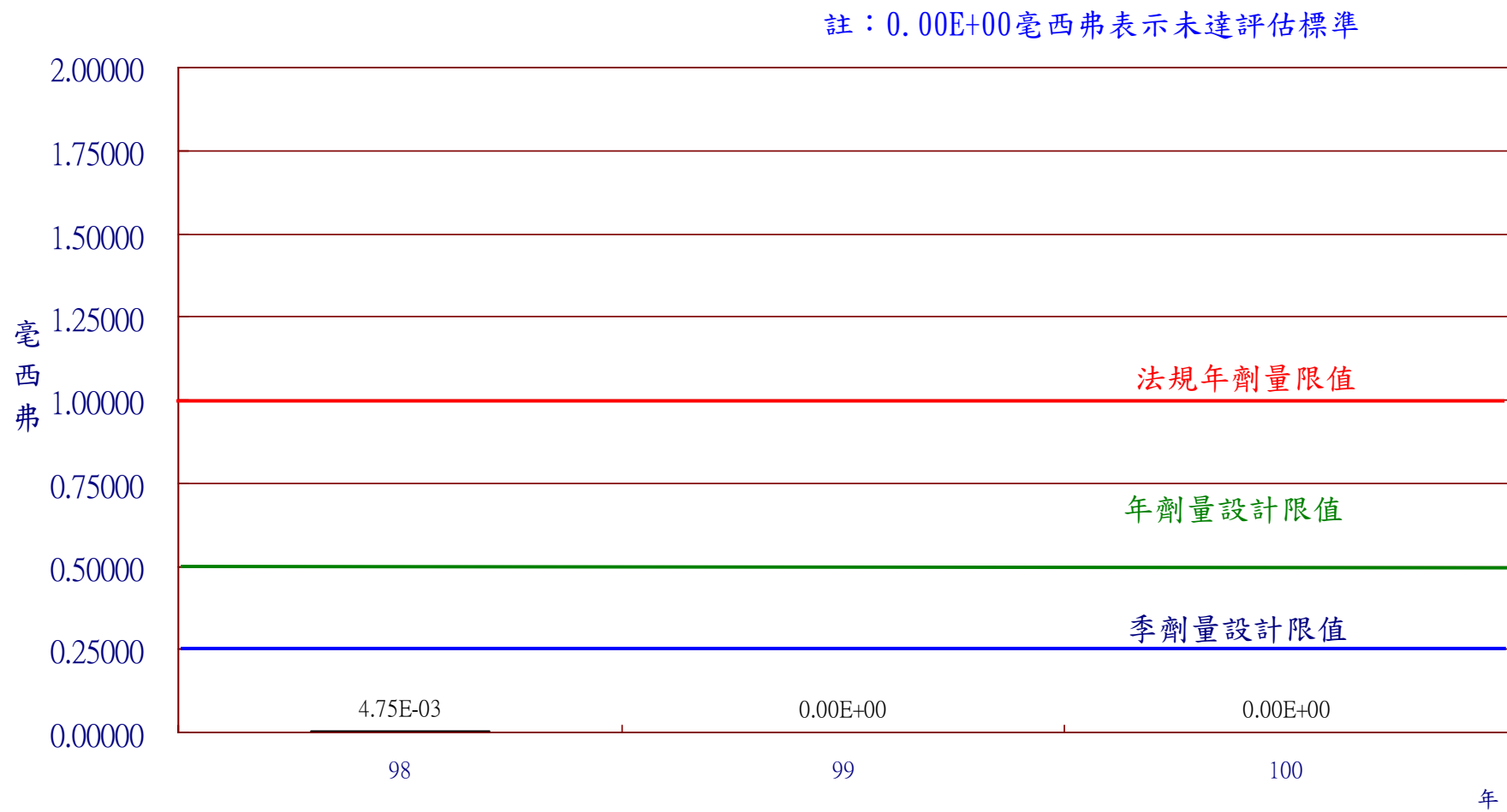
圖18 核能一廠100年民眾最大個人全身劑量
