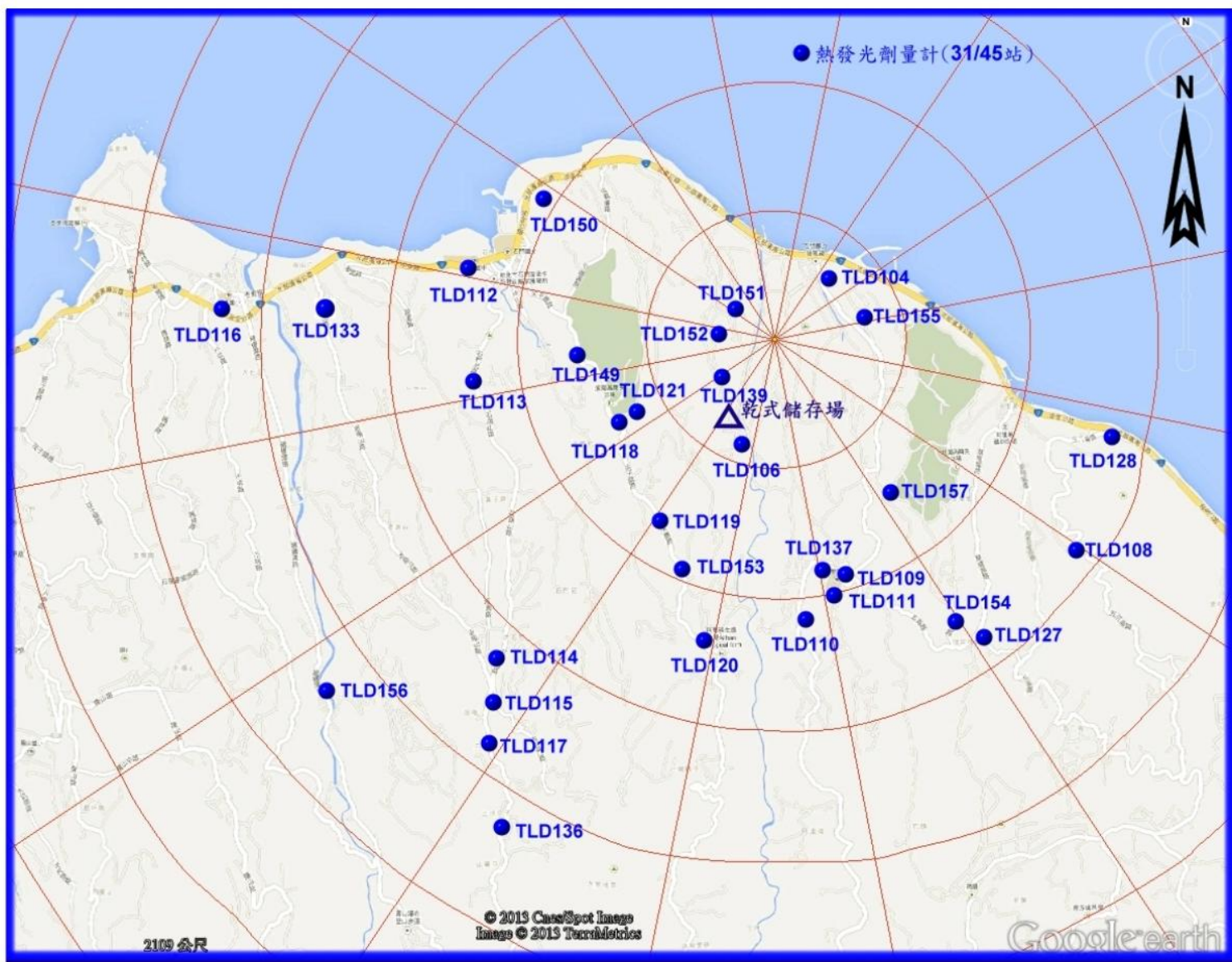
圖 1 核能一廠熱發光劑量計監測站分佈圖(5 公里內)
