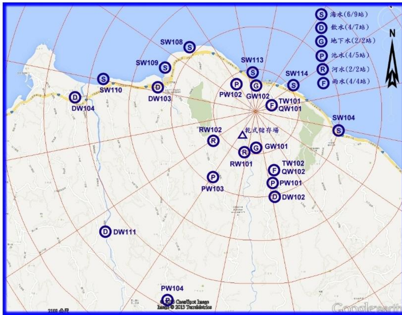
圖 5 核能一廠各類水樣取樣站分佈圖(5 公里內)
