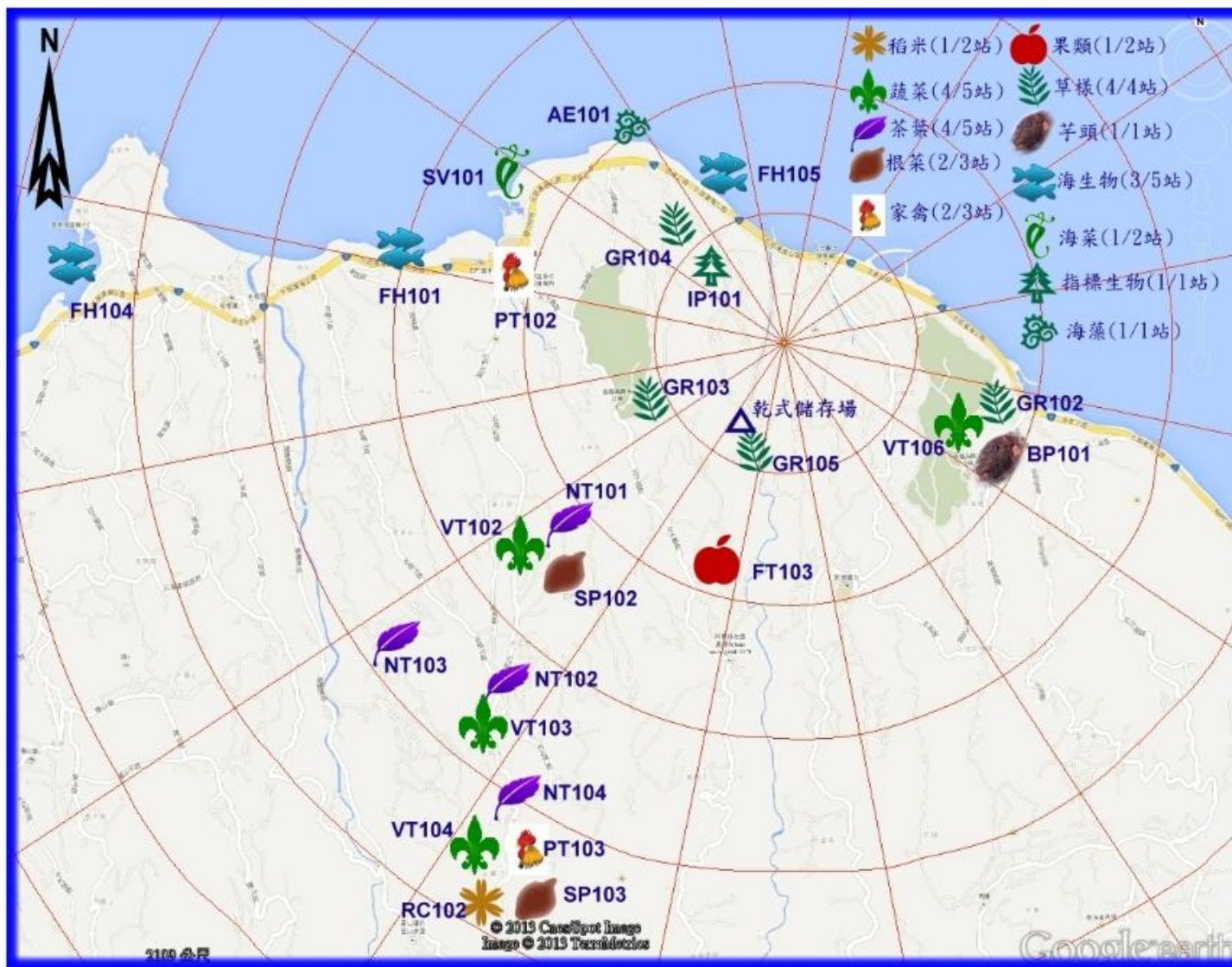
圖 7 核能一廠各類生物樣取樣站分佈圖(5 公里內)
