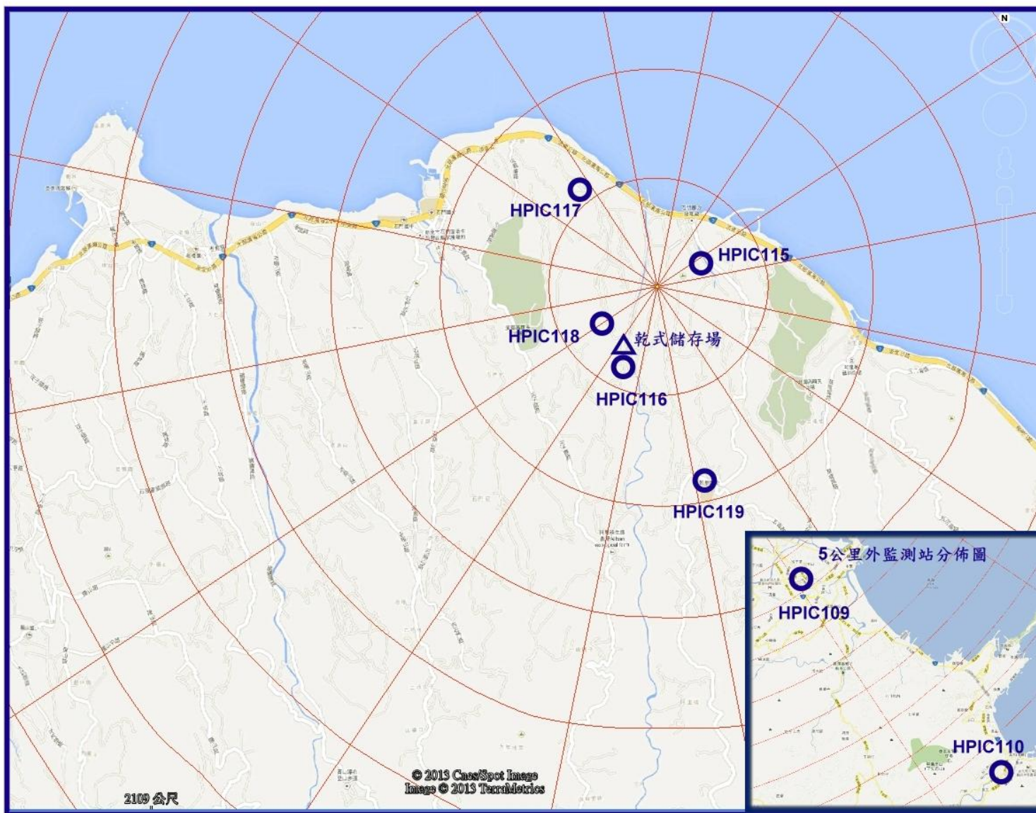
圖 3 核能一廠高壓游離腔監測站分佈圖
