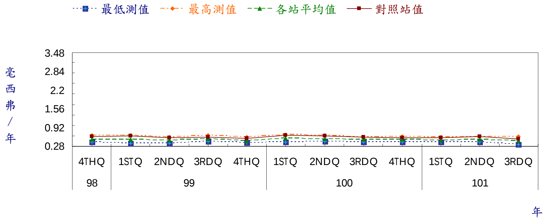
圖14 核能三廠環境熱發光劑量計監測結果
