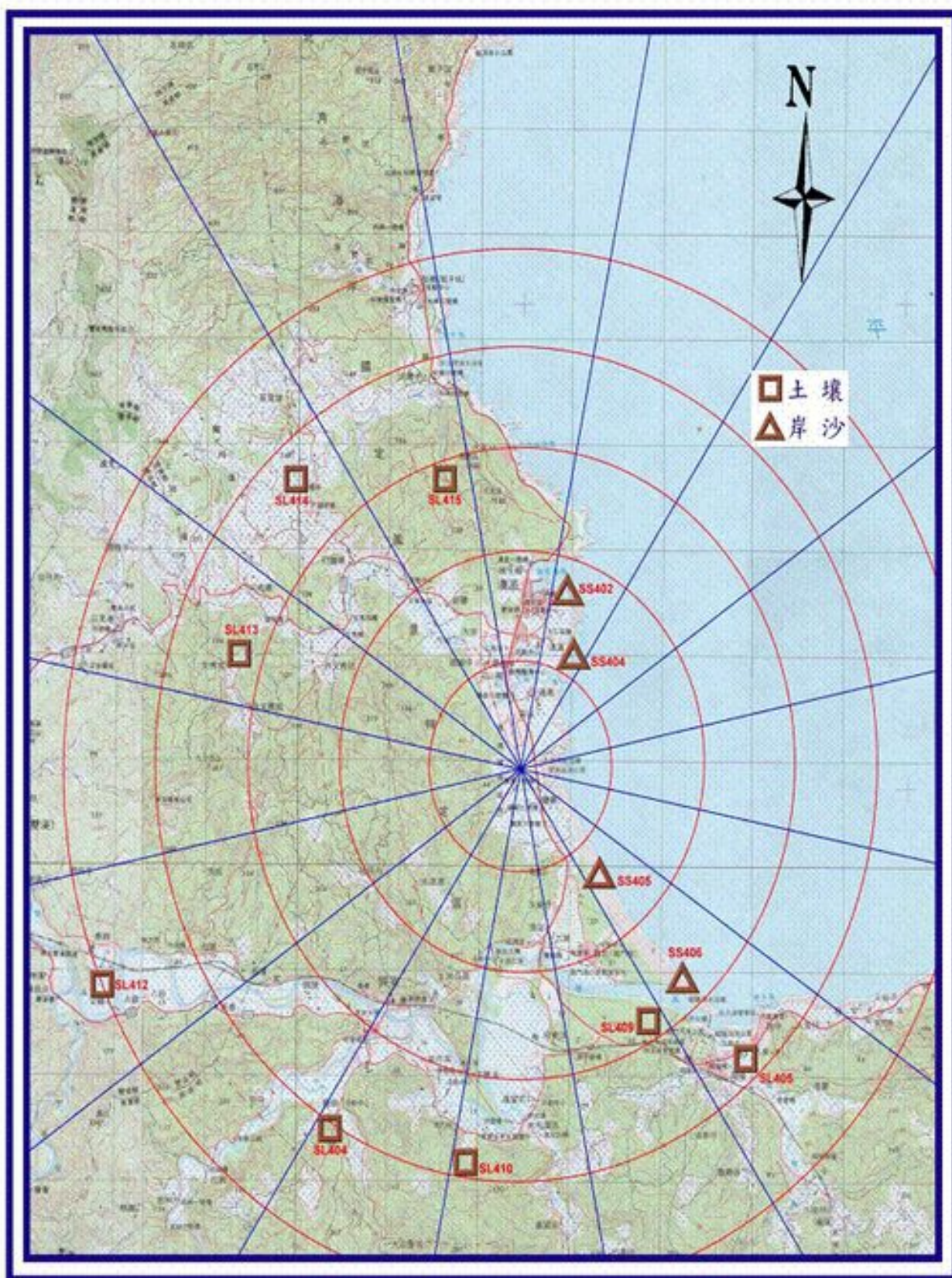
圖10 核能四廠累積試樣取樣站分佈圖(5公里內)
