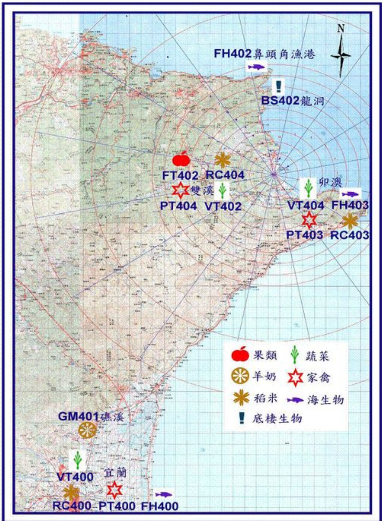
圖9 核能四廠各類生物取樣站分佈圖(5公里外)
