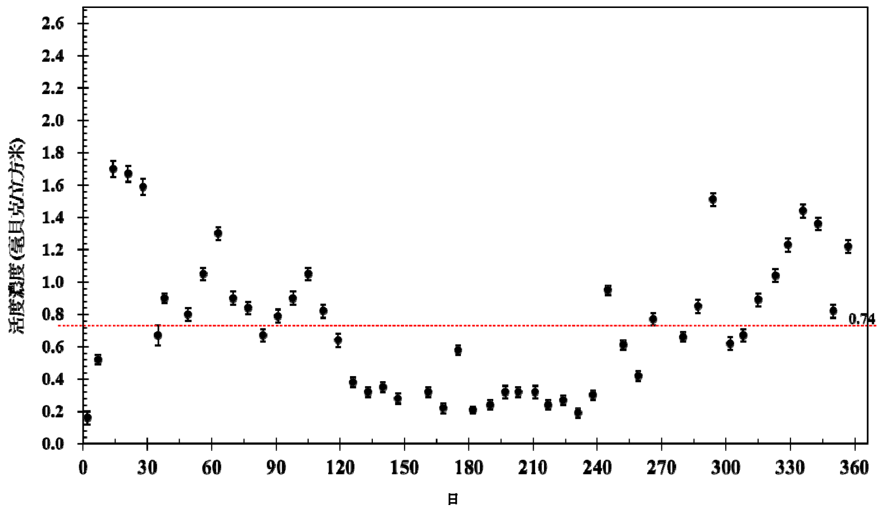
圖7 102年空浮微粒活度濃度變動圖(速器館側)
