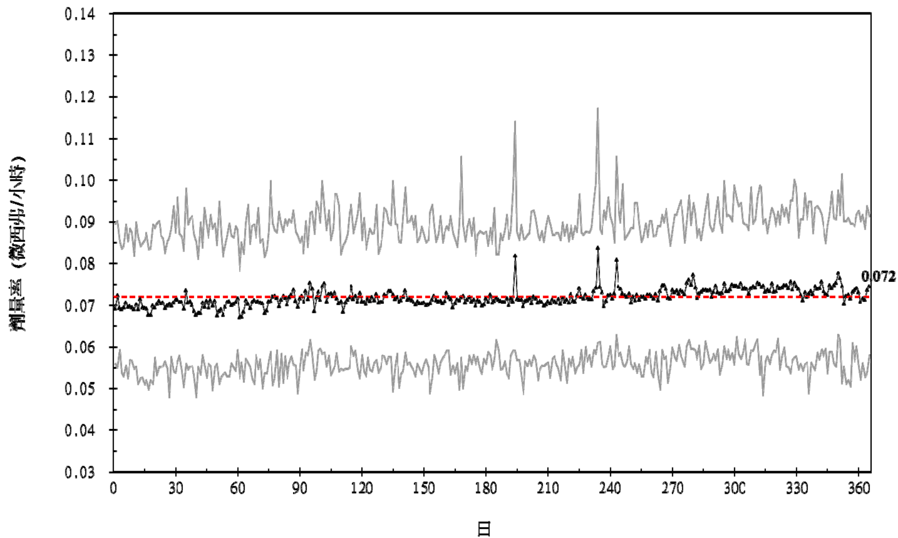
圖5 102年連續輻射偵測劑量率變動圖(加速器館側)
