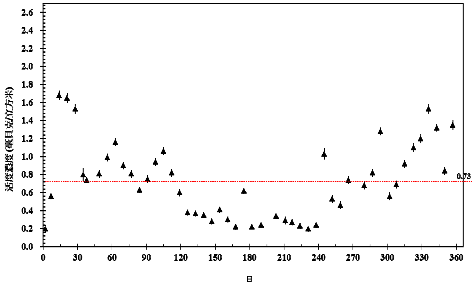
圖6 102年空浮微粒活度濃度變動圖(原科中心)
