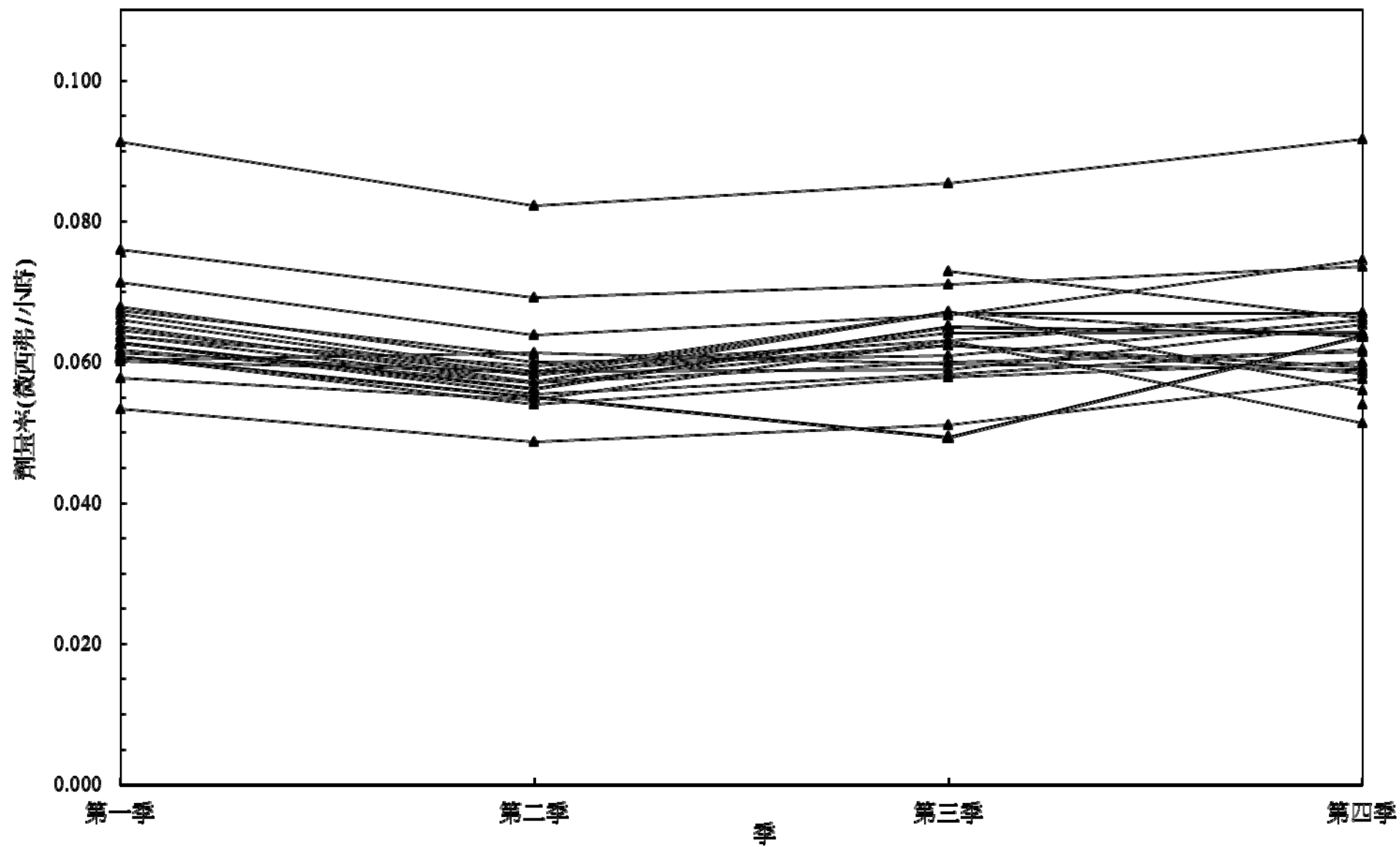
圖2 102年熱發光劑量計偵測站劑量率變動圖
