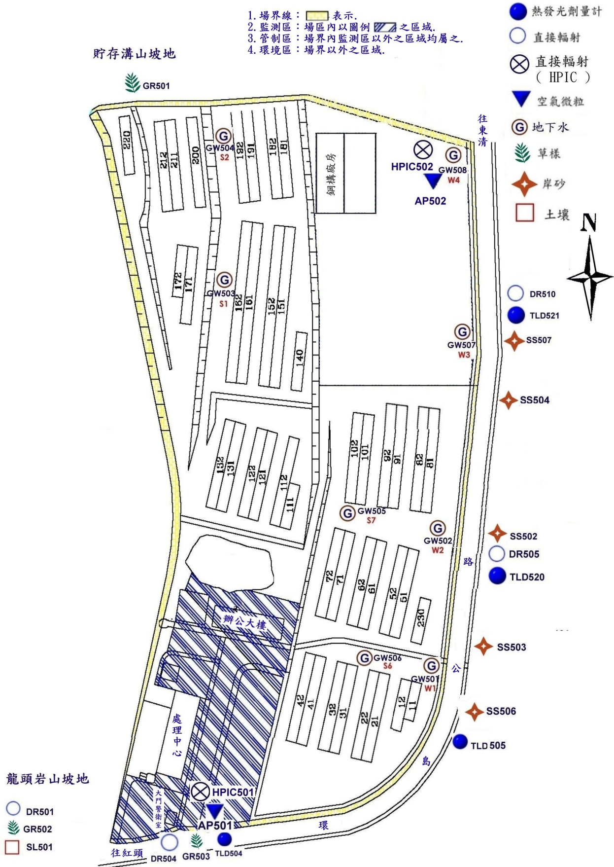
圖2 蘭嶼貯存場周邊各類試樣取樣／監測站分布圖
