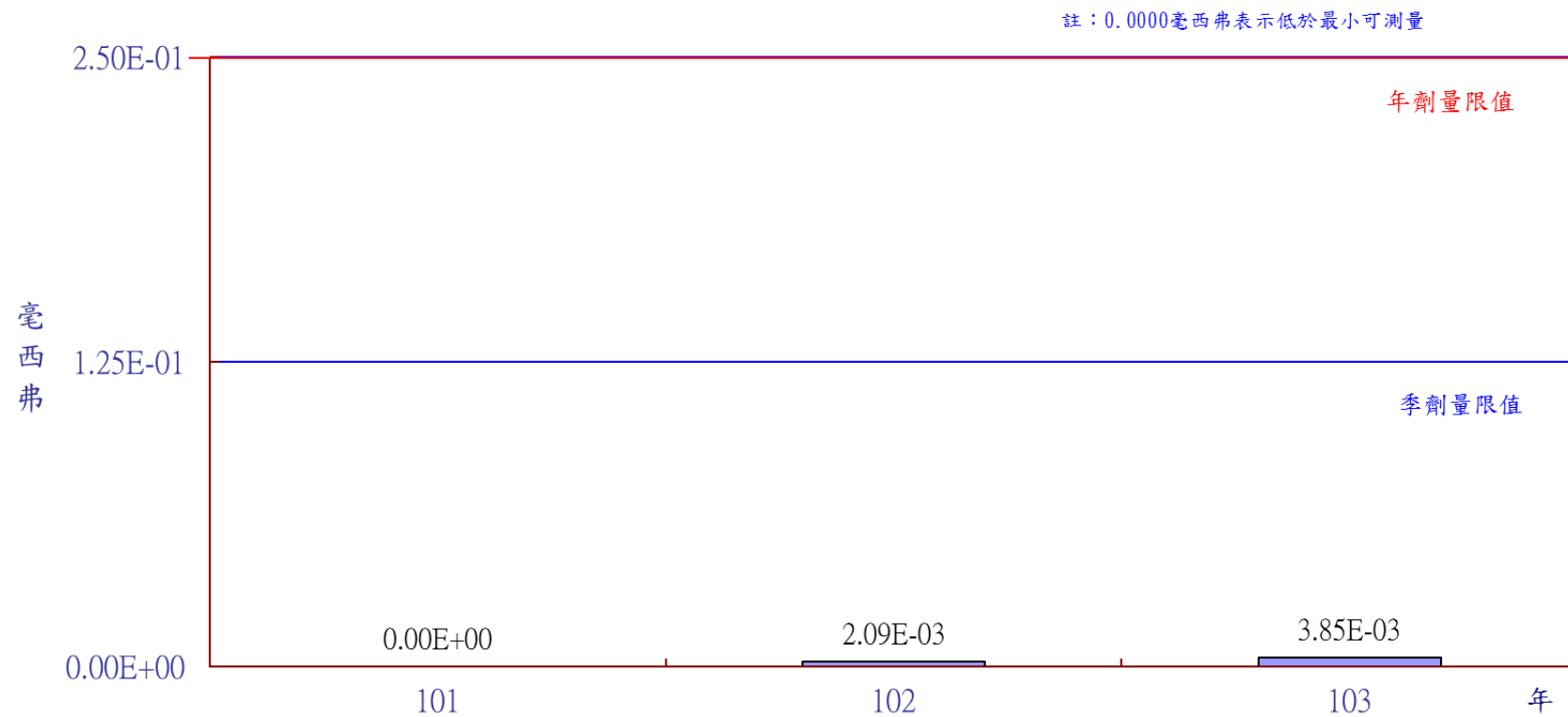
圖5 蘭嶼貯存場103年民眾最大個人全身劑量
